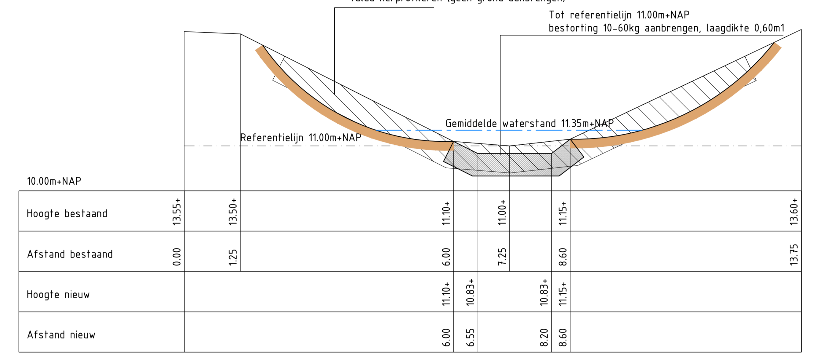
Dwarsprofiel A-A Schaal 1:50
