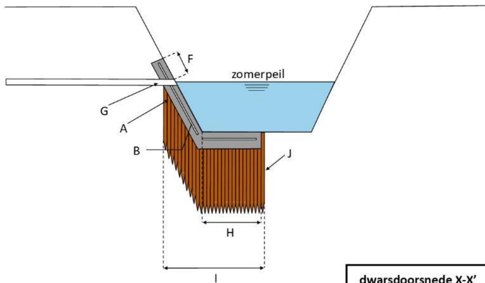
dwarsdoorsnede X-X'
