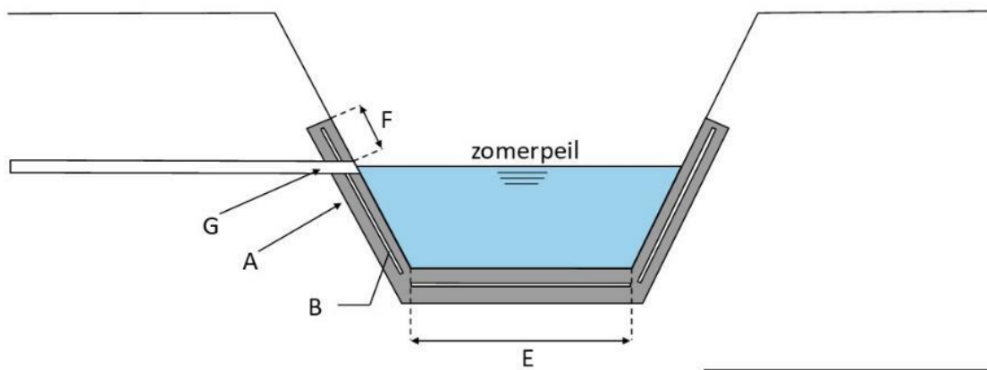
dwarsdoorsnede X-X'
