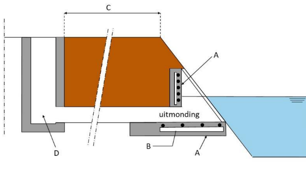
Dwarsdoorsnede X-X'
