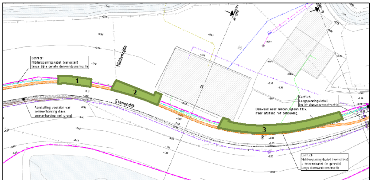
Figuur 4.1: de locaties van de sierheester (1) en ligusterhaag (2 en 3) ten opzichte van het damwandprofiel (oranje lijn)
