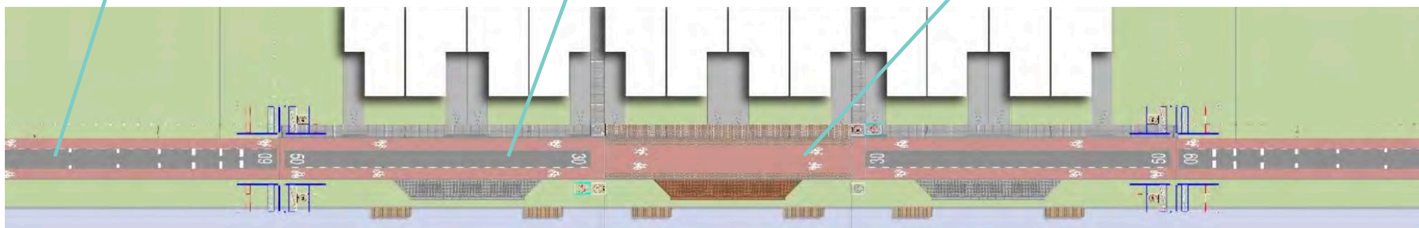
Principeprofiel voor de Ringvaartdijk (gemeente Haarlemmermeer)
