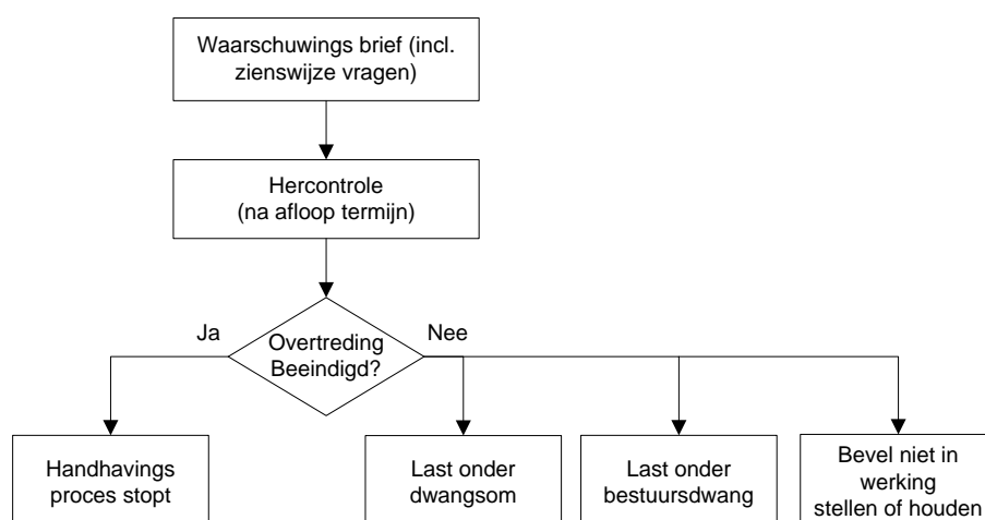
Schema reactie 2
