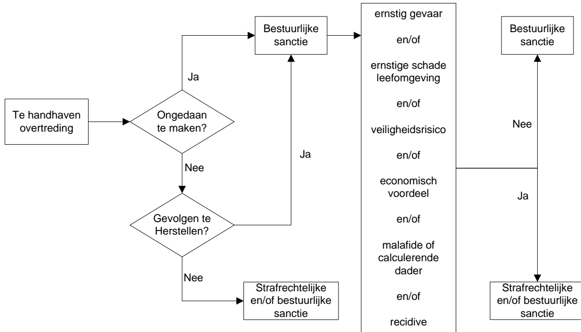
Schema reactie 3
