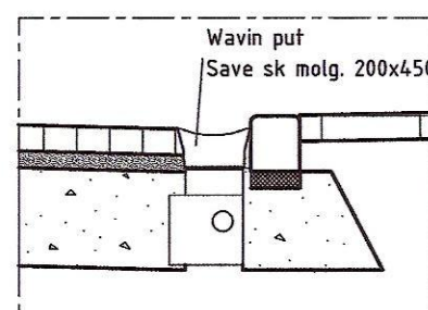
Doorsnede A-A (t.p.v. kolk) Schaal 1:10
