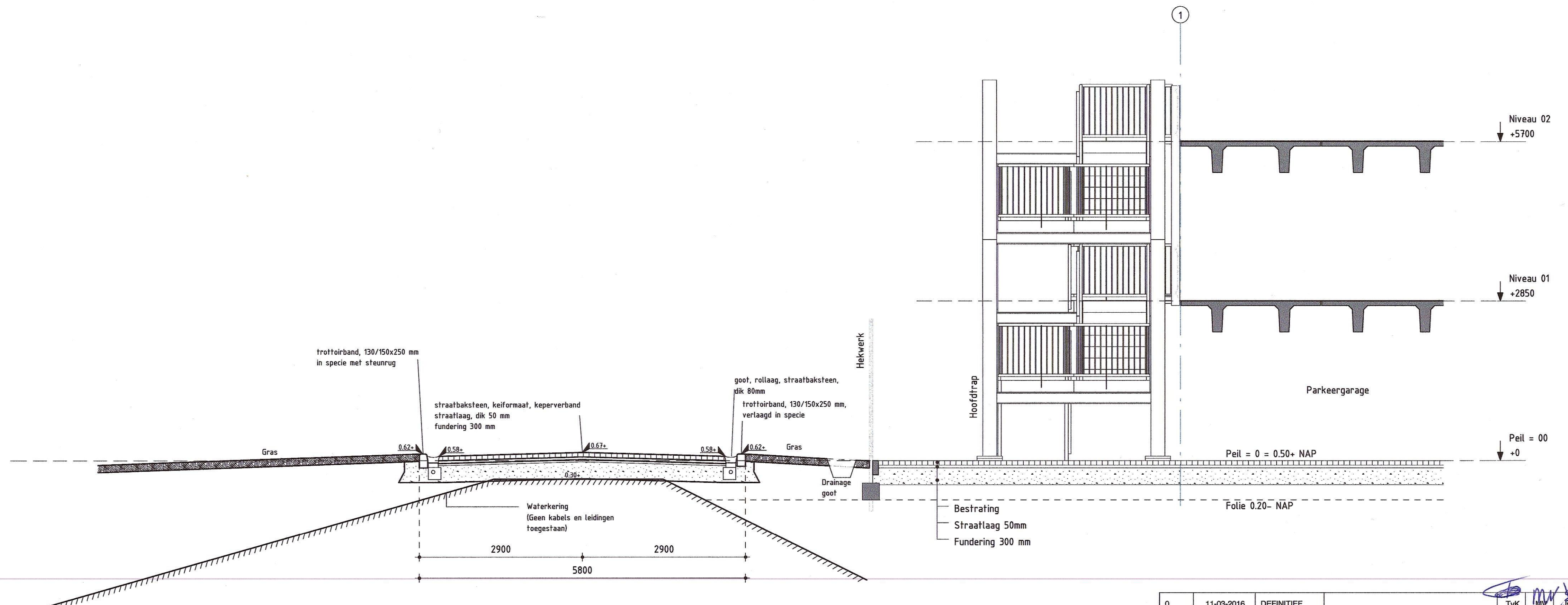
Doorsnede C-C schaal 1:50
