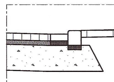
Doorsnede B-B (hoogste punt tussen de kolken) Schaal 1:10
