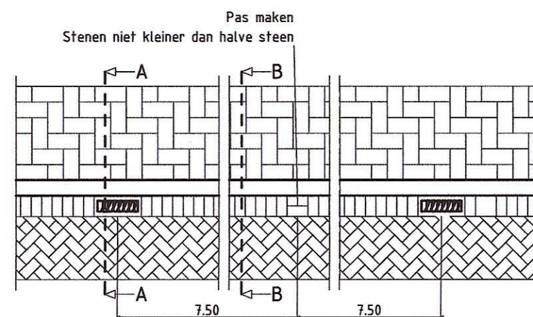
PRINCIPE DETAIL 6: Goot, rollaag straatbaksteen Schaal: 1:20
