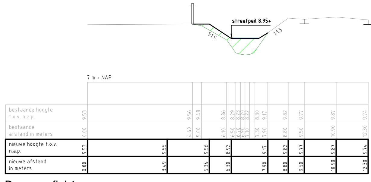
Dwarsprofiel 1
