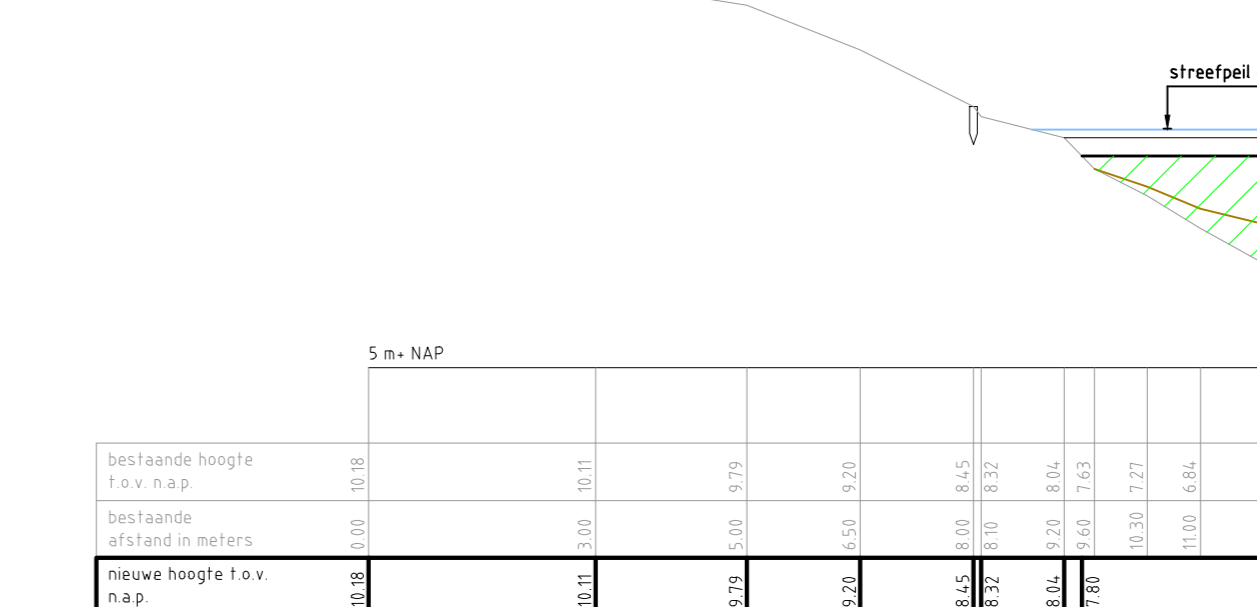
Dwarsprofiel 10
