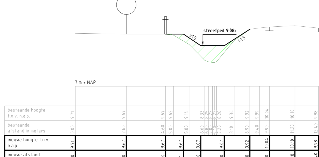
Dwarsprofiel 3
