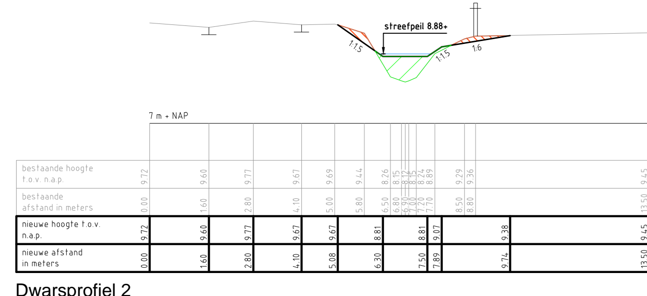
Dwarsprofiel 2
