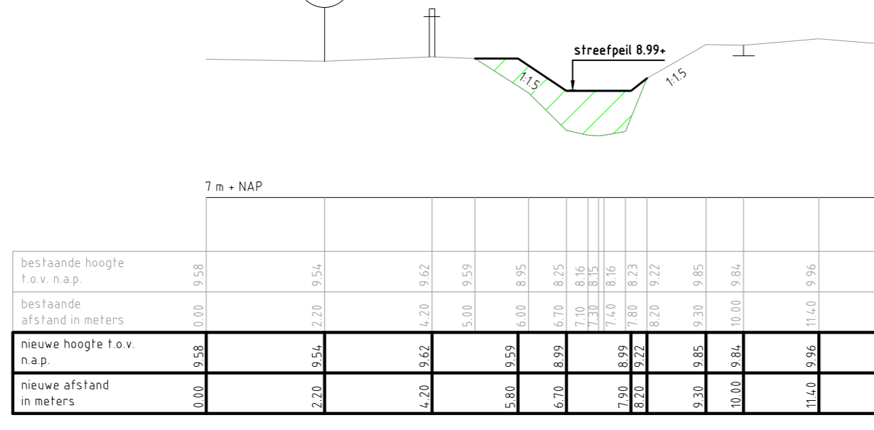
Dwarsprofiel 2
