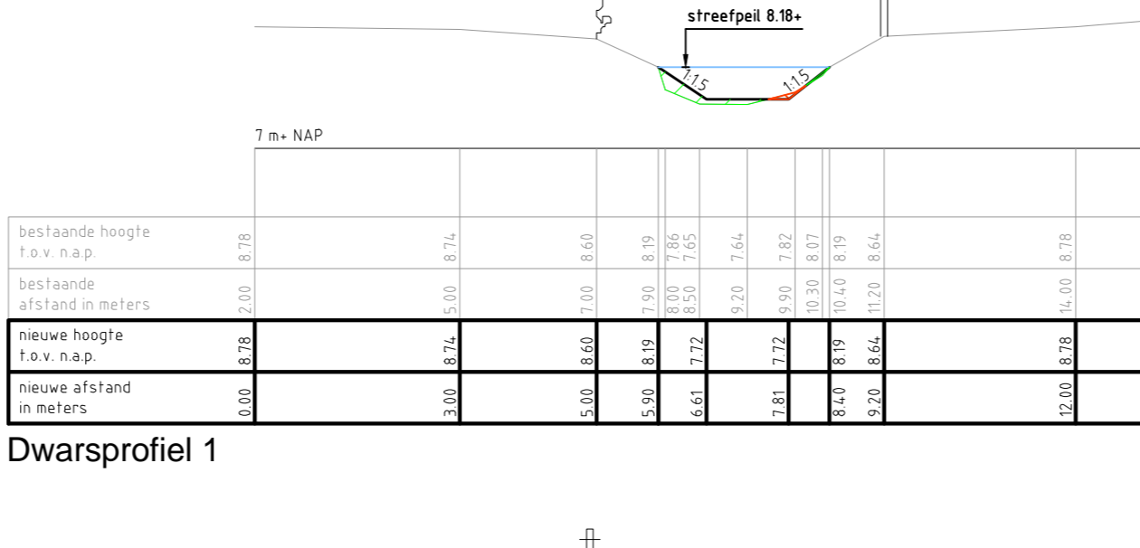
Dwarsprofiel 2
