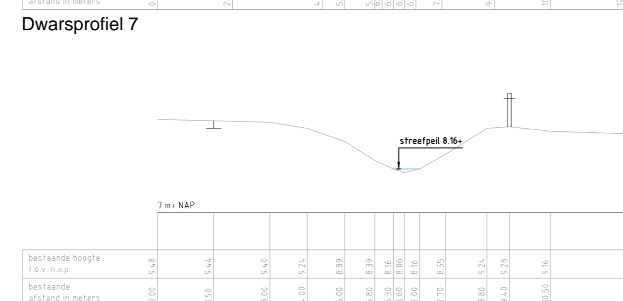
Dwarsprofiel 7
