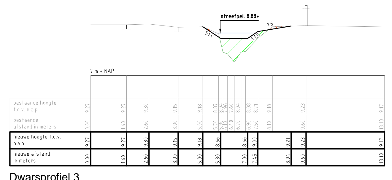
Dwarsprofiel 3
