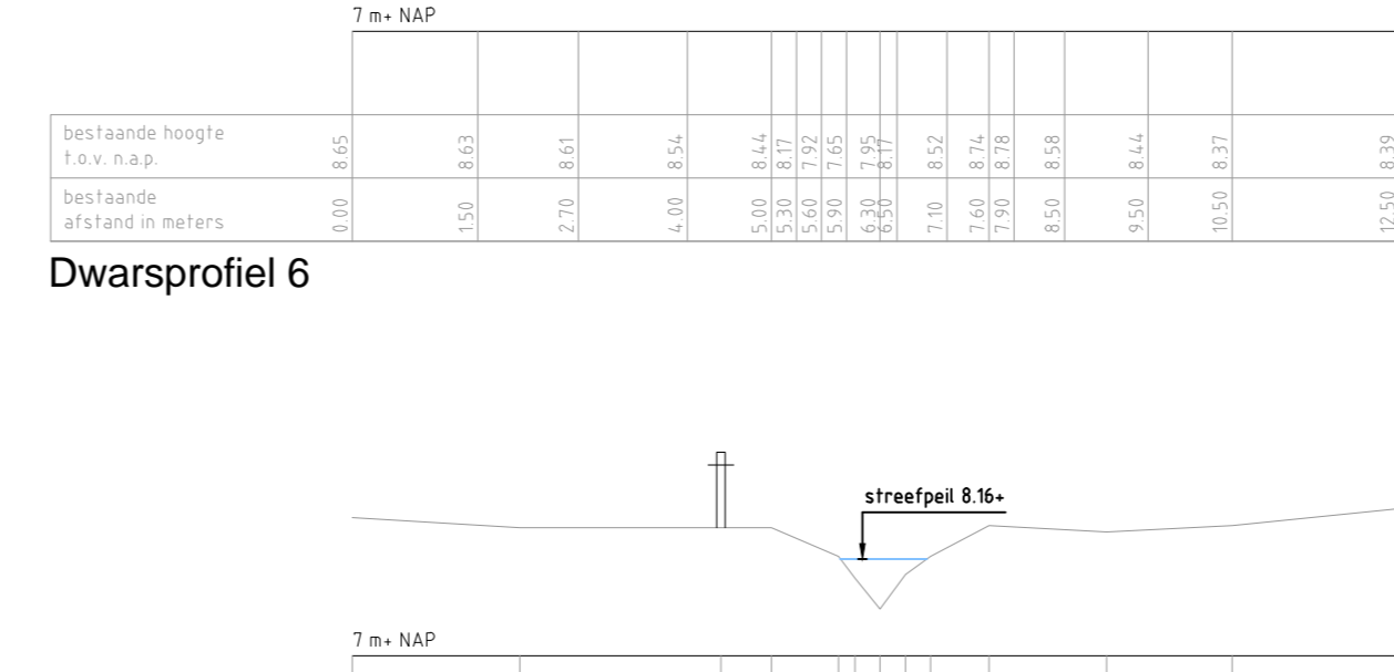
Dwarsprofiel 6
