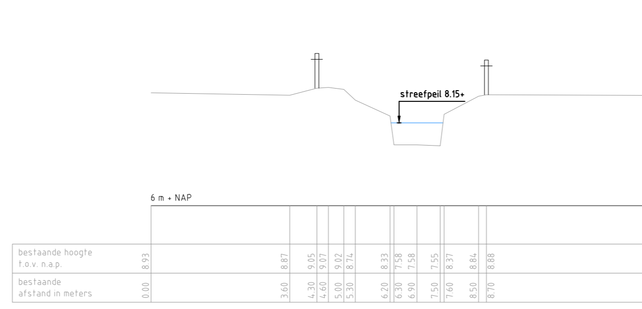
Dwarsprofiel 3
