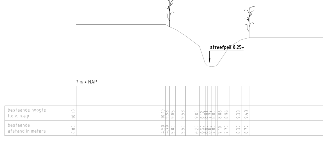
Dwarsprofiel 4
