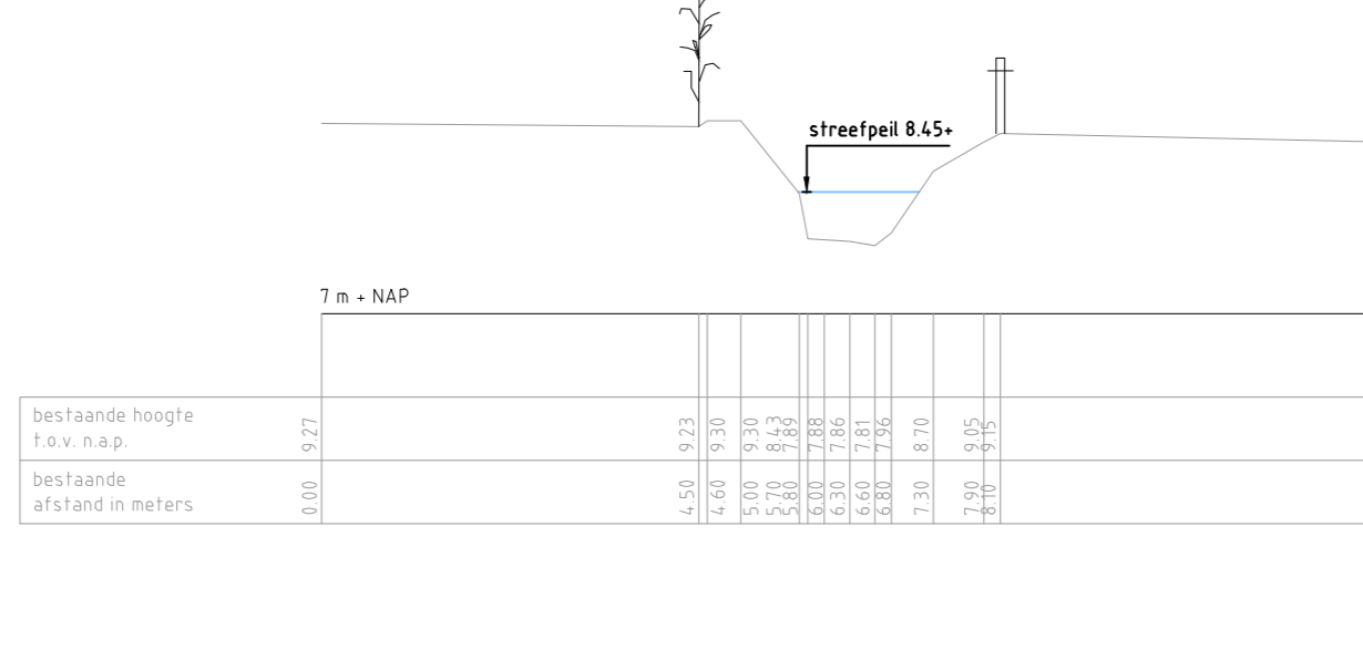
Dwarsprofiel 6
