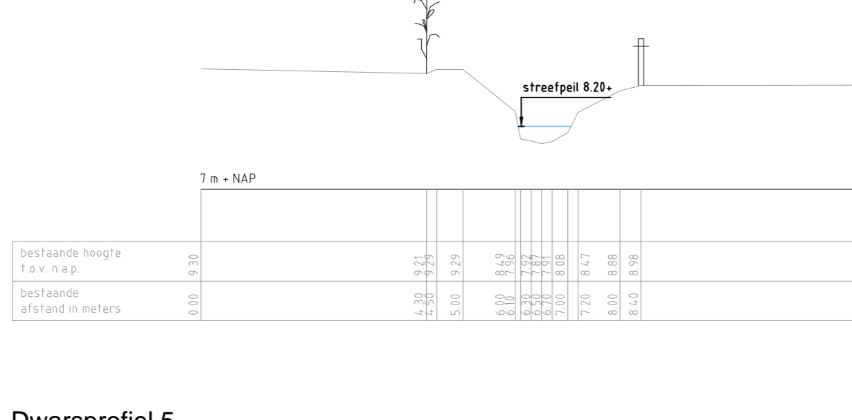
Dwarsprofiel 5
