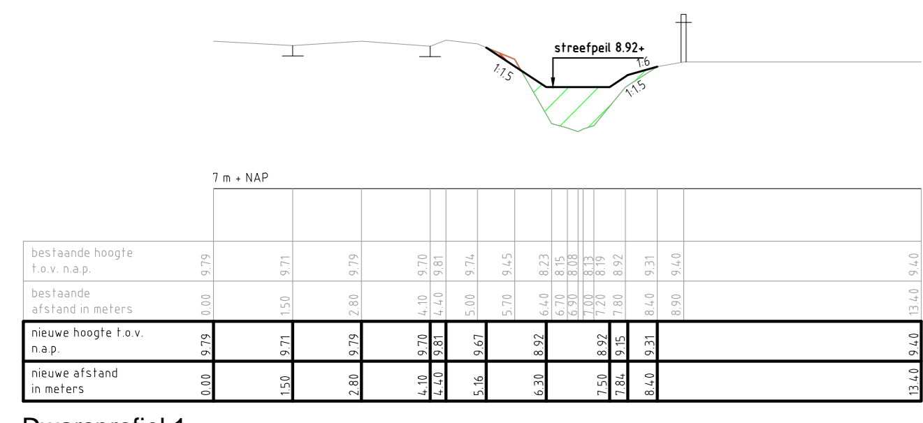
Dwarsprofiel 1
