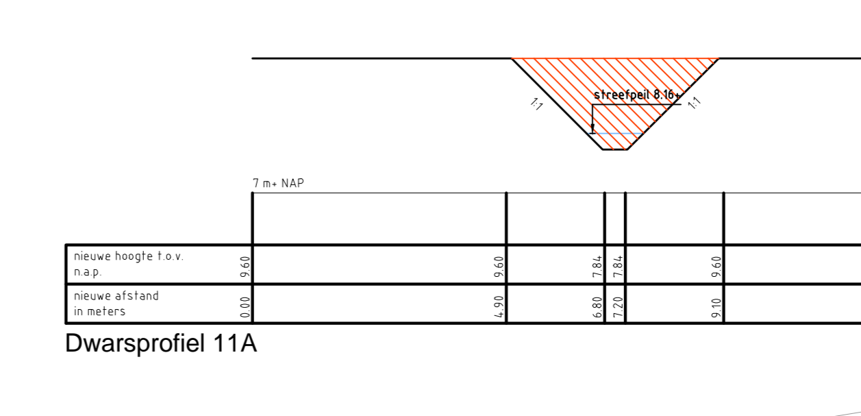
Dwarsprofiel 11
