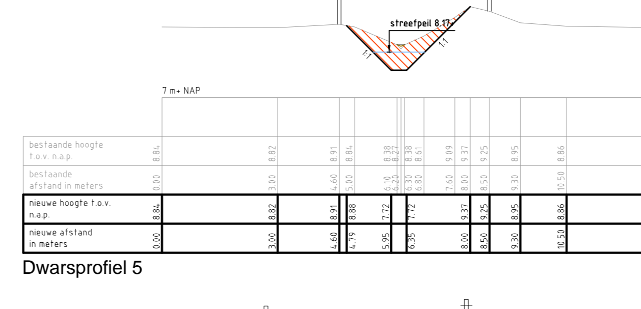
Dwarsprofiel 5
