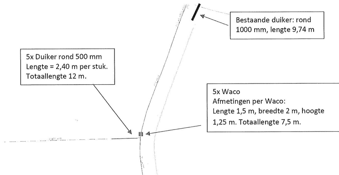
Figuur 1 Situatieschets van de te plaatsen duikers in de ES108 en ES3.
