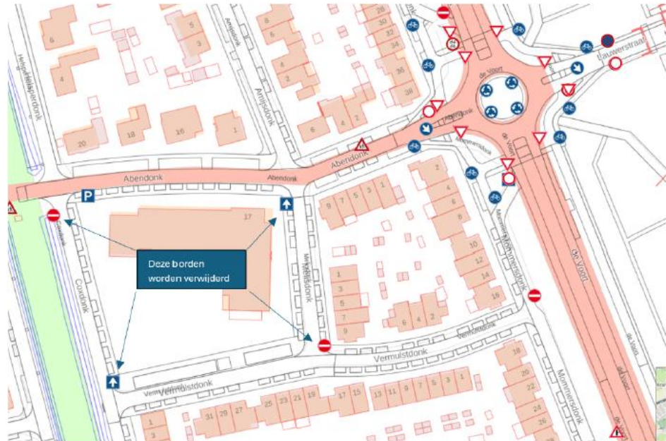
Figuur 1 Oude situatie eenrichtingsverkeer Melisdonk, Vermulstondk, Coxdonk.
