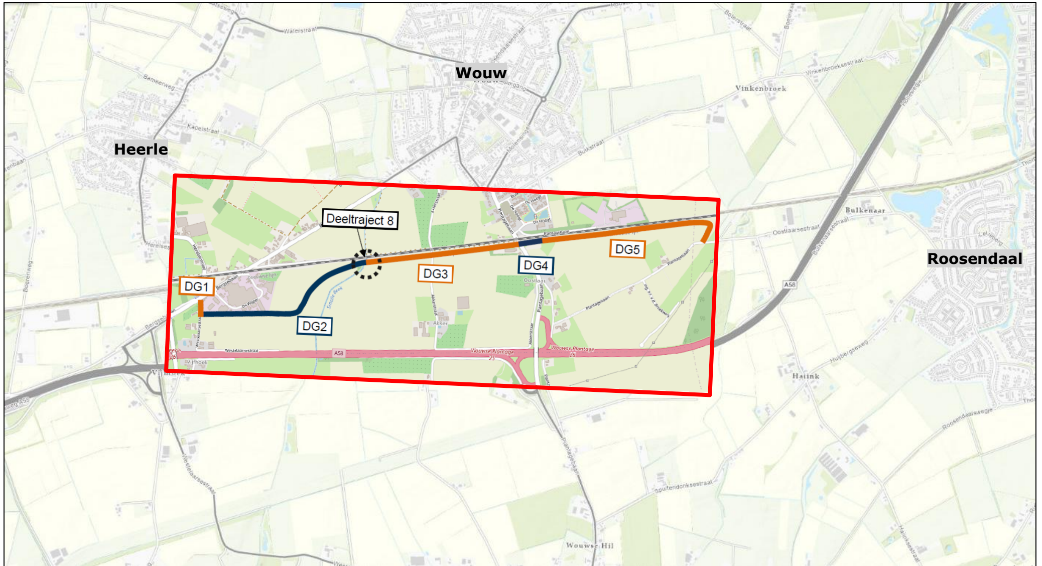
988846-A Topografische situatie
