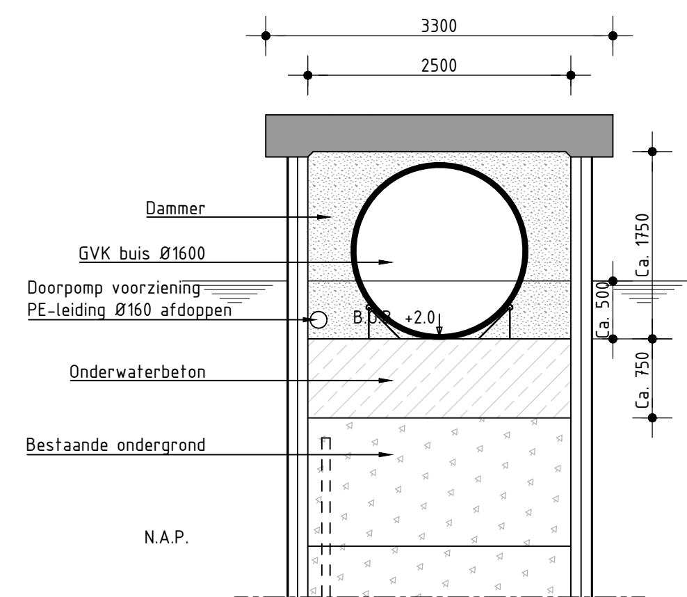
Doorsnede B-B Schaal 1:50
