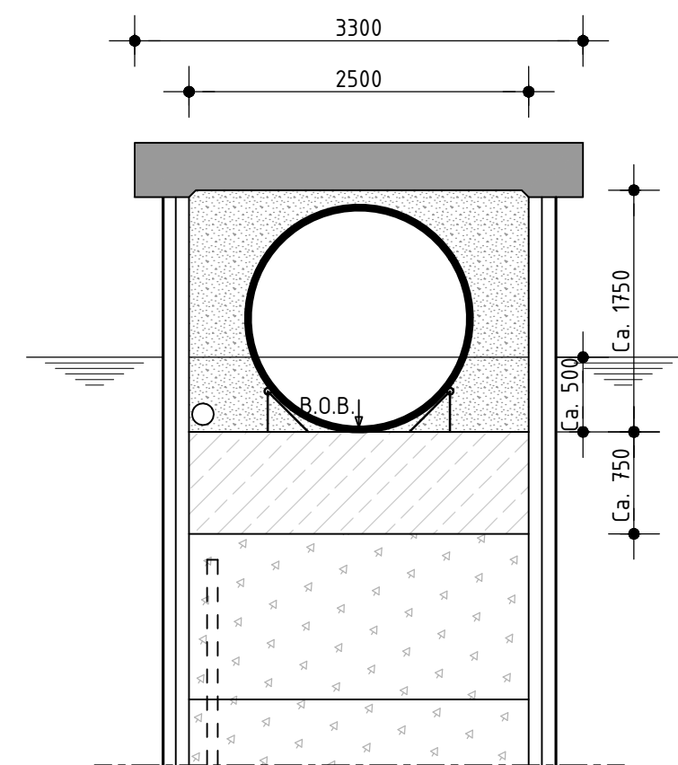
Doorsnede B-B Schaal 1:150
