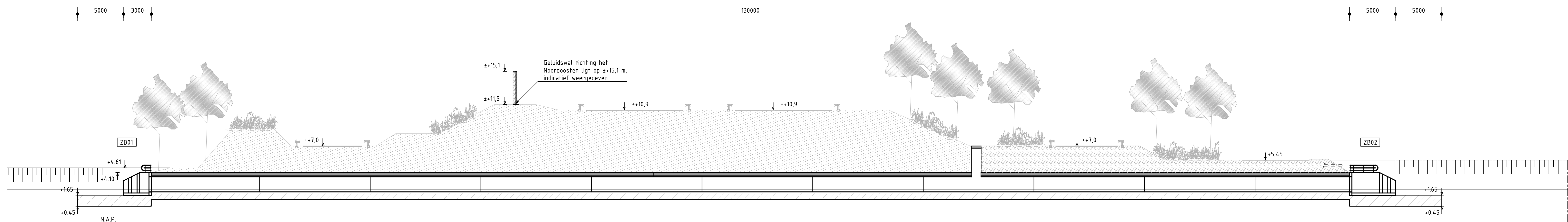
Doorsnede A-A Schaal 1:200
