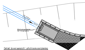
Detail bovenaanzicht uitstroombestemming Situat. 151
