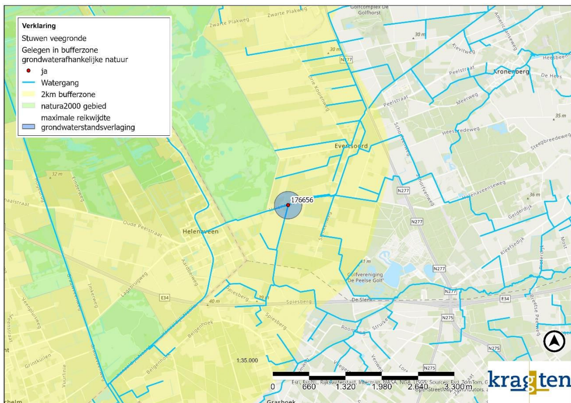
Afbeelding 9 Reikwijdte bemaling stuw 176656 Mariagepeel
