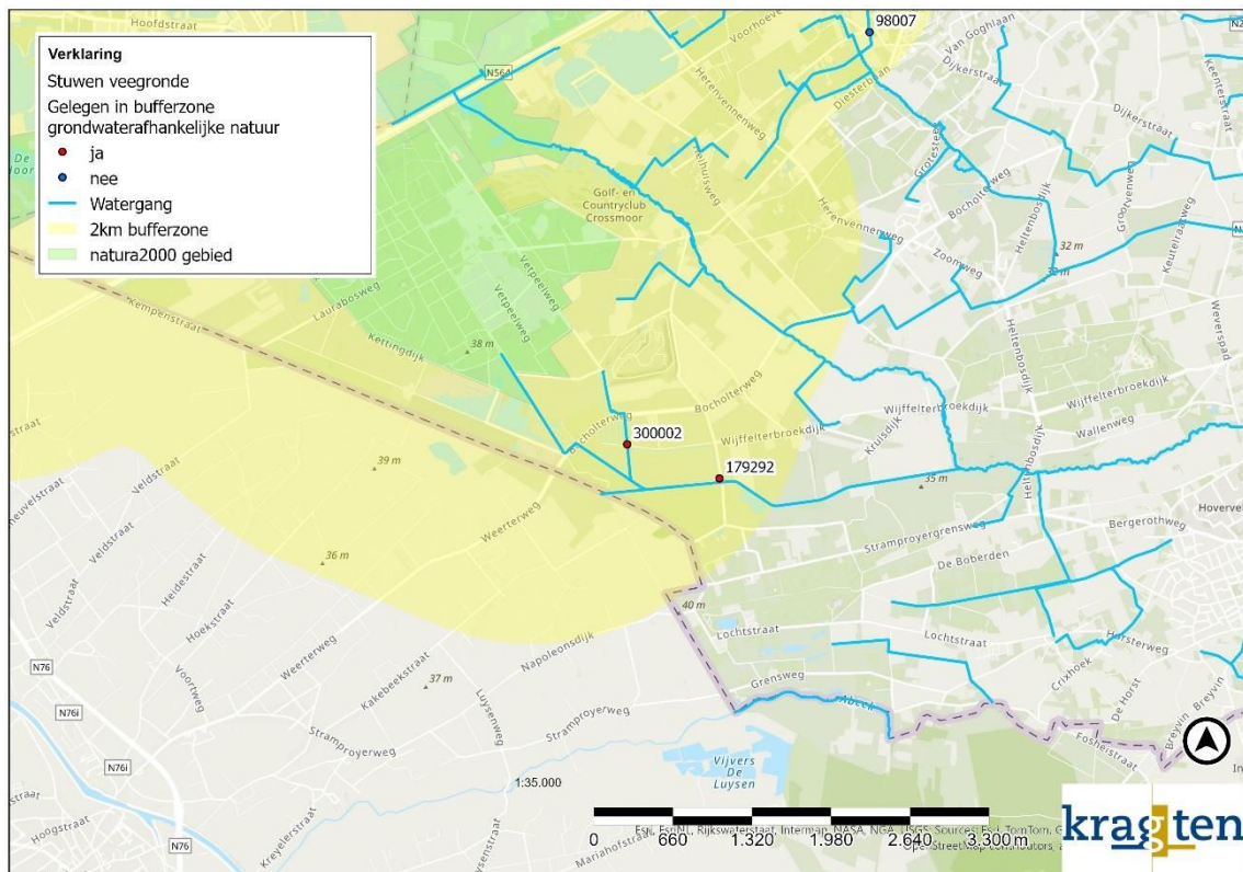
Afbeelding 4 Stuwen 300002 en 179292 nabij Natura 2000-gebied Weerter- en Budeler Bergen
