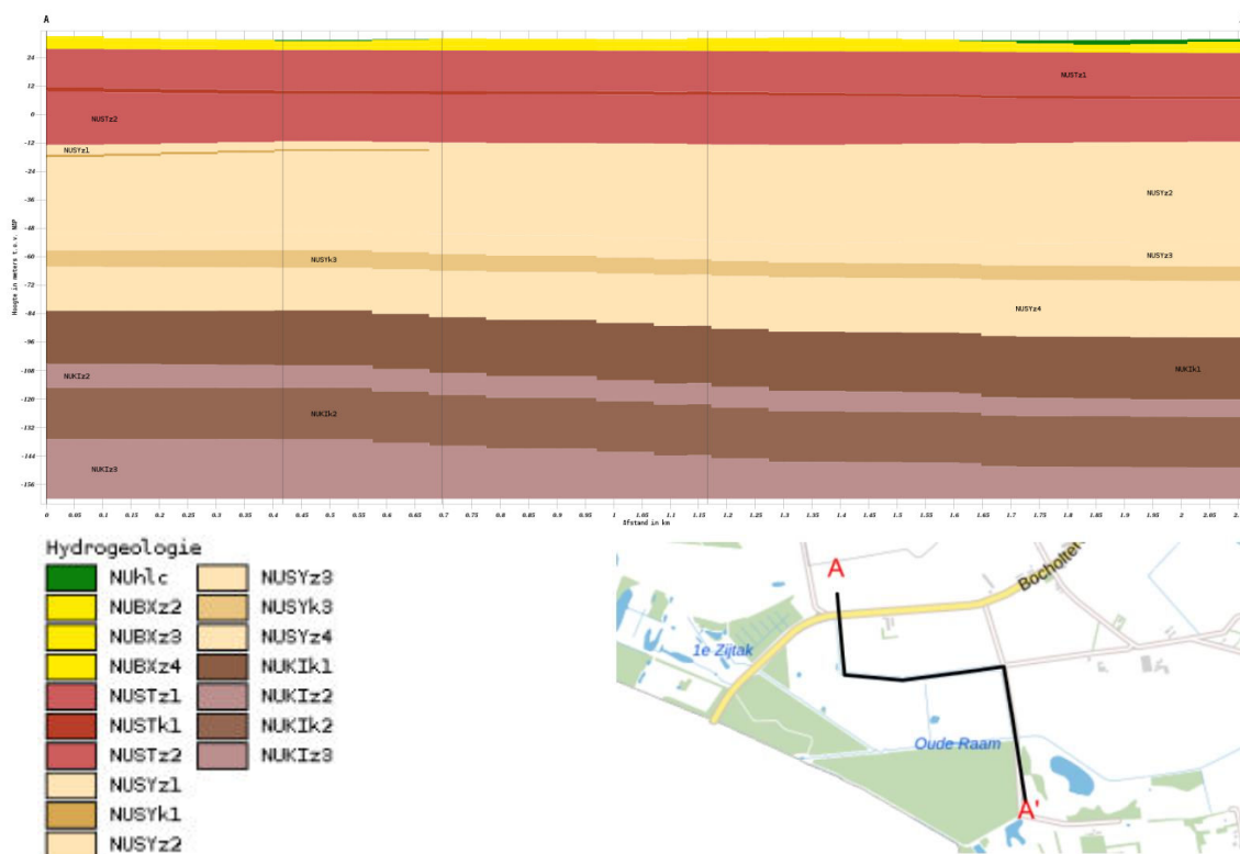
Afbeelding 7 Bodemopbouw volgens REGIS II v2.2 met tussen de buitenste grijze lijnen het plangebied
