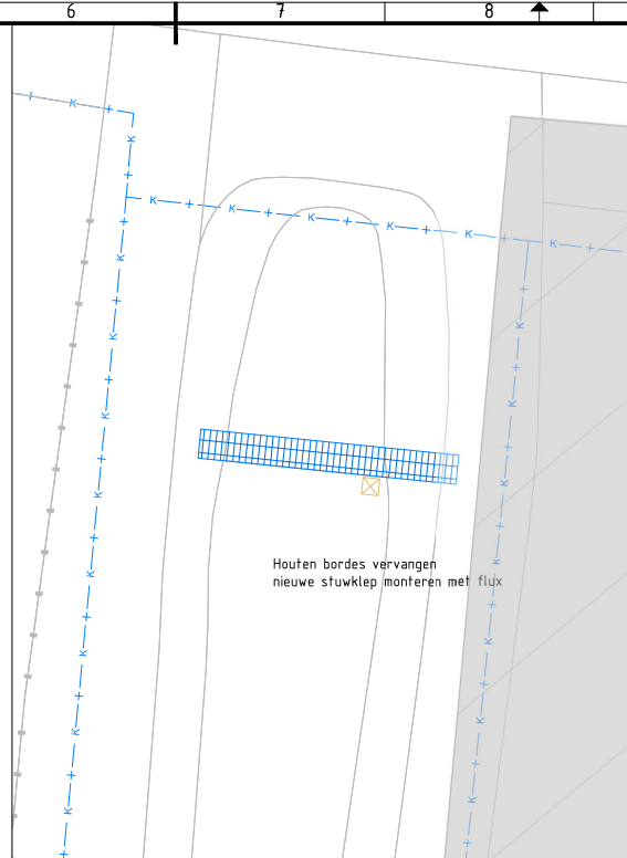
BOVENAANZICHT 1:100
