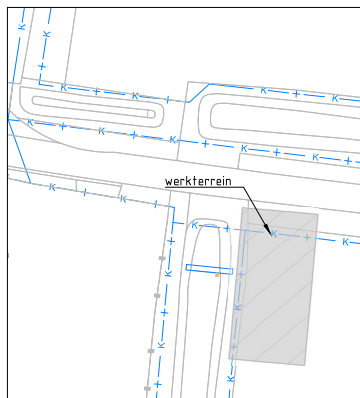
SITUATIE WERKTERREIN 1:500
