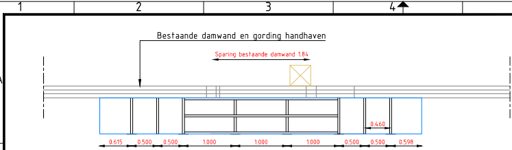
Montage Beugels 150
