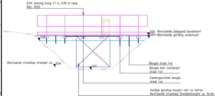
Montage Beugels 150
