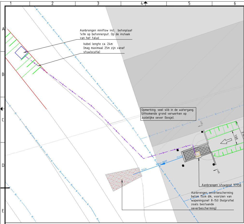
BOVENAANZICHT 1:100
