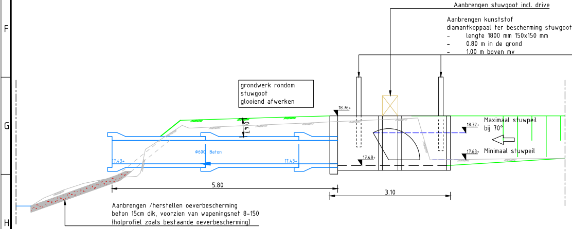
LENGTEPROFIEL 1:50
