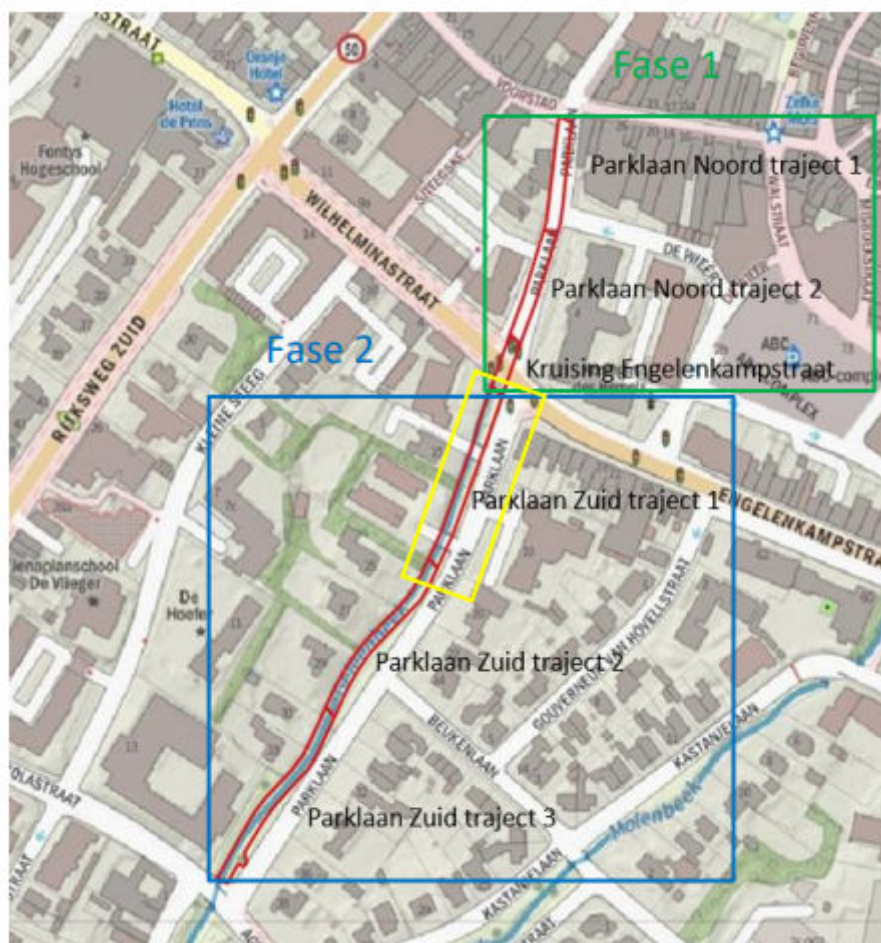
Projectlocatie opgedeeld in trajecten en fases, met afbakening huidige projectfase (geel omkaderd)
