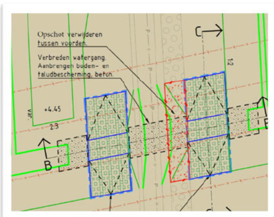
Ontwerp besteksontwerp
