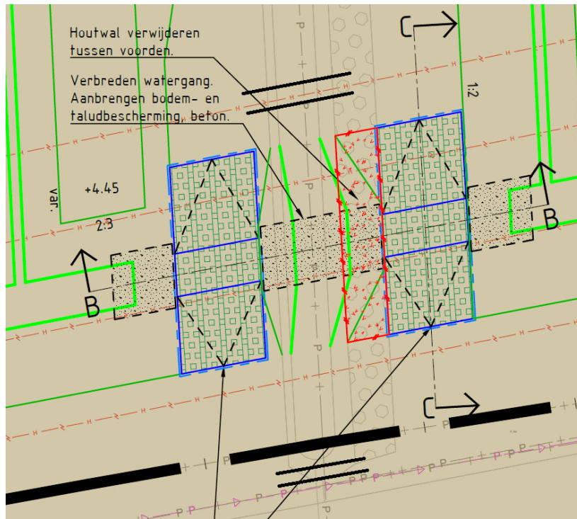
Figuur 2. Locatie waar de afdamming (dubbele zwarte lijnen) gemaakt wordt.
