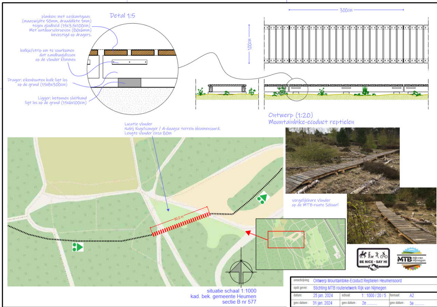
Figuur 5 Bouwtekening van de houten reptienvlinder. De dragers liggen op de liggers (i.p.v. los op de grond) zoals rechtsboven weergegeven, zodat reptielen eronderdoor kunnen.
