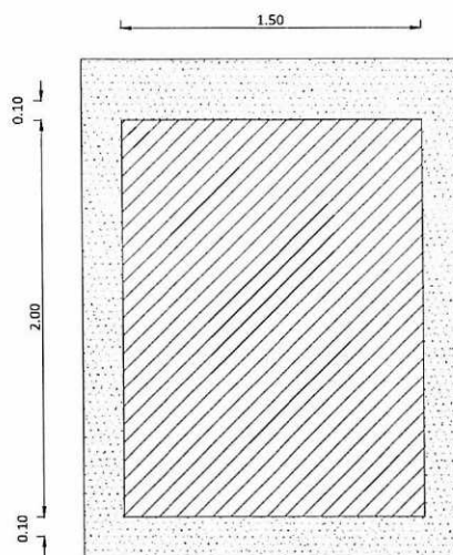
Steenmodel M5-3 Vooraanzicht Schaal 1:20
