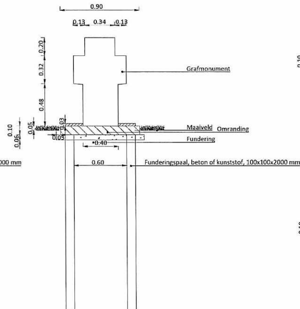
Steenmodel M4-2 Vooraanzicht Schaal 1:20
