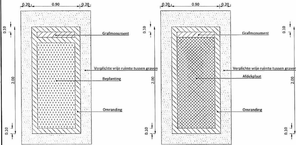
Steenmodel M6-2 Bovenaanzicht Te gebruiken materiaal: natuursteen Schaal 1:20
