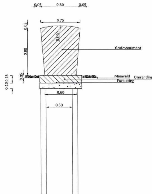
Steenmodel M6-2 Vooraanzicht Schaal 1:20
