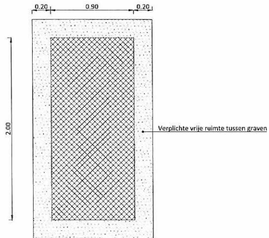
Steenmodel M1 Bovenaanzicht Te gebruiken materiaal: natuursteen Schaal 1:20
