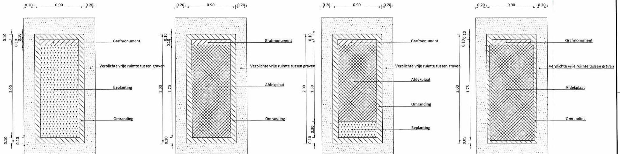
Steenmodel M4-2 Bovenaanzicht Te gebruiken materiaal: natuursteen Schaal 1:20
