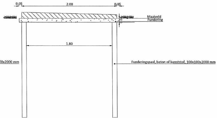
Steenmodel M1 Zijaanzicht Schaal 1:20
