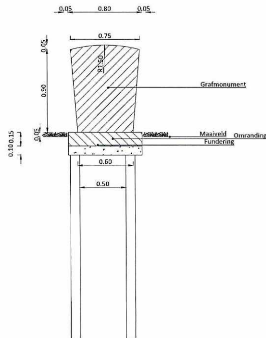
Steenmodel M4-2 Vooraanzicht Schaal 1:20
