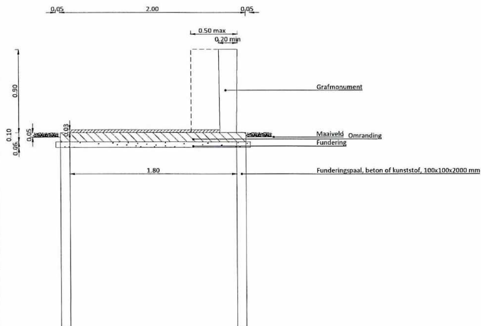
Steenmodel M5-3 Zijaanzicht Schaal 1:20
