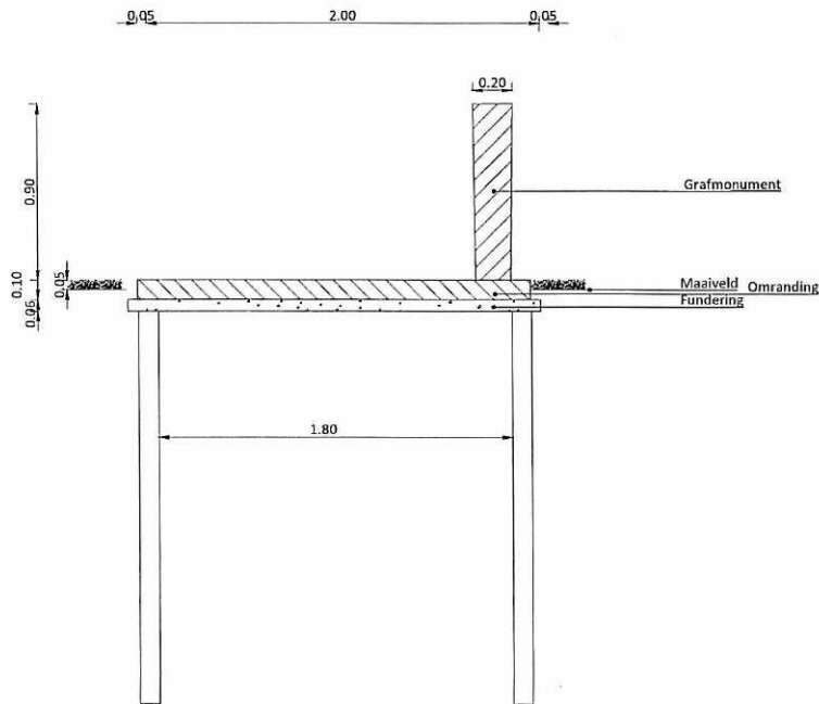
Steenmodel M6-2 Zijaanzicht Schaal 1:20
