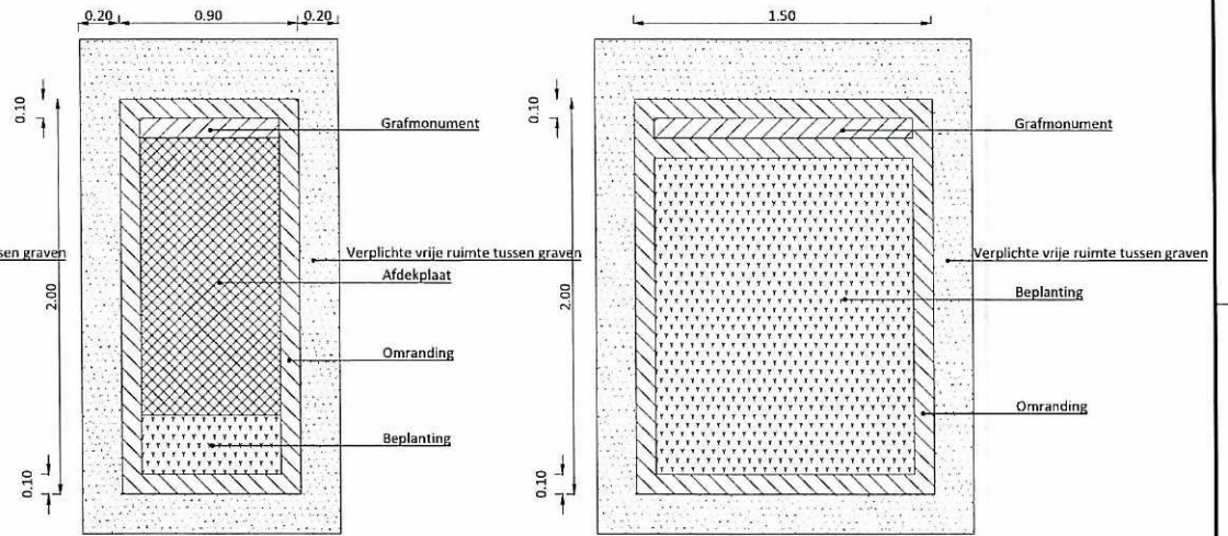
Steenmodel M6-2 Bovenaanzicht dubbel Te gebruiken materiaal: natuursteen Schaal 1:20
