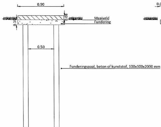
Steenmodel M1 Zijaanzicht Schaal 1:20
