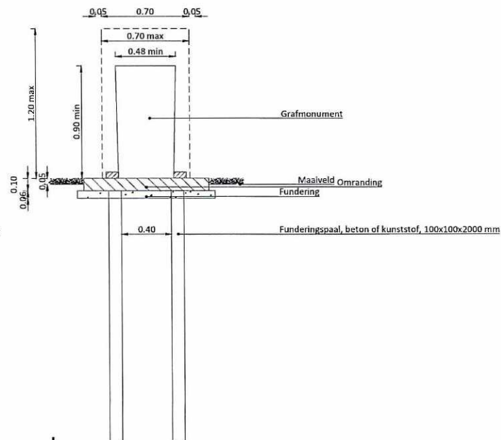
Steenmodel M5-3 Vooraanzicht Schaal 1:20
