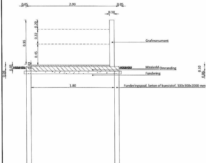
Steenmodel M4-2 Zijaanzicht Schaal 1:20
