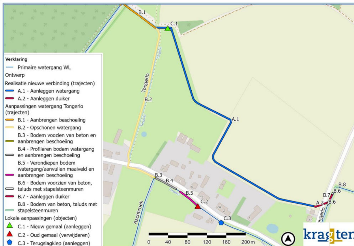
Abbeelding 1. Overzicht werkzaamheden gemaal Tongerlo.
