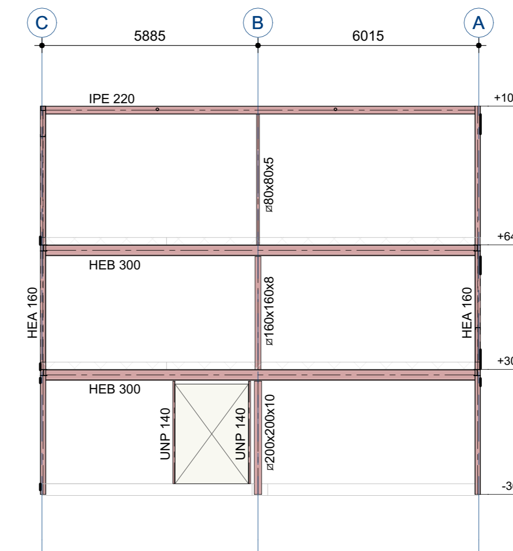
STAALANZICHT AS 6
