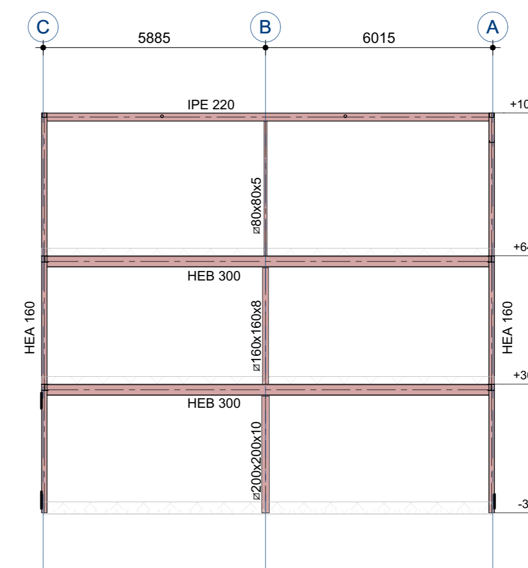
STAALANZICHT AS 7
