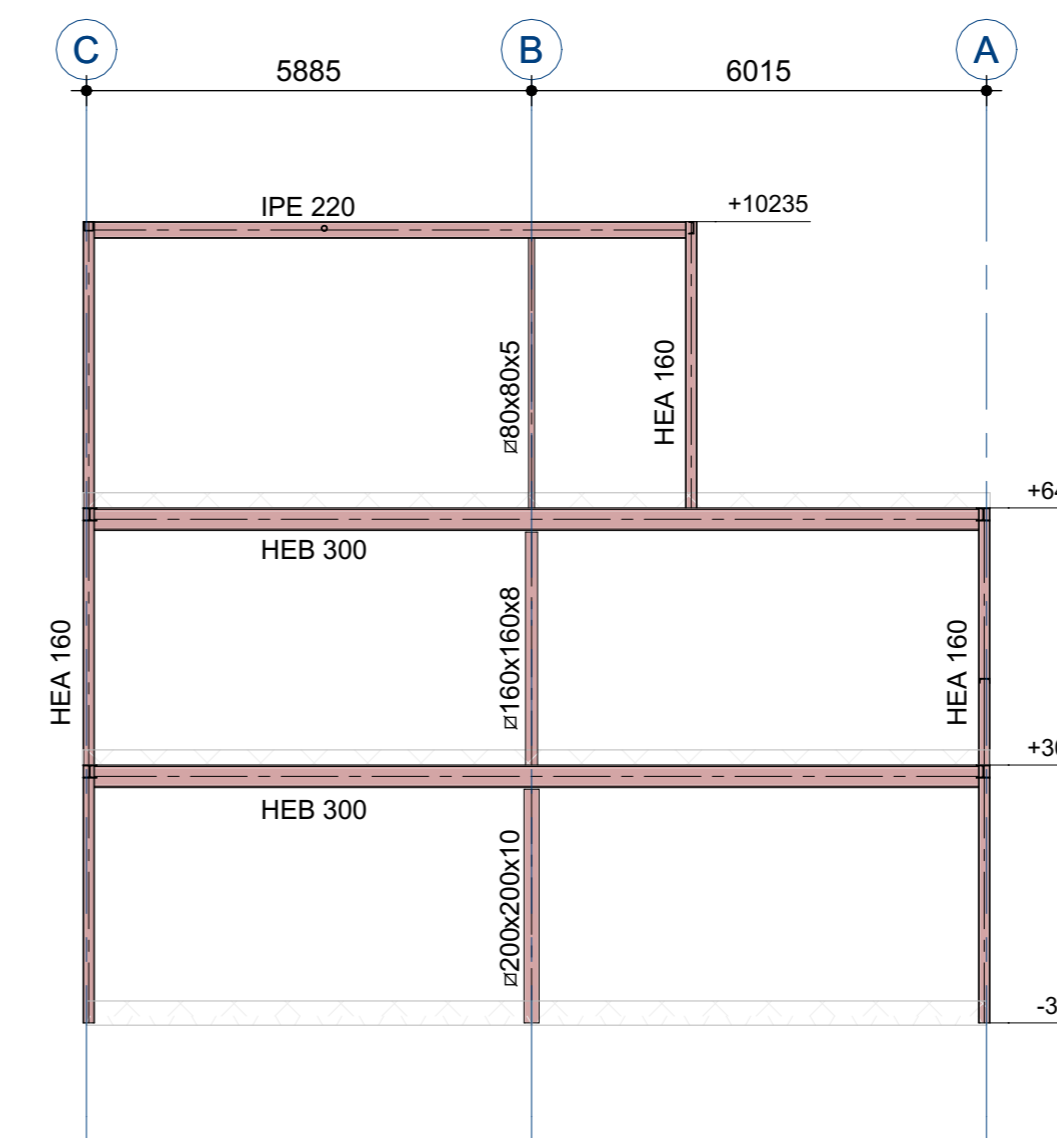
STAALANZICHT AS 4
