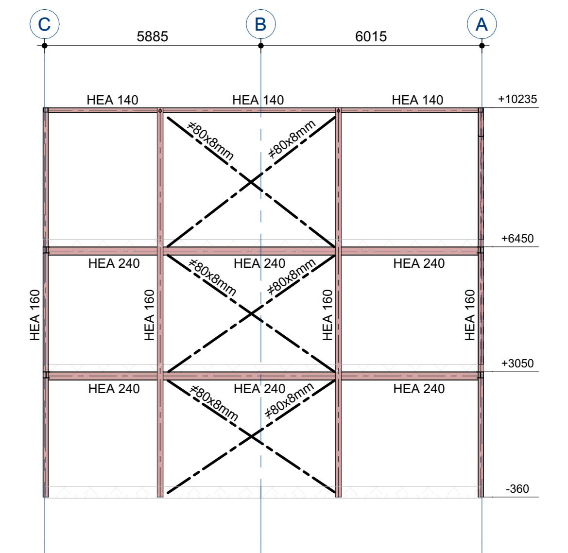
STAALANZICHT AS 8
