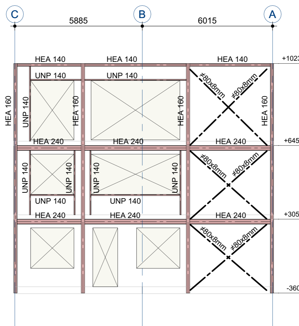
STAALANZICHT AS 1
