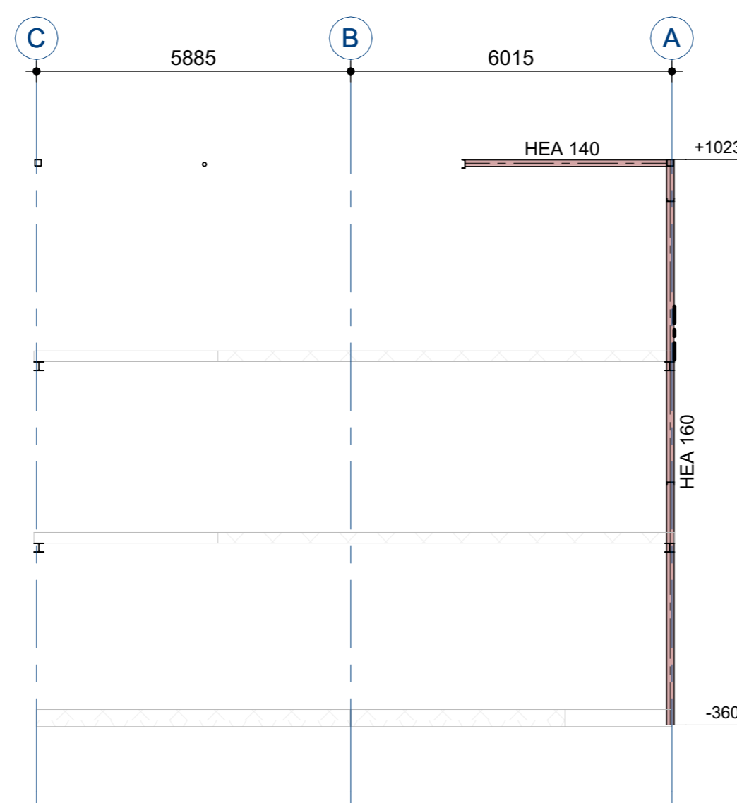
STAALANZICHT AS 3
