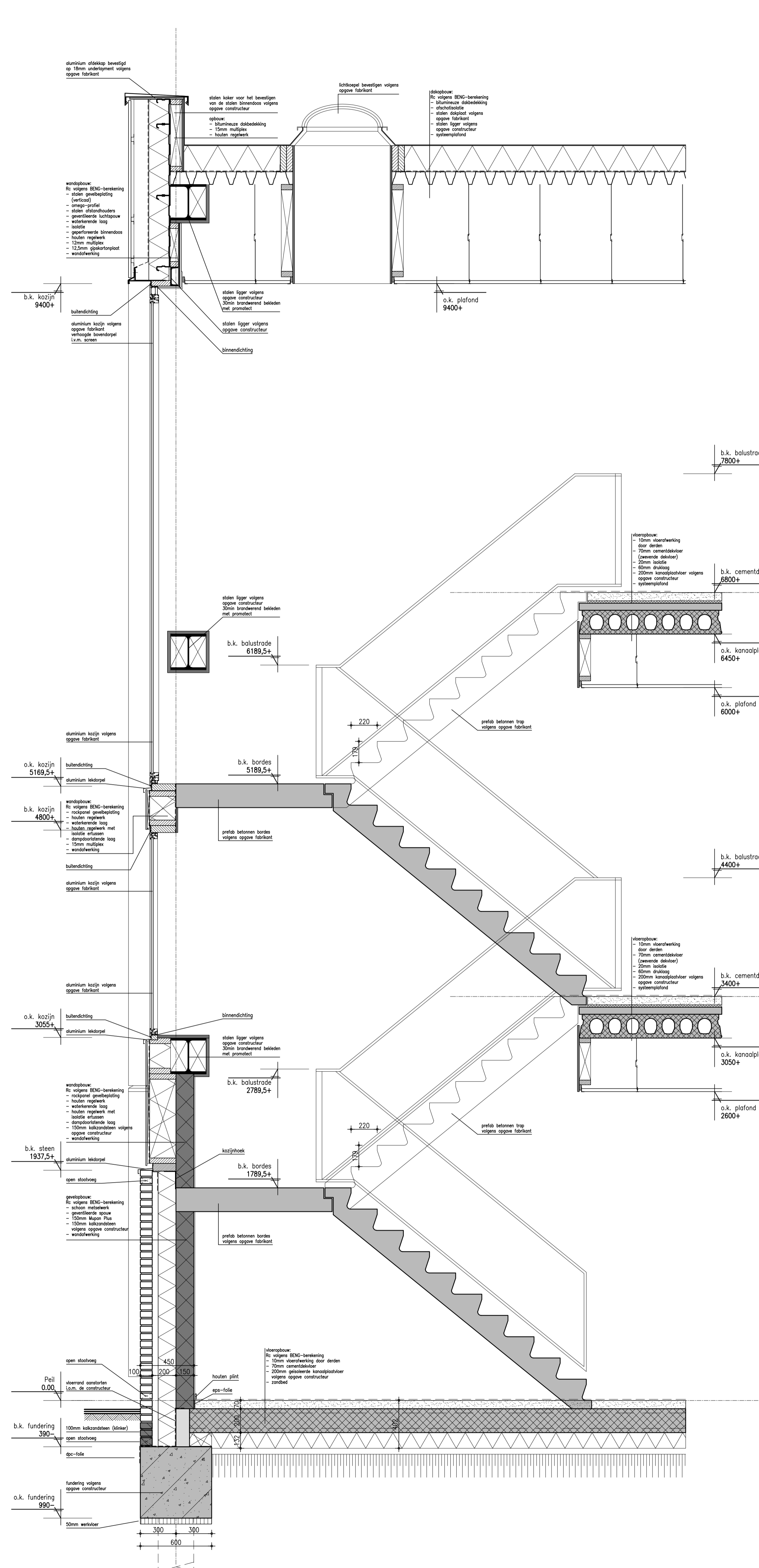
- Doorsnede 05 - schaal 1:20
