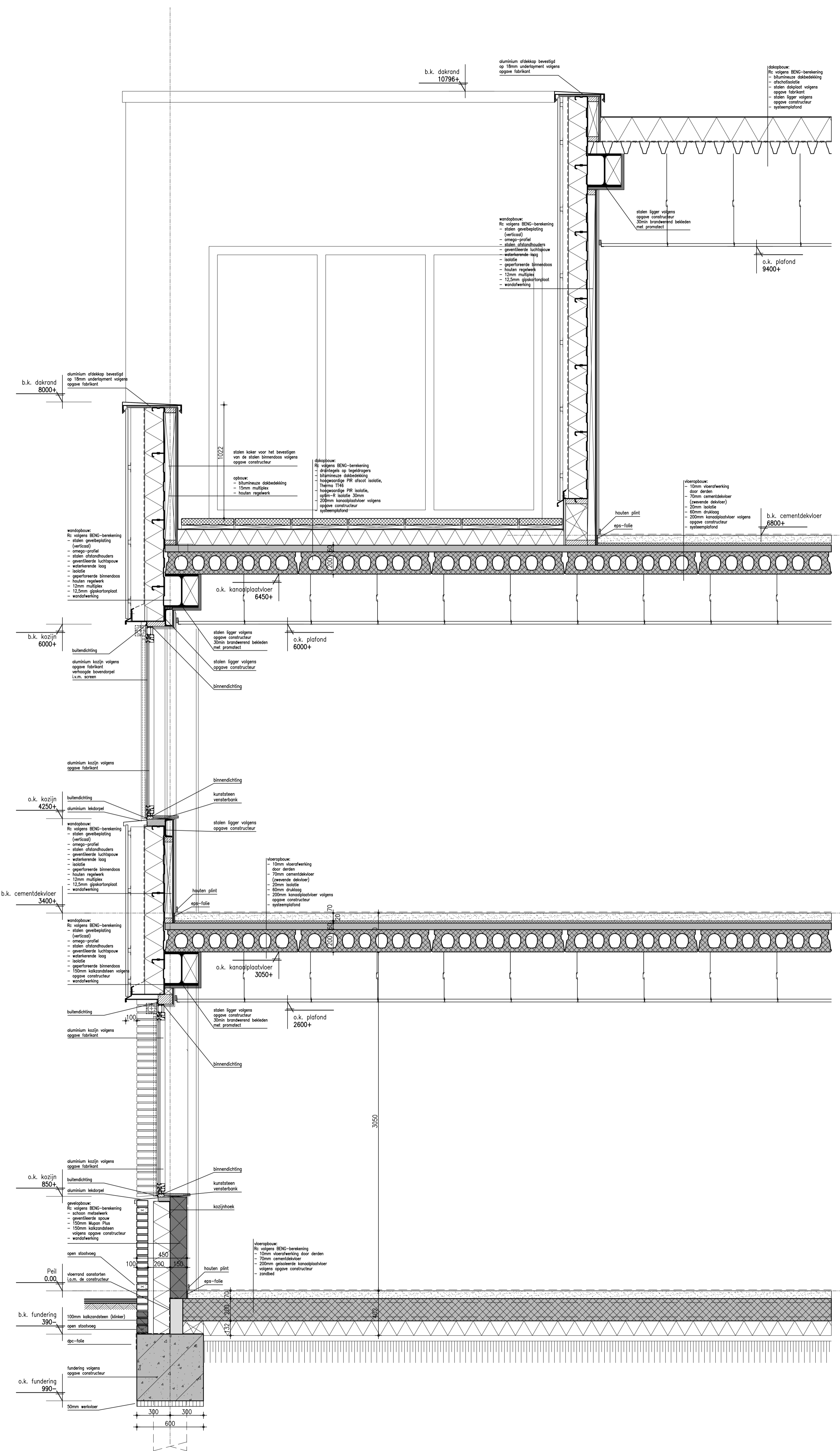
- Doorsnede 01 - schaal 1:20
