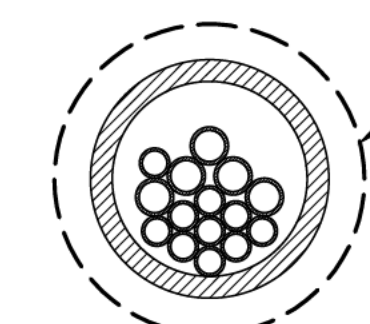
BOORGANG: Ø4,11mm 1x BUS HPE Ø315mm PE100 SDR11 (t.b.v.: MANTELBUISZIJN VULLINGSGRAAD 43% MET DAARIN: 10x BUS HPE Ø40mm PE100 SDR11 5x BUS HPE Ø50mm PE100 SDR11
