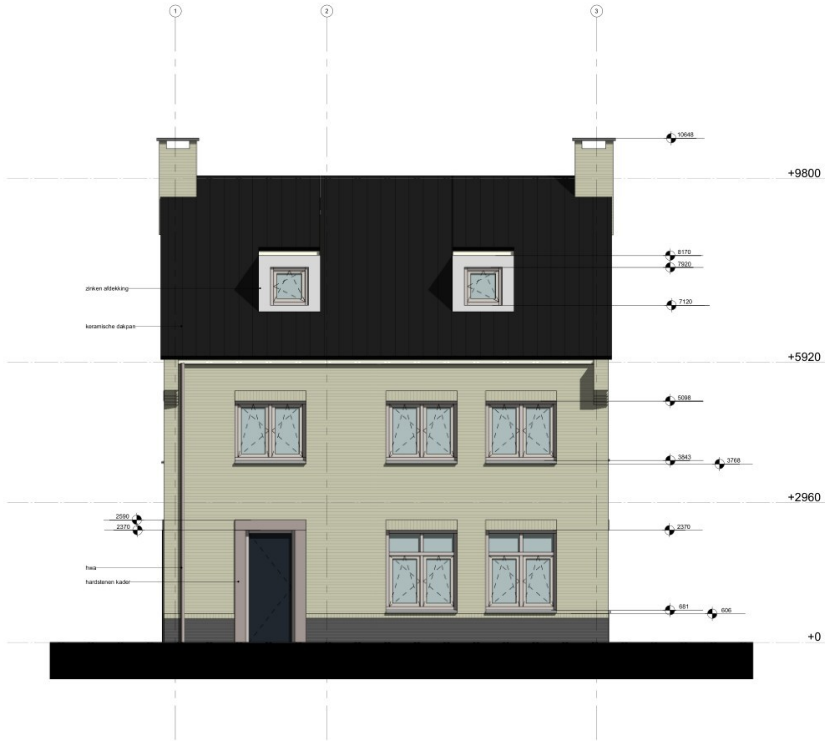
1 Voorgevel 1 : 50
