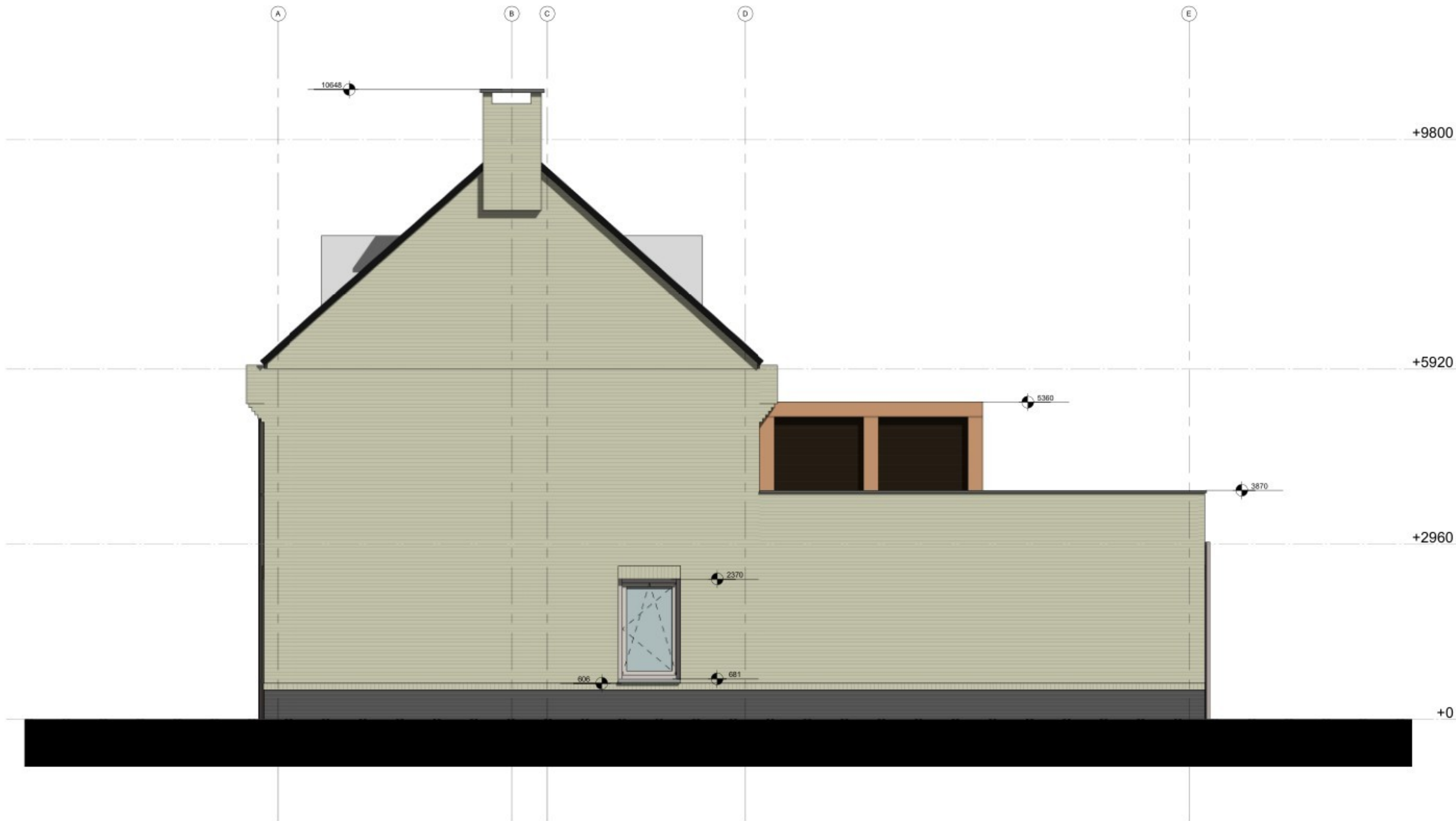
2 Rechtergevel 1 : 50
