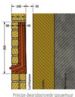
Principe dwarsdoorsnede spouwmuur
