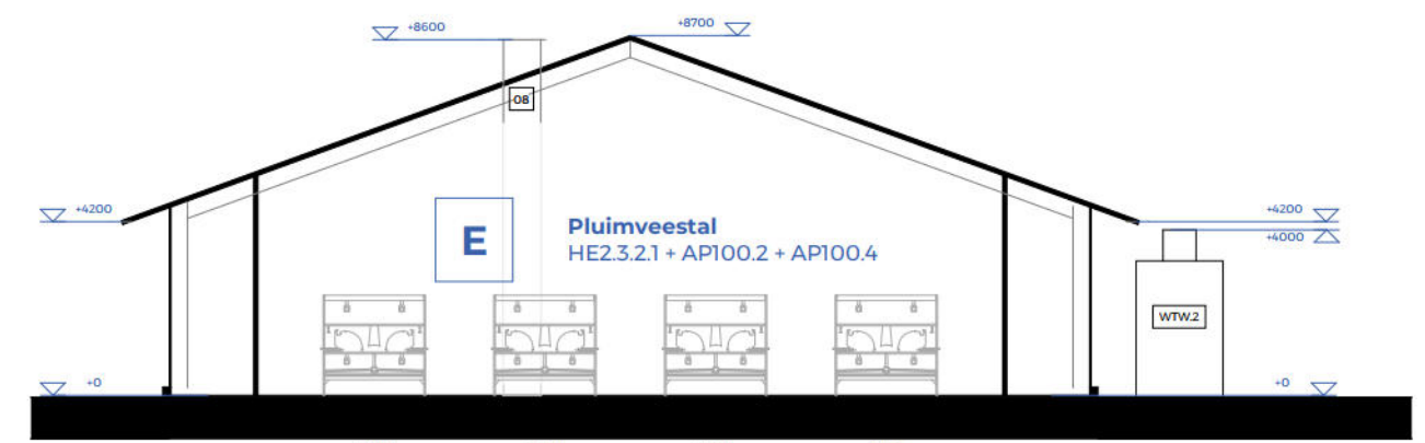
Gebouw E - stalruimte 1:200
