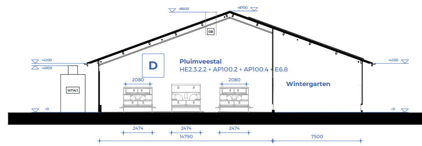
Gebouw D - stalruimte 1:200
