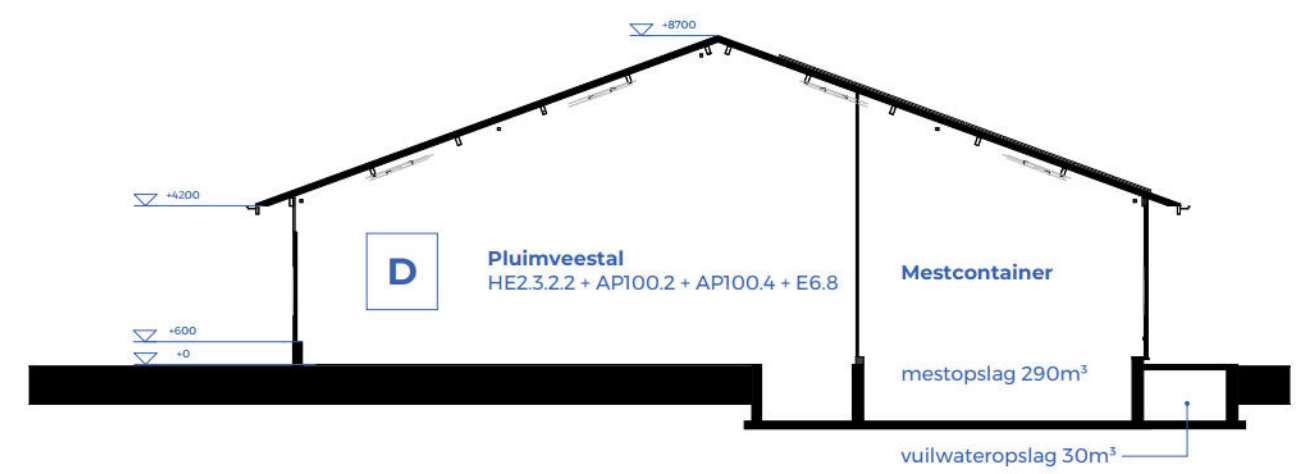
Gebouw D - achterruimte 1:200
