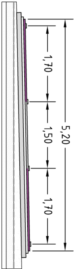
verhardingsprofiel op één oor
