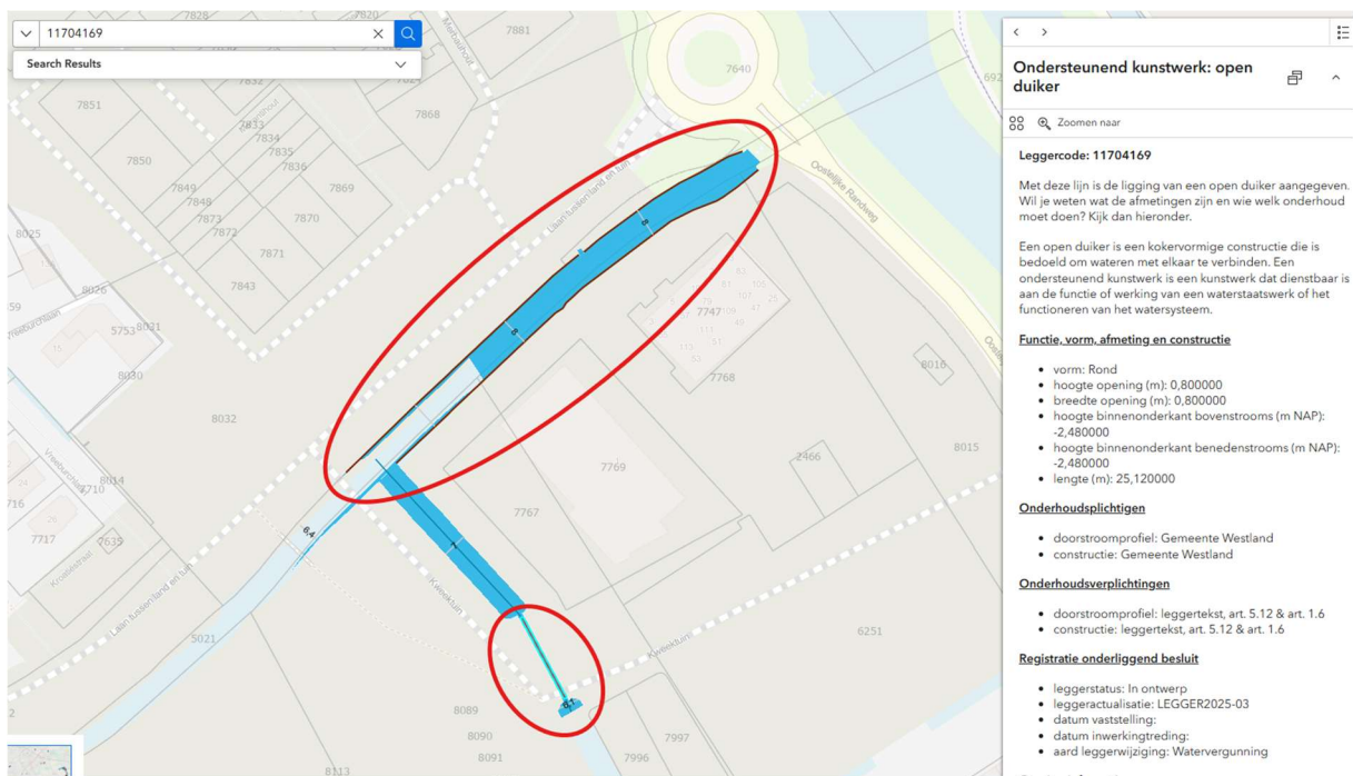
Figuur 4, Ontwerp-leggerwijzigingskaart LEGGER2025-03, van de open duiker en de oeverconstructies.
