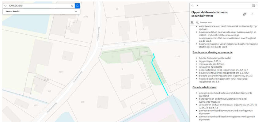
Figuur 6, Ontwerp-leggerwijzigingskaart LEGGER2025-03, van het secundair water.
