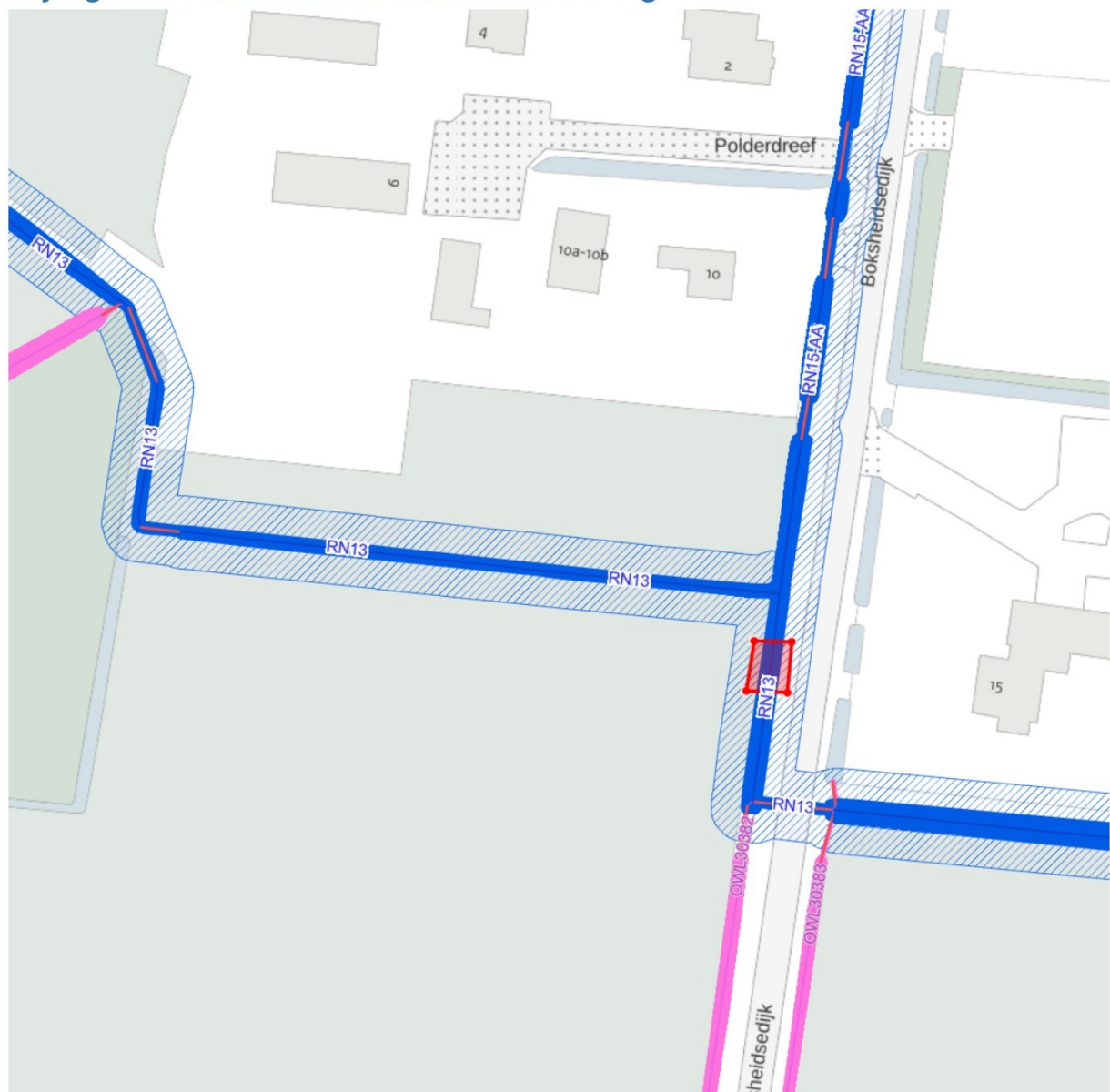
Figuur 1: Globale locatieaanduiding van de dam met duiker nabij de Boksheidsdijk in Eersel, ten zuiden van de Polderdreef. Het rode vlak is de locatie voor de dam met duiker. Het blauwe vlak zijn a-wateren, het roze vlak zijn b-wateren. De rode lijnen zijn duikers.
