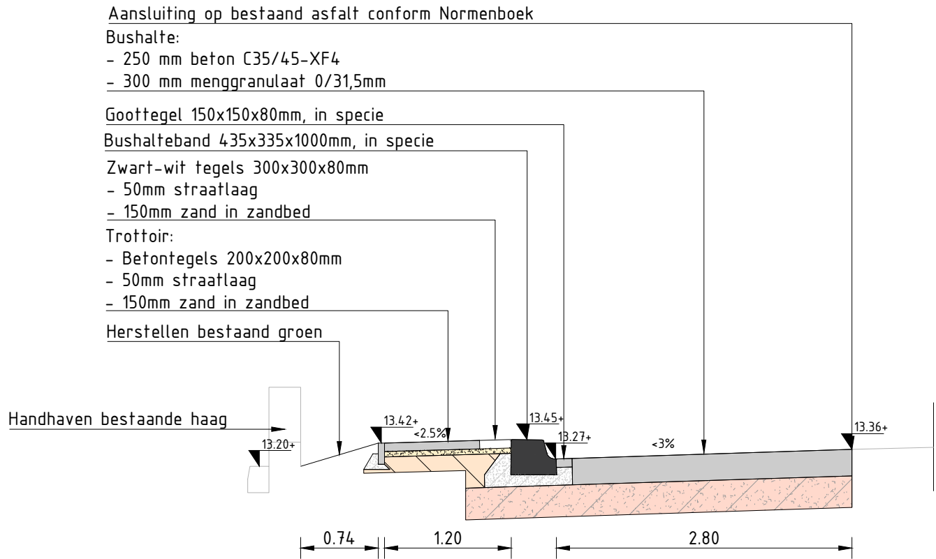
Locatie 6 | Ringbaan Oost - Eekhofstraat Oost Schaal 1:50
