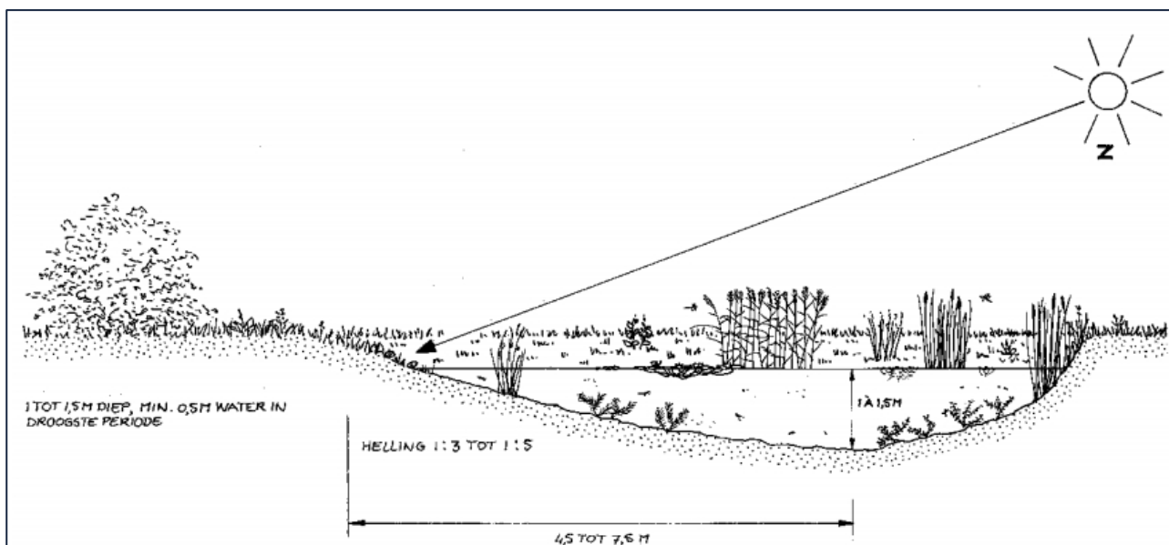
Afbeelding 3.3: Schematische dwarsdoorsnede van een poel die geschikt is voor amfibieën (Stichting vitaal platteland, z.d.).
