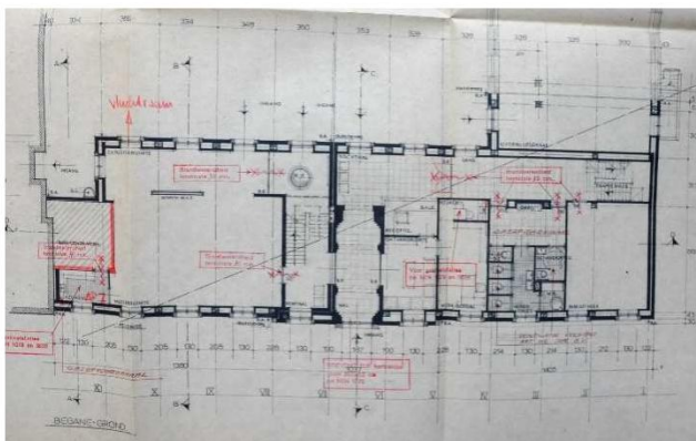
15 Plattegrond van de nieuwe toestand van de begane grond van de westvleugel, 1977. Alle zwart ingekleurde muren zijn nieuw geplaatst.
