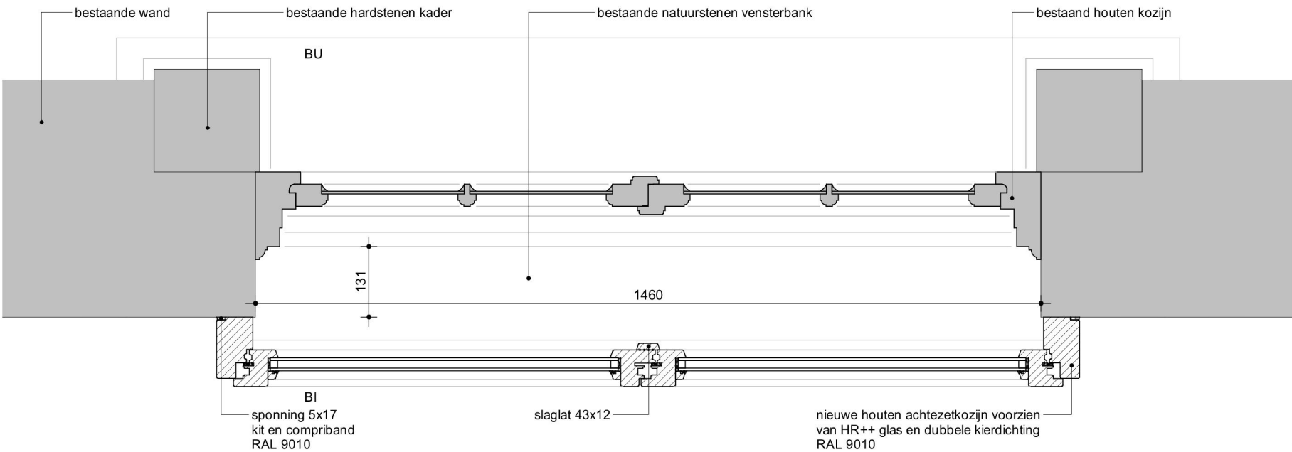
Merk 5C.08 - Nieuw detail N40-H
