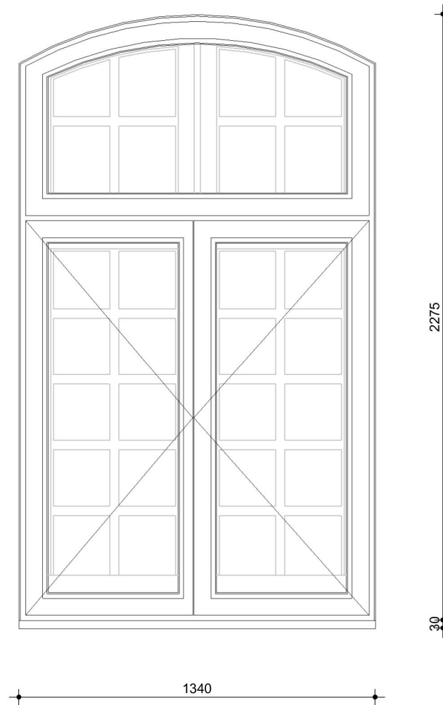
Merk 5C.06 - binnenaanzicht nieuw
