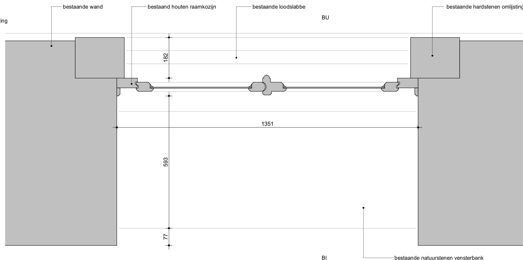
Merk 5A.04 - Bestaand detail B08-H
