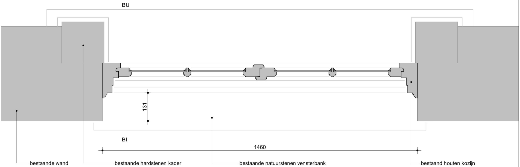
Merk 5C.08 - Bestaand detail B40-H
