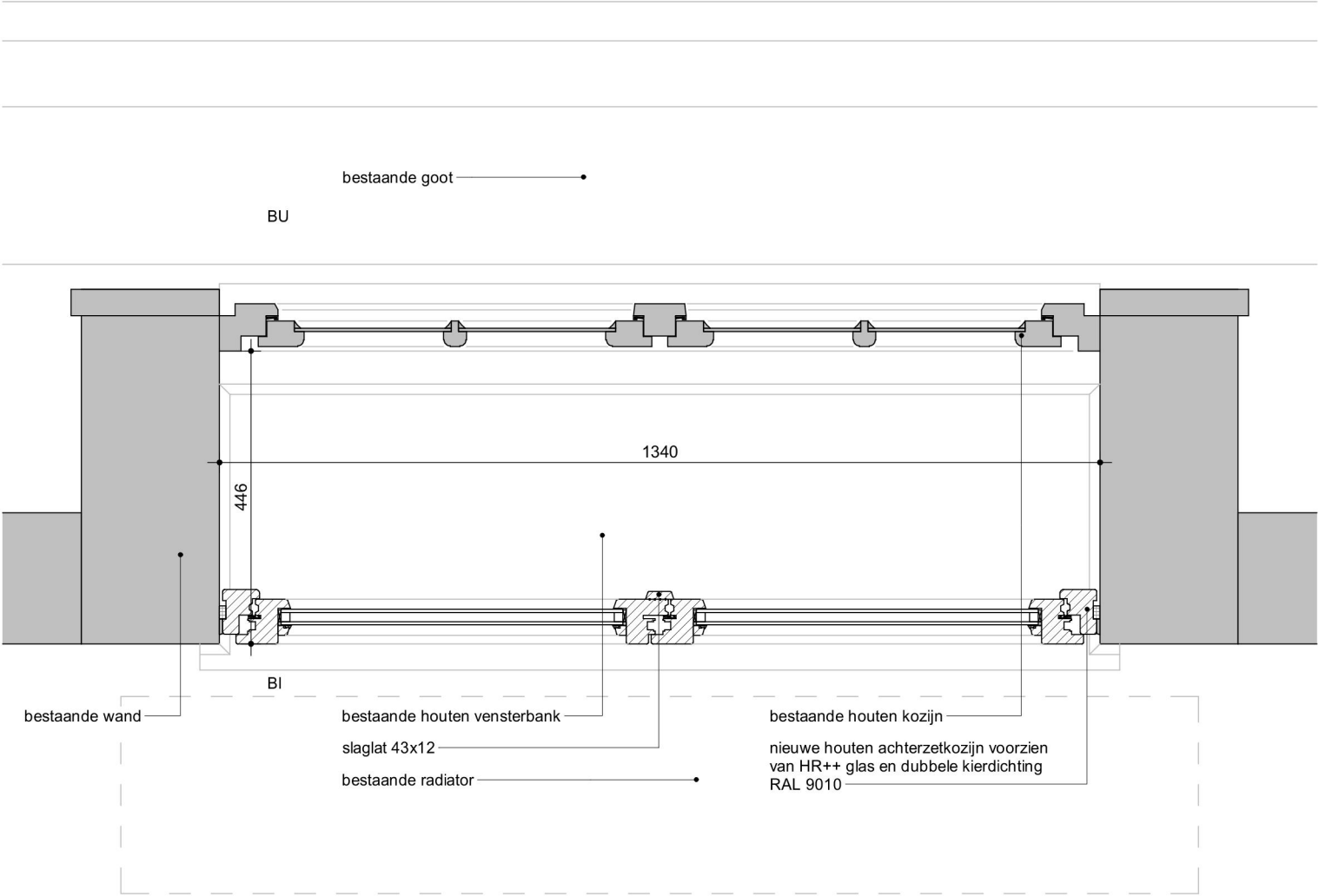
Merk 5C.05 - Nieuw detail N34-H
