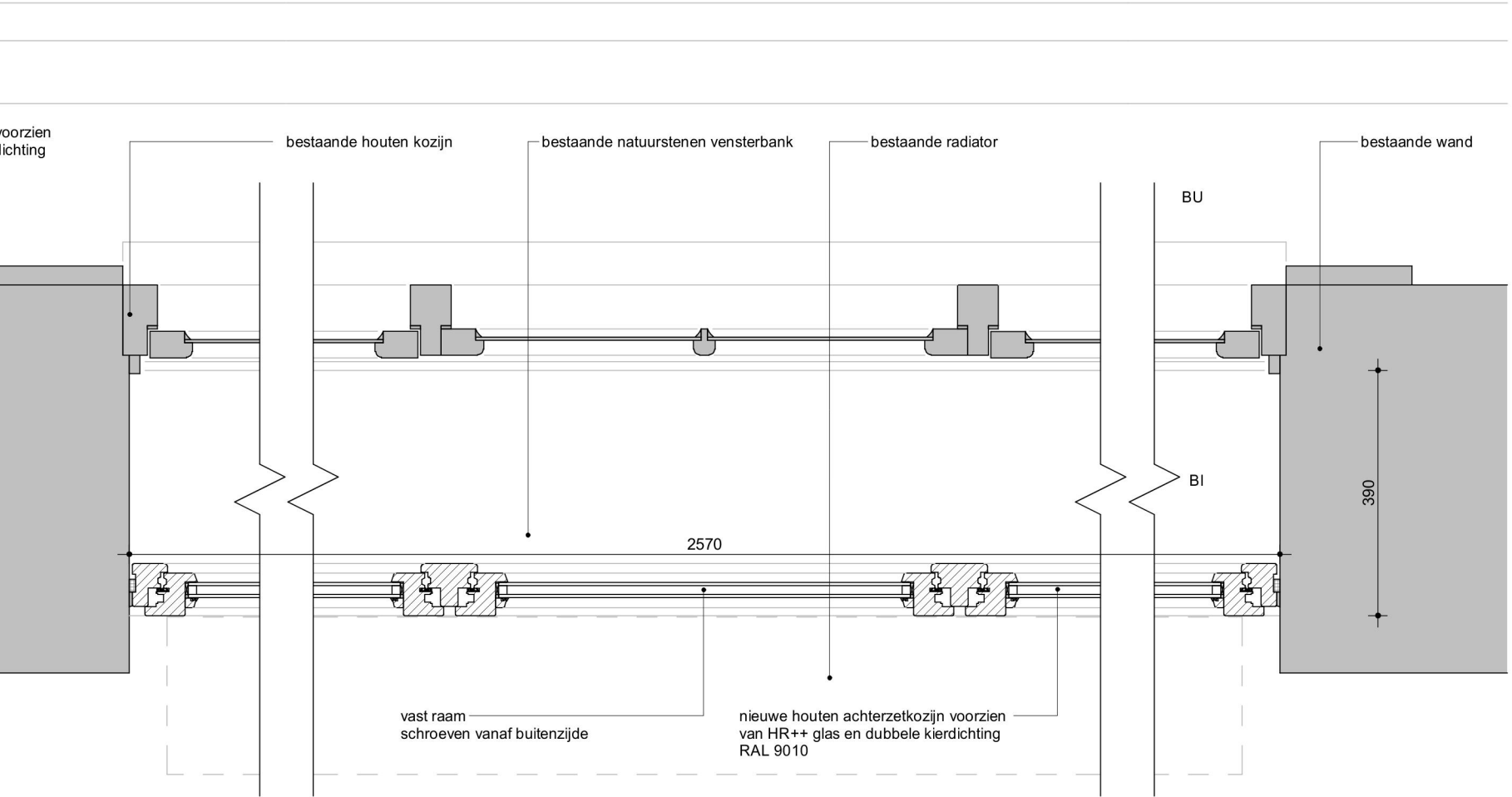
Merk 5C.07 - Nieuw detail N38-H
