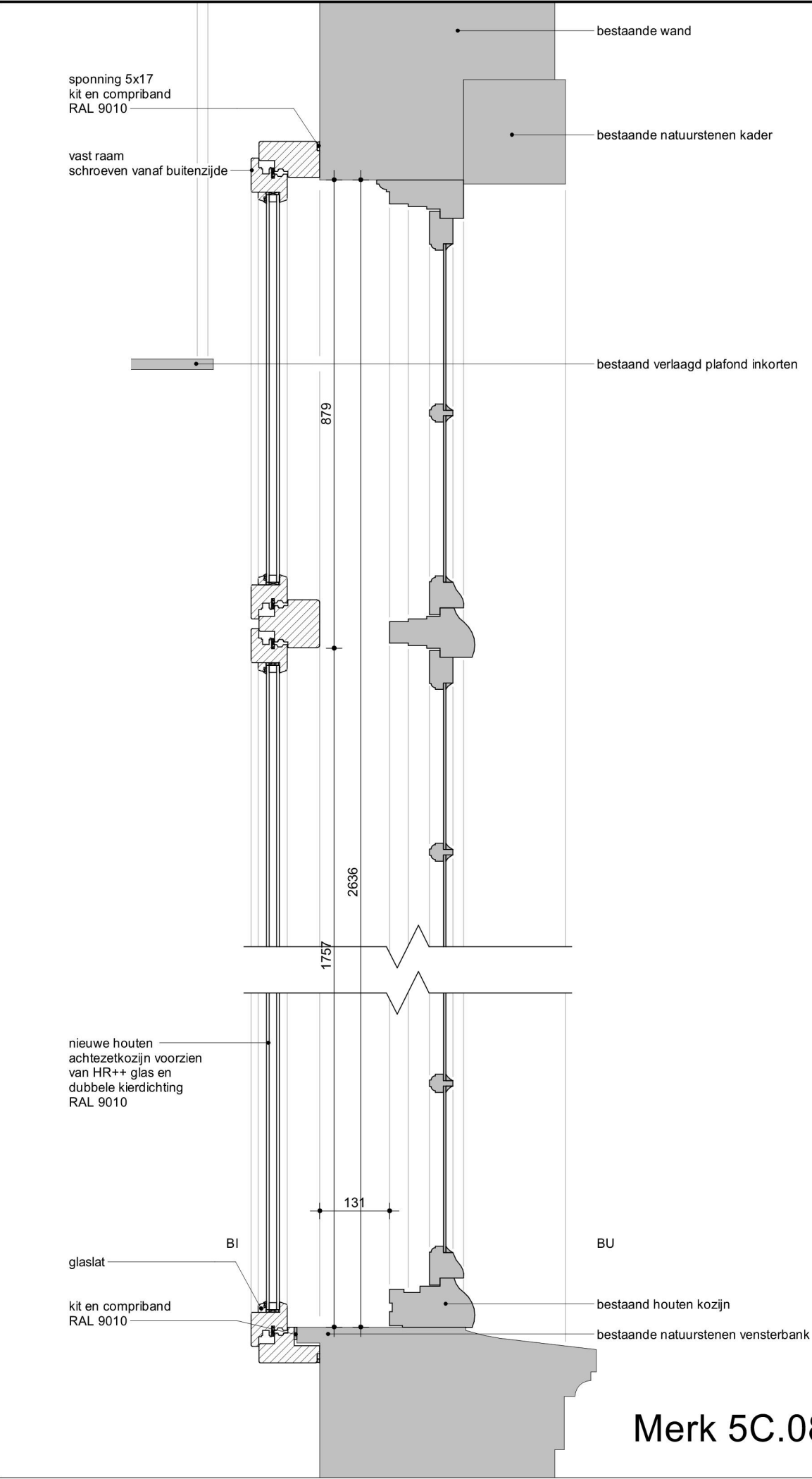
Merk 5C.08 - Nieuw detail N40-H
