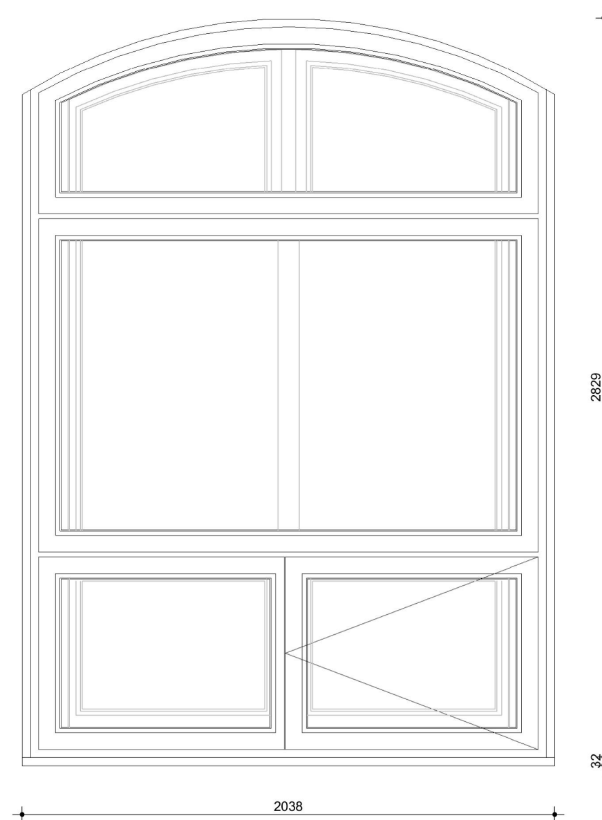
Merk 5C.03 - binnenaanzicht nieuw
