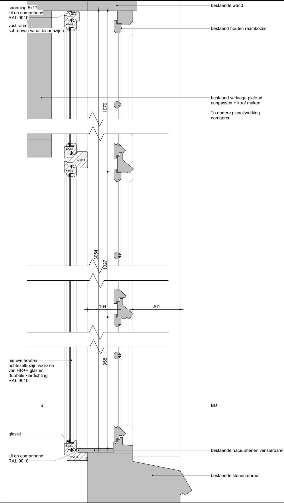
Merk 5B.01 - Nieuw detail N12-H
