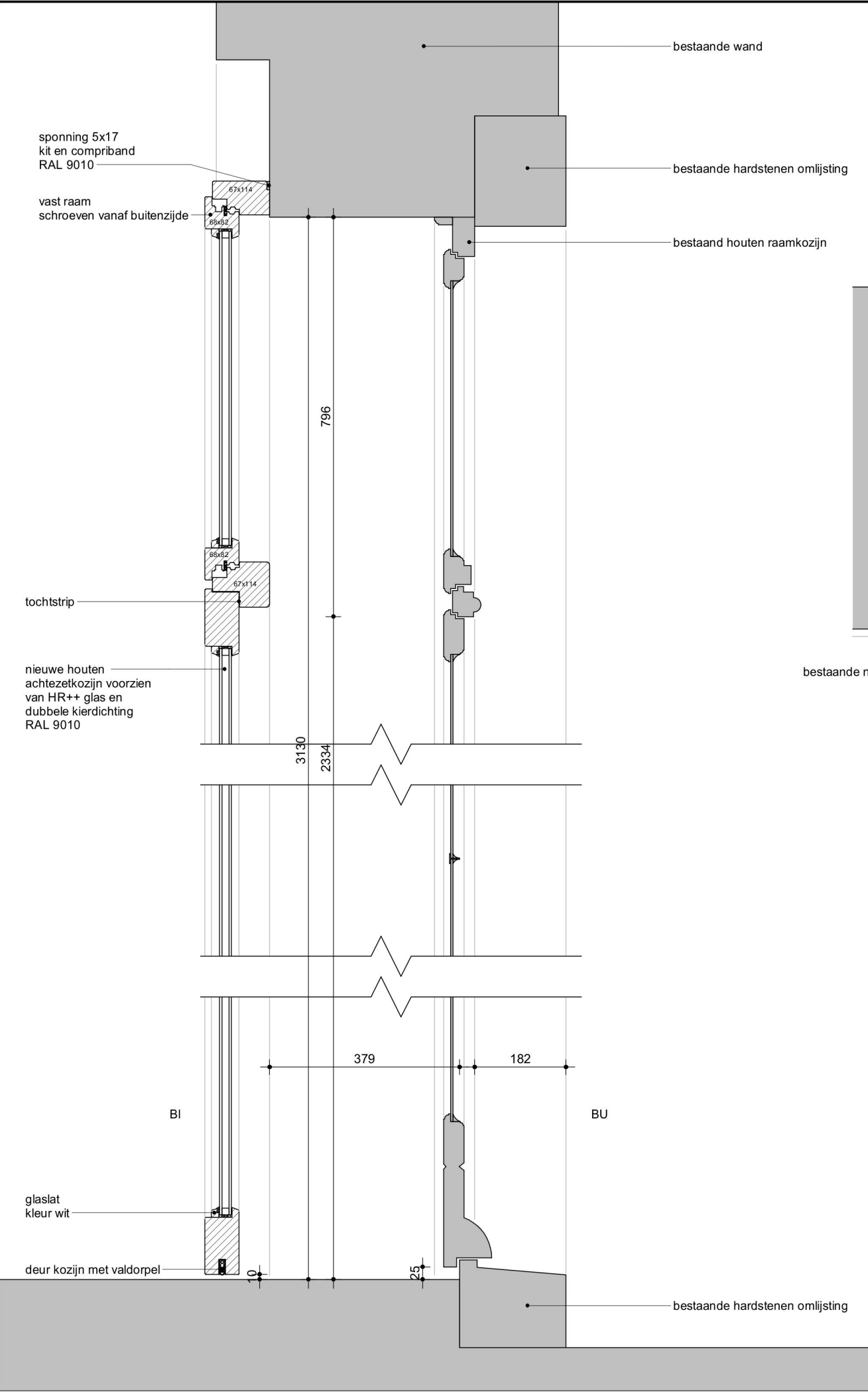
Merk 5A.01 - Nieuw detail N02-H
