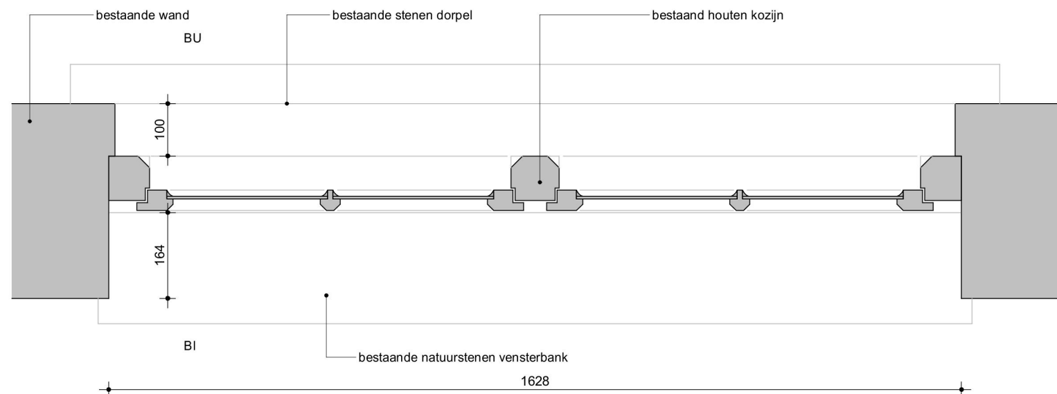
Merk 5B.07 - Bestaand detail B24-H
