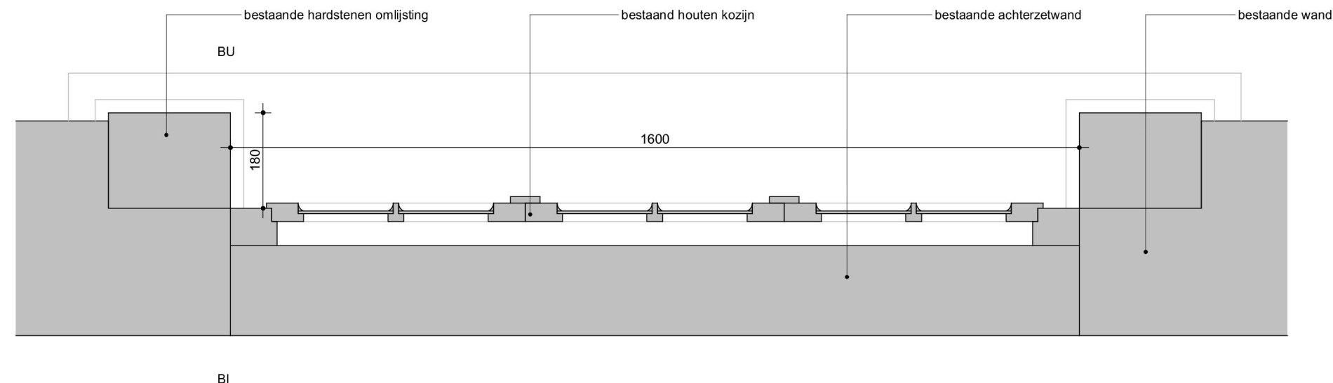
Merk 5C.04 - Bestaand detail B32-H
