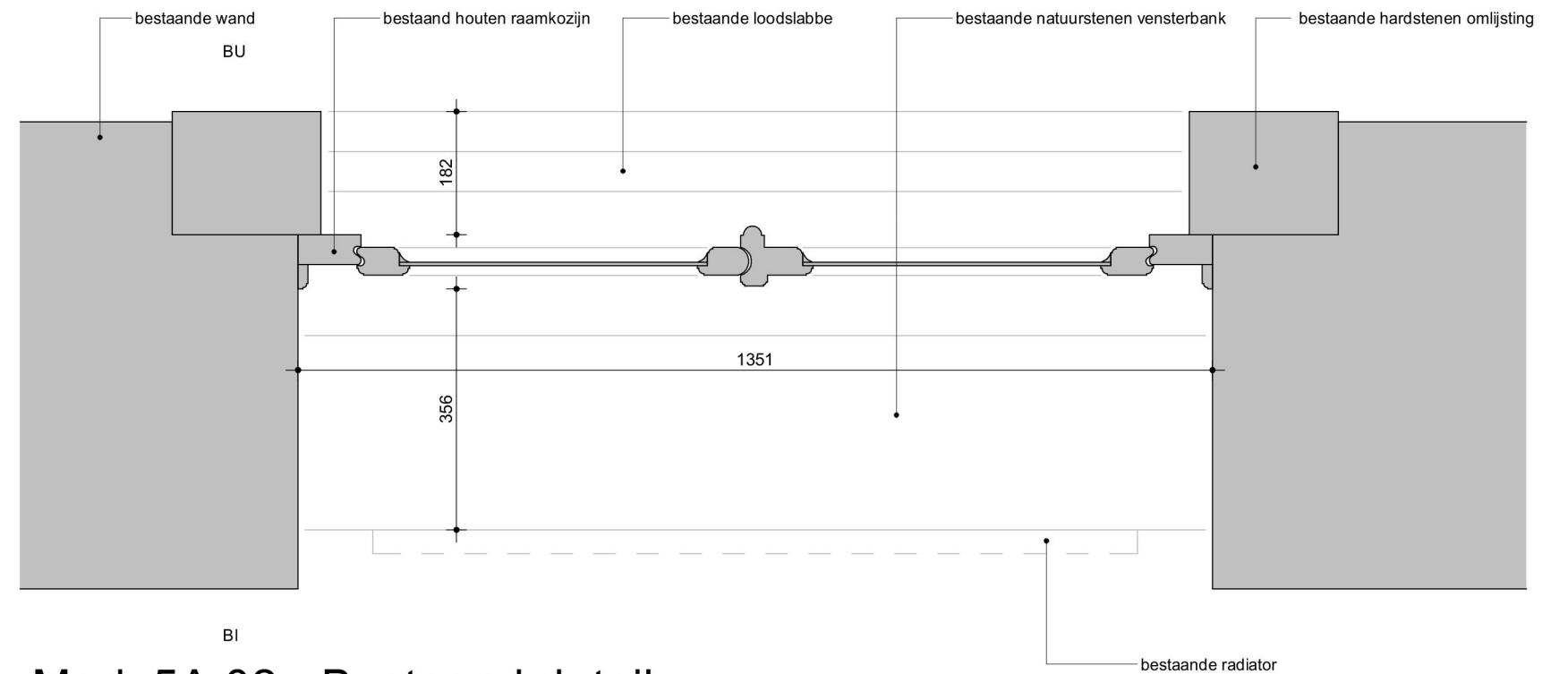
Merk 5A.02 - Bestaand detail B04-H
