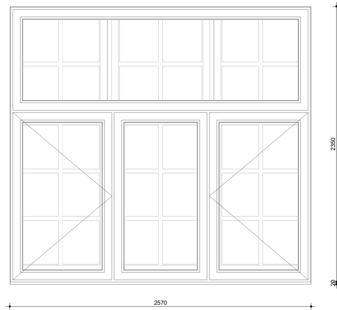
Merk 5C.07 - binnenaanzicht nieuw
