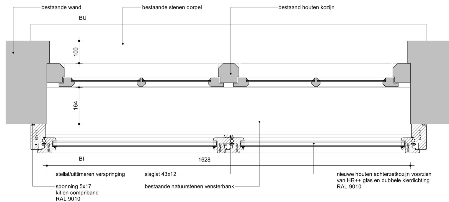
Merk 5B.07 - Nieuw detail N24-H
