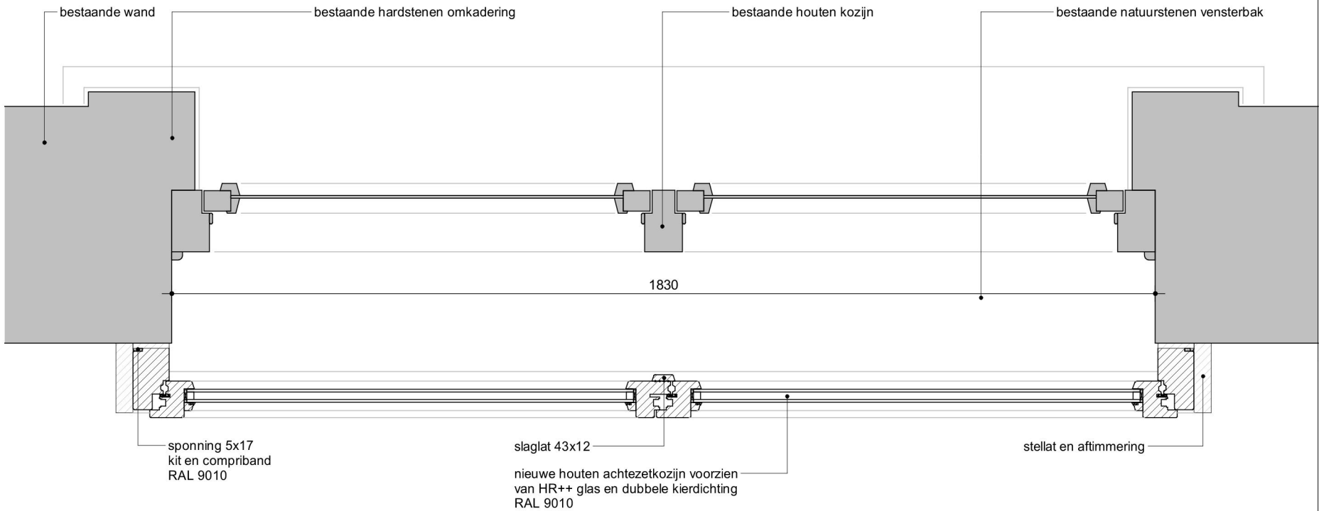
Merk 5C.03 - Nieuw detail N30-H
