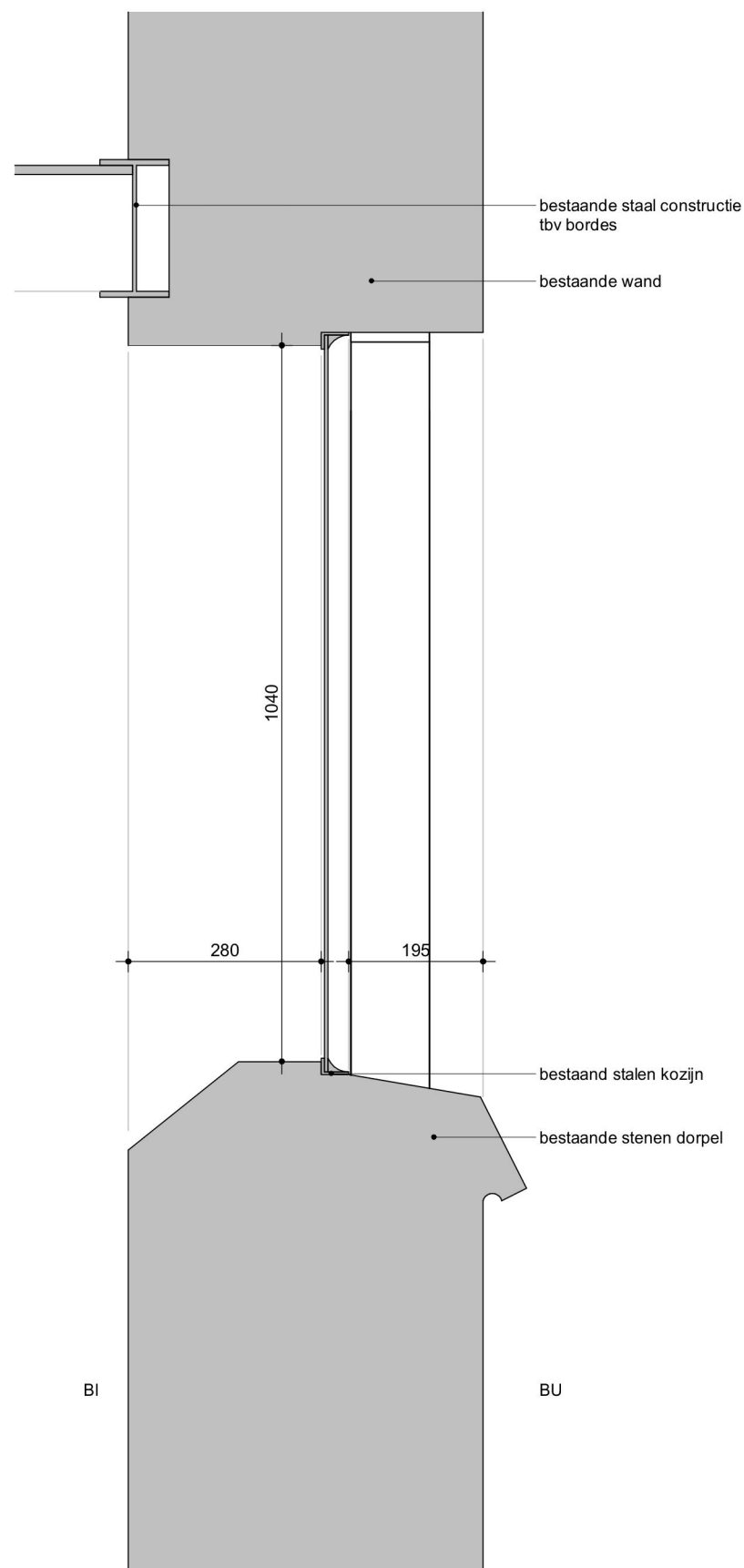
Merk 5B.04 - Bestaand detail B17-V
