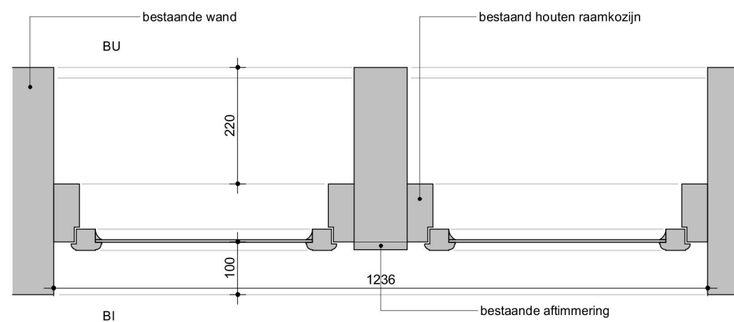
Merk 5B.02 - Bestaand detail B14-H
