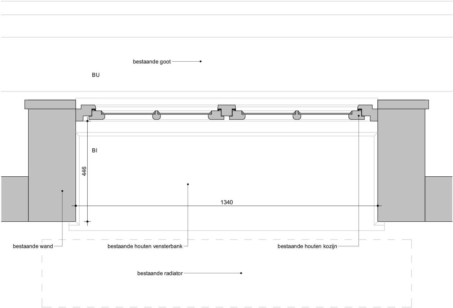
Merk 5C.05 - Bestaand detail B34-H
