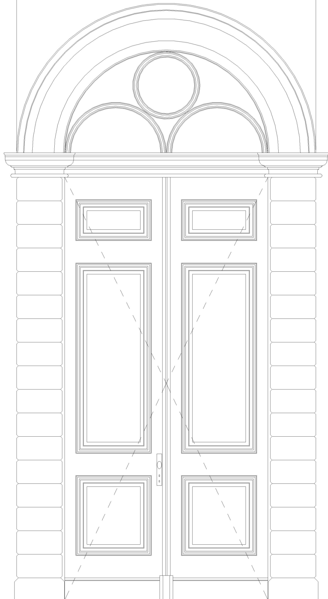
Merk 5A.03 - buitenaanzicht
