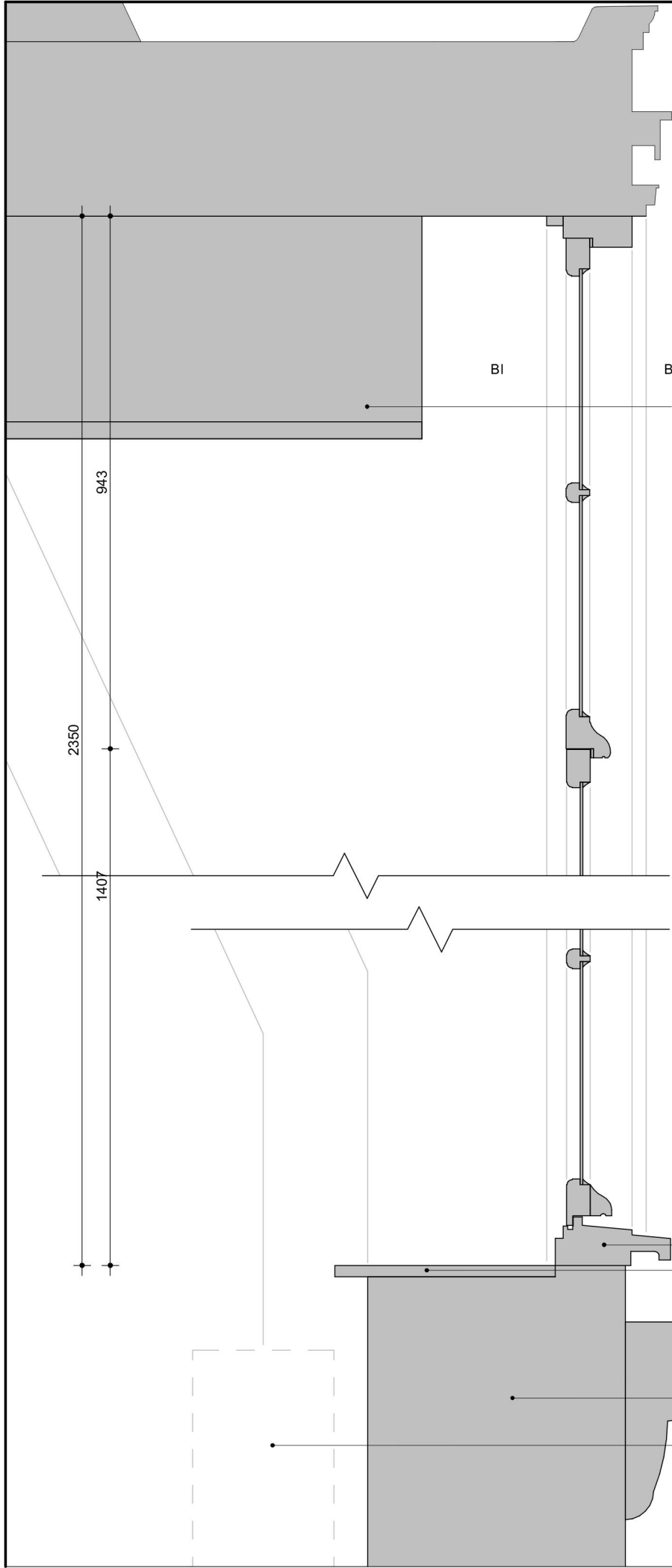
Merk 5C.07 - Bestaand detail B37-V
