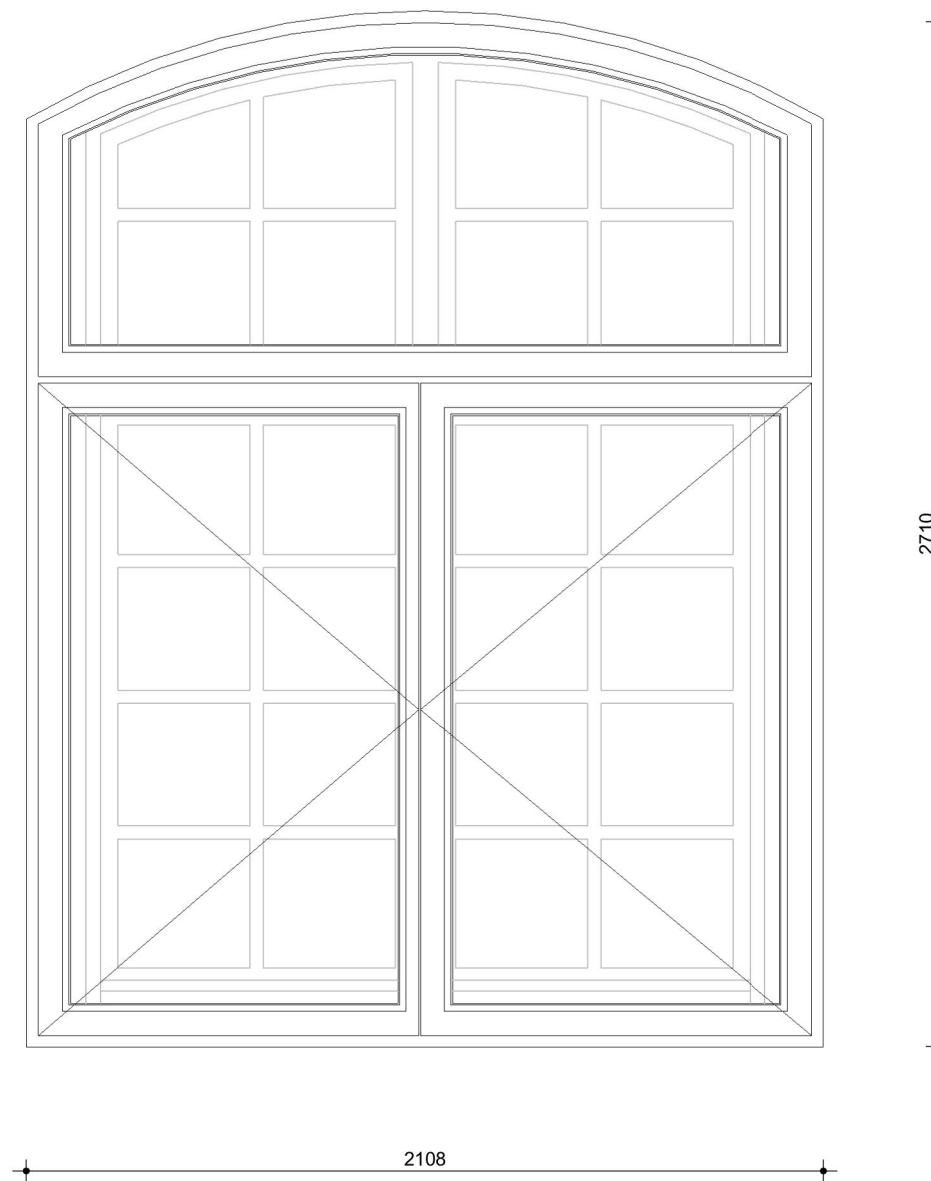
Merk 5C.01 - binnenaanzicht nieuw
