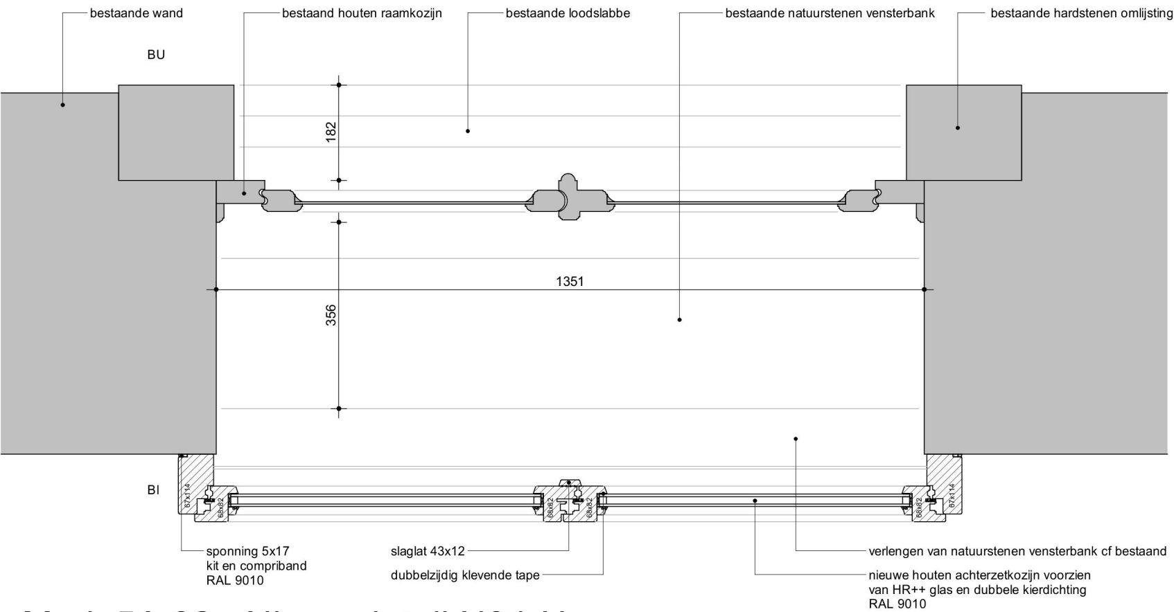
Merk 5A.02 - Nieuw detail N04-H
