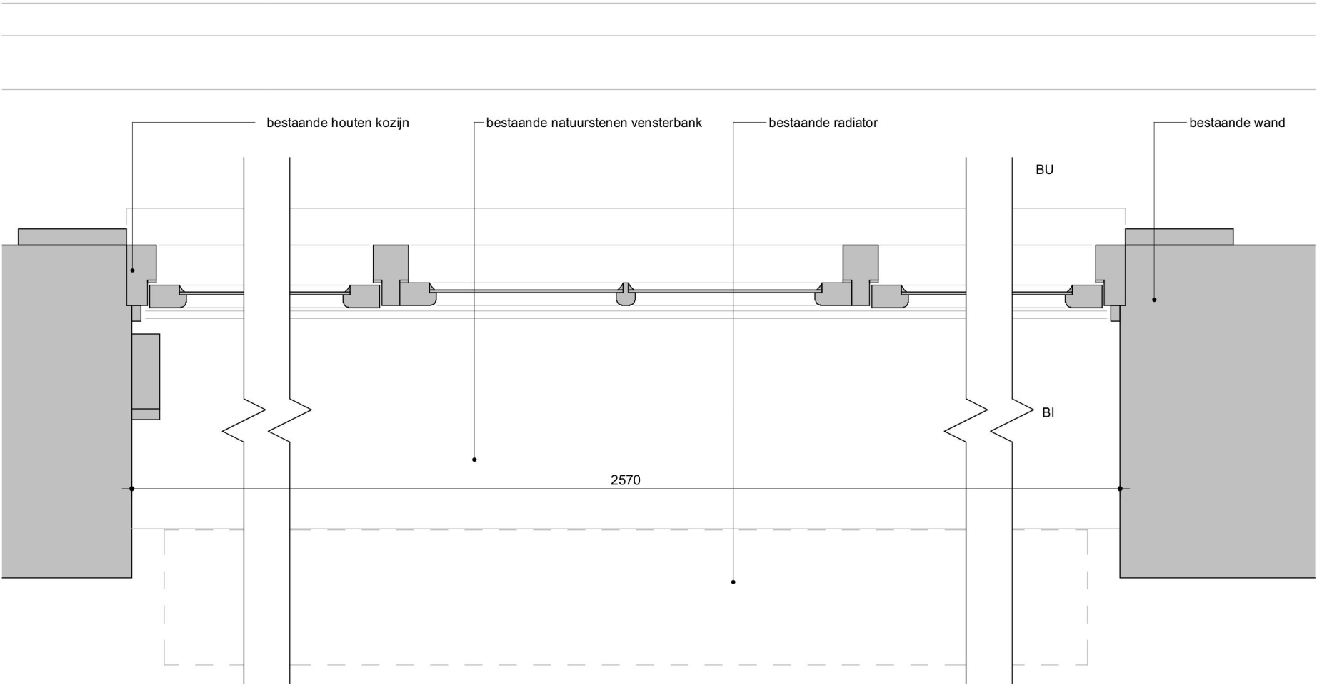
Merk 5C.07 - Bestaand detail B38-H
