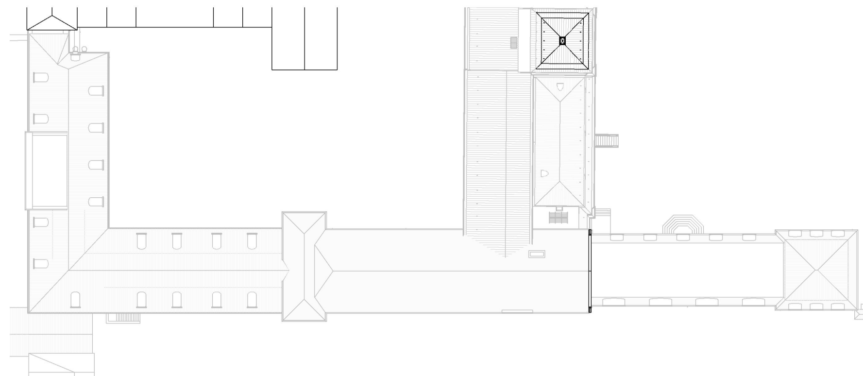
Dakaanzicht
