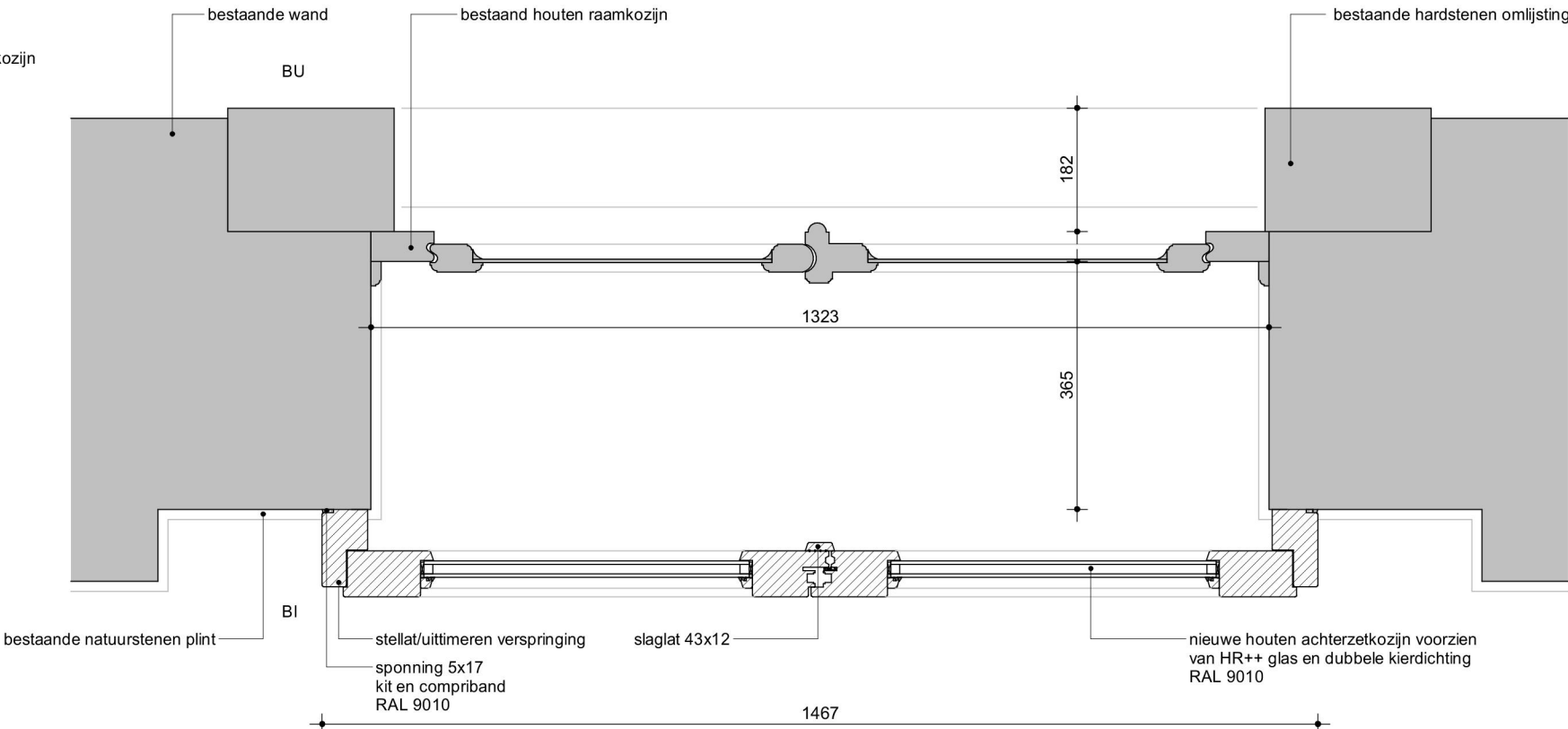
Merk 5A.01 - Nieuw detail N02-H
