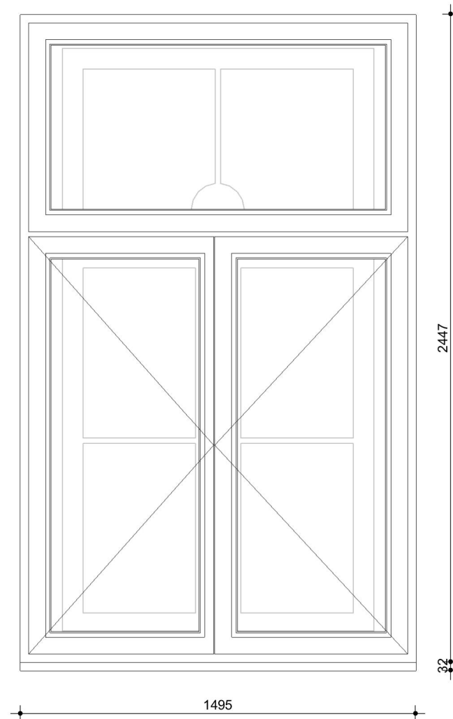
Merk 5A.04 - binnenaanzicht nieuw
