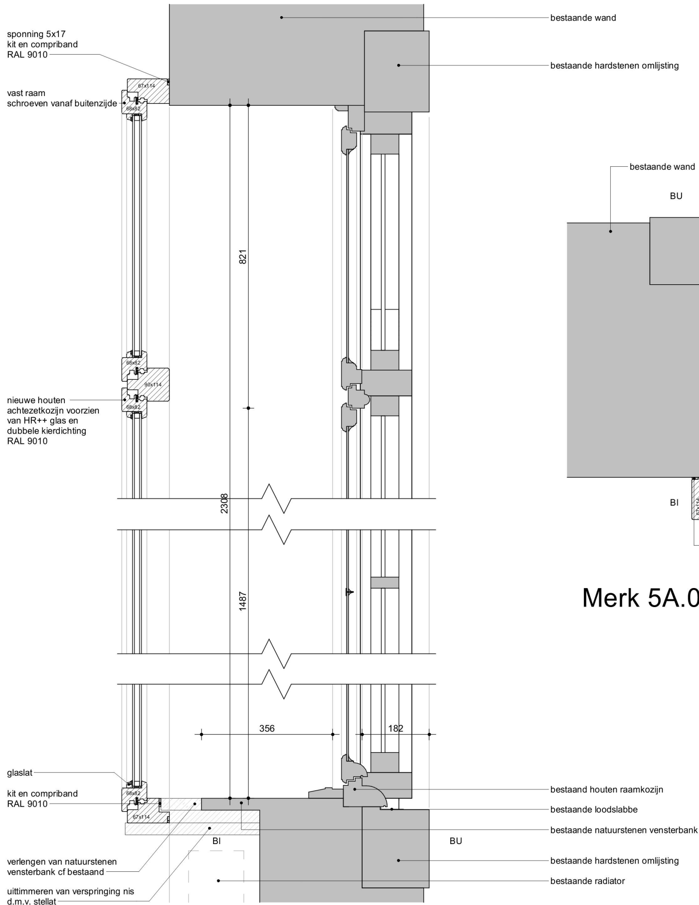
Merk 5A.02 - Nieuw detail N03-V
