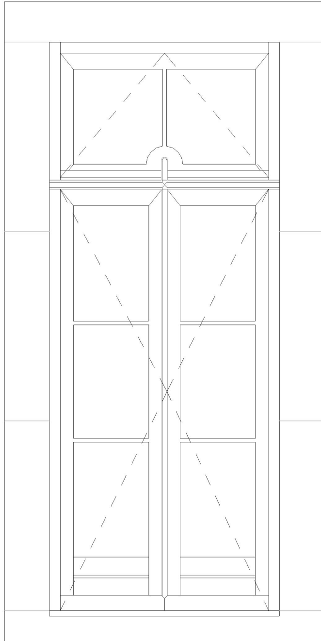
Merk 5A.01 - buitenaanzicht
