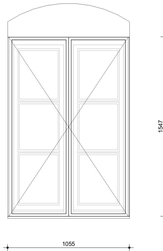
Merk 5A.05 - binnenaanzicht nieuw
