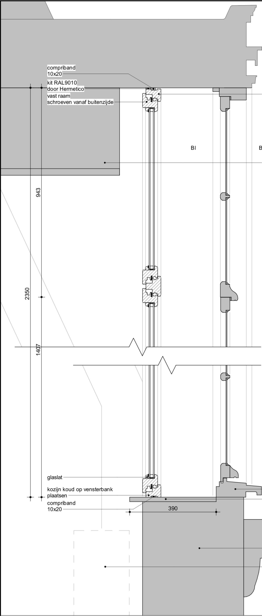
Merk 5C.07 - Nieuw detail N37-V
