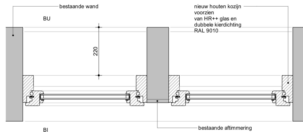
Merk 5B.02 - Nieuw detail N14-H
