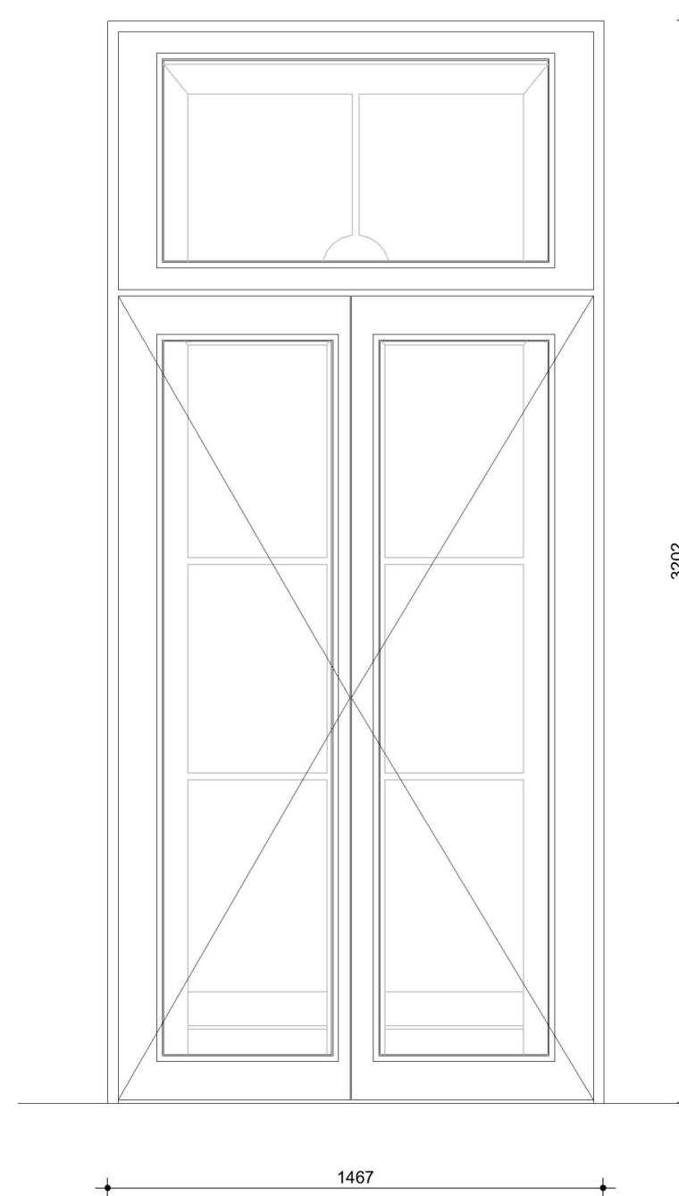
Merk 5A.01 - binnenaanzicht nieuw
