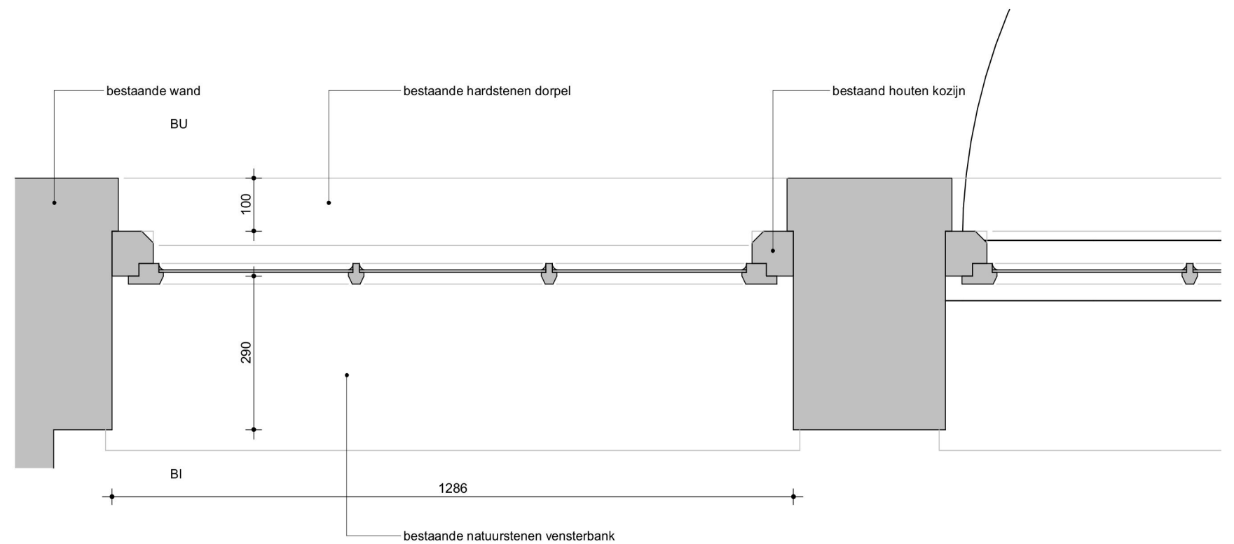
Merk 5B.06 - Bestaand detail B22-H
