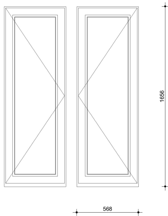
Merk 5B.02 - binnenaanzicht nieuw
