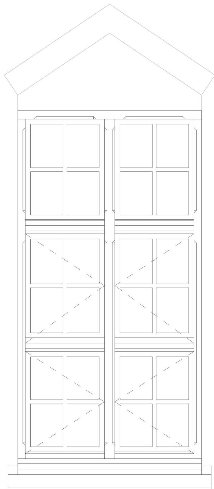
Merk 5B.01 - buitenaanzicht
