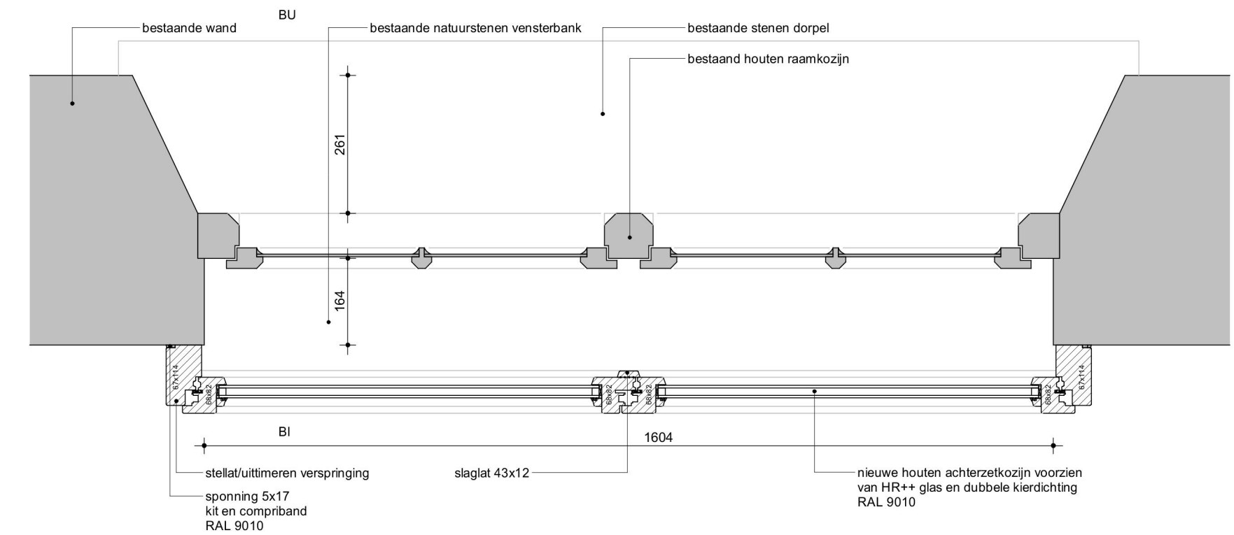
Merk 5B.01 - Nieuw detail N12-H
