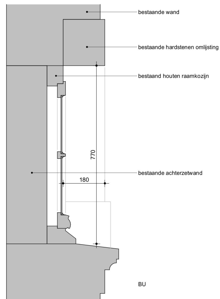
Merk 5C.04 - Bestaand detail B31-V
