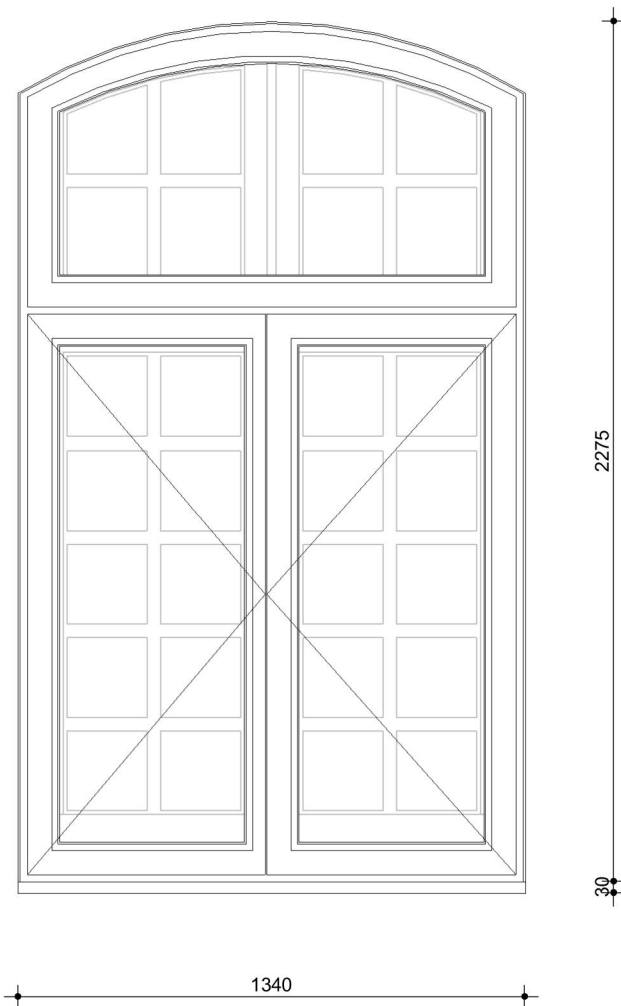
Merk 5C.05 - binnenaanzicht nieuw
