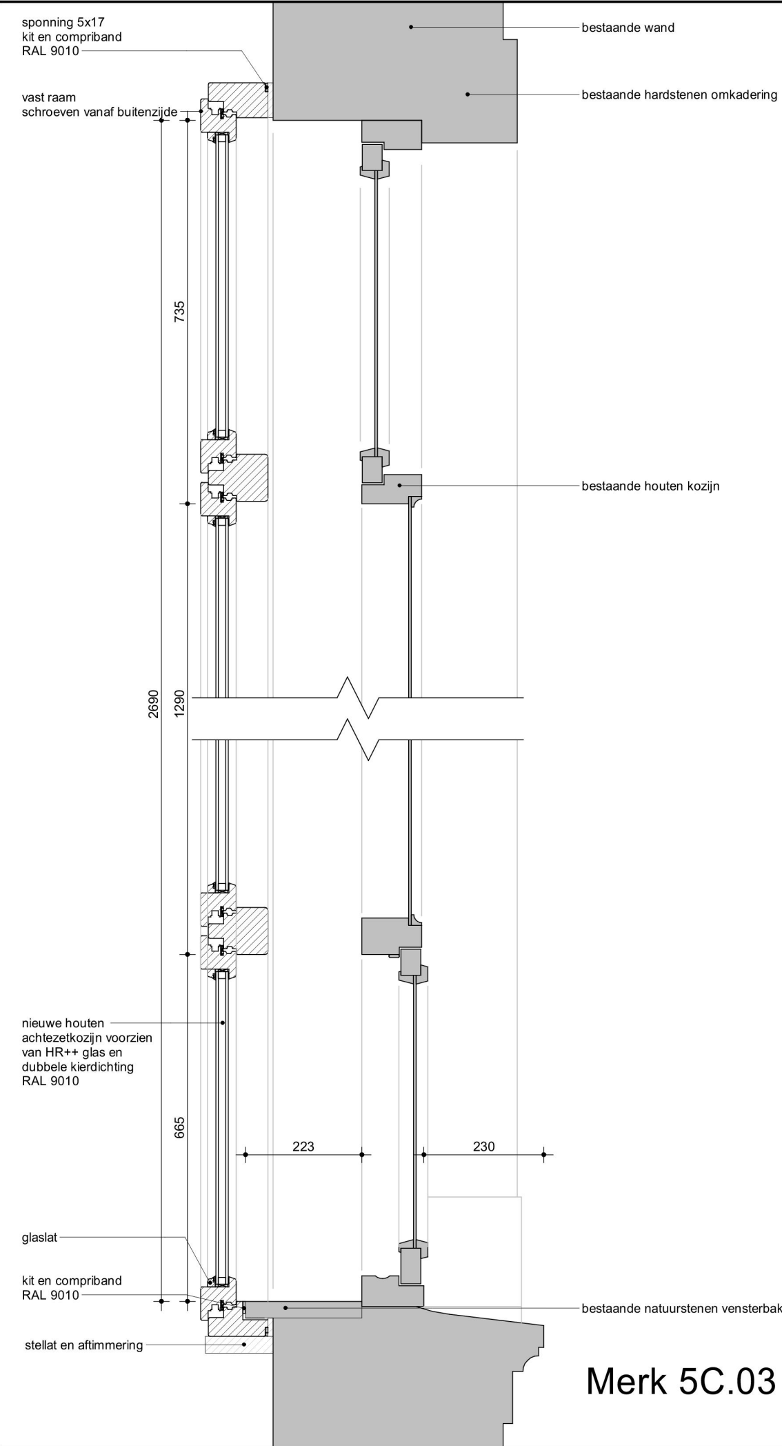
Merk 5C.03 - Nieuw detail N30-H
