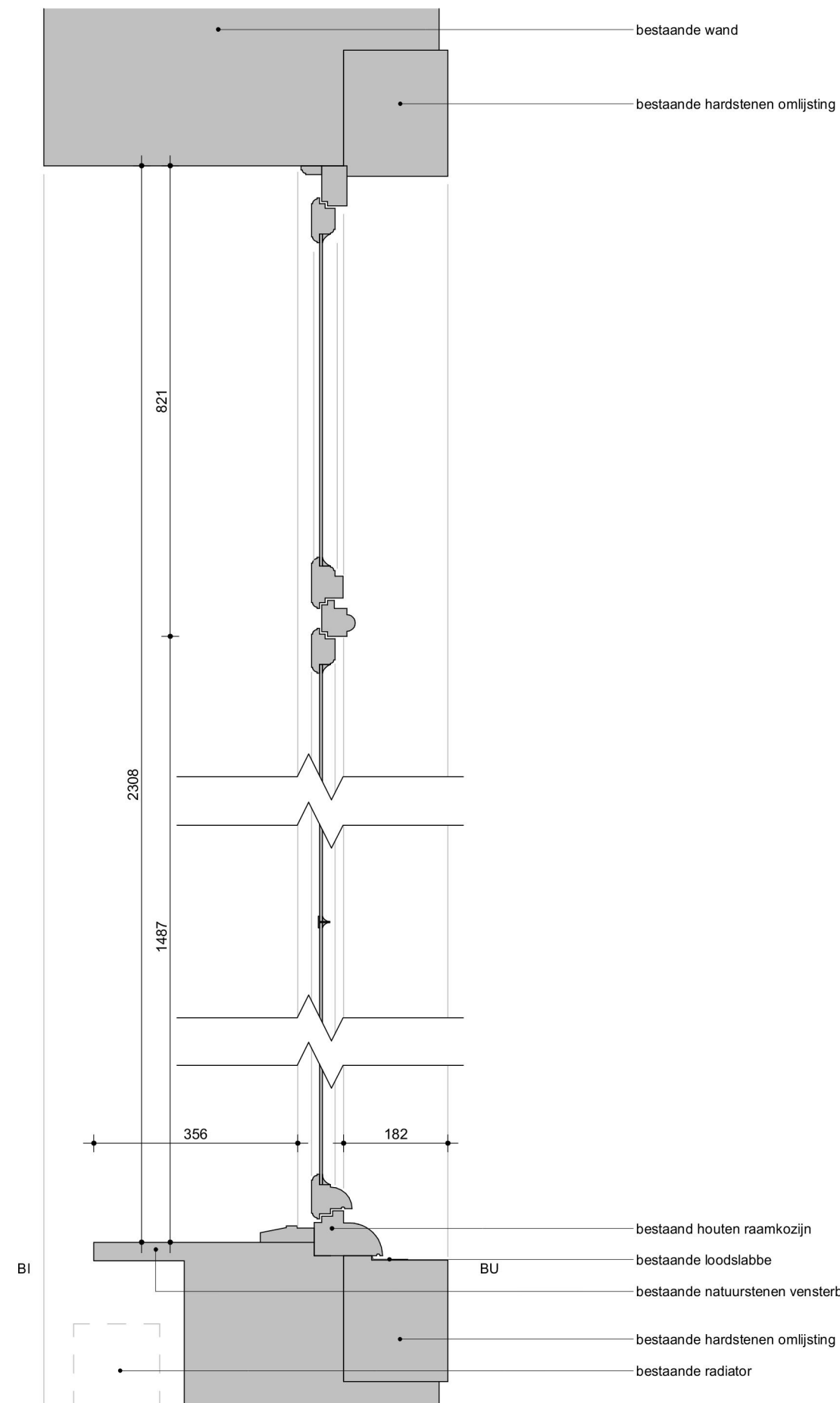
Merk 5A.02 - Bestaand detail B03-V
