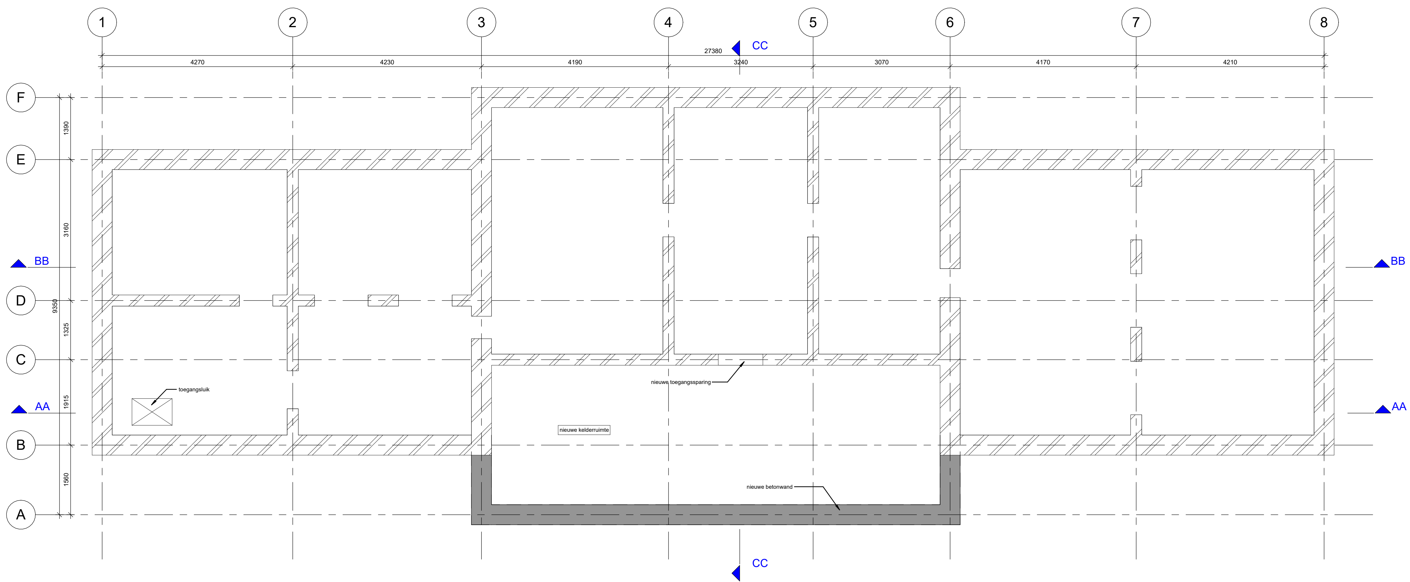
KELDER 1 : 50
