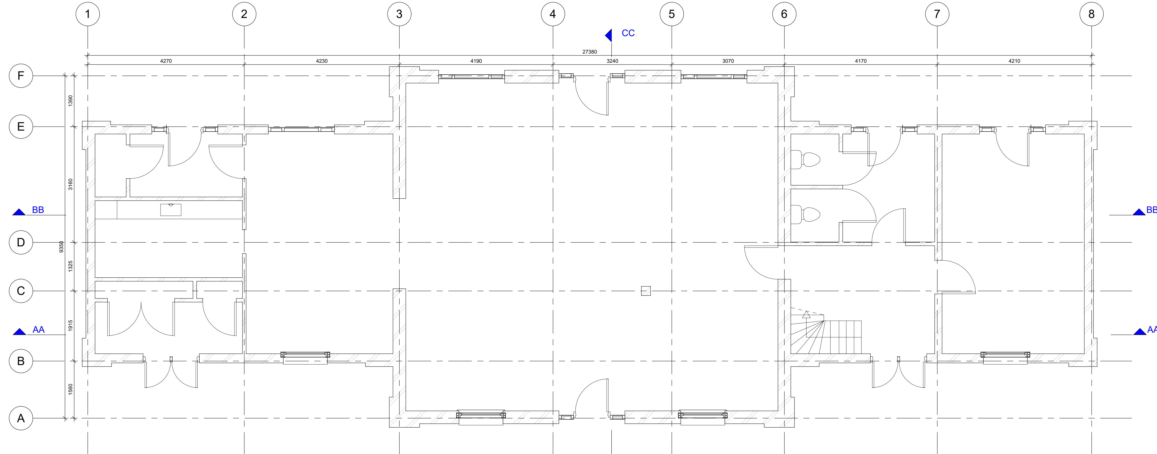
BEGANE GROND
