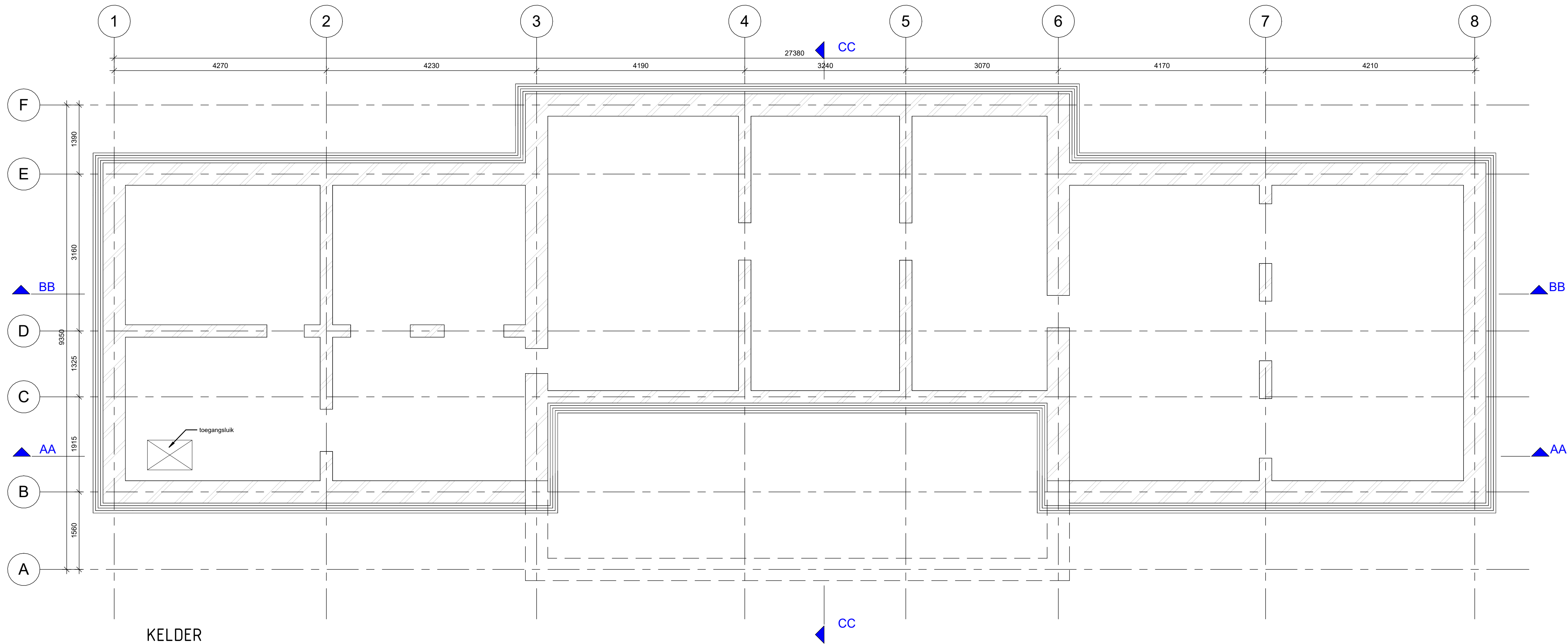
KELDER
