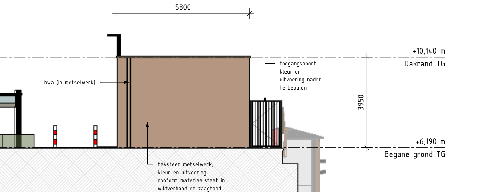
Techniekgebouw Noordgevel schaal: 1 : 100
