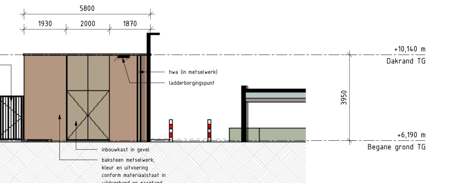
Techniekgebouw Zuidgevel schaal: 1 : 100
