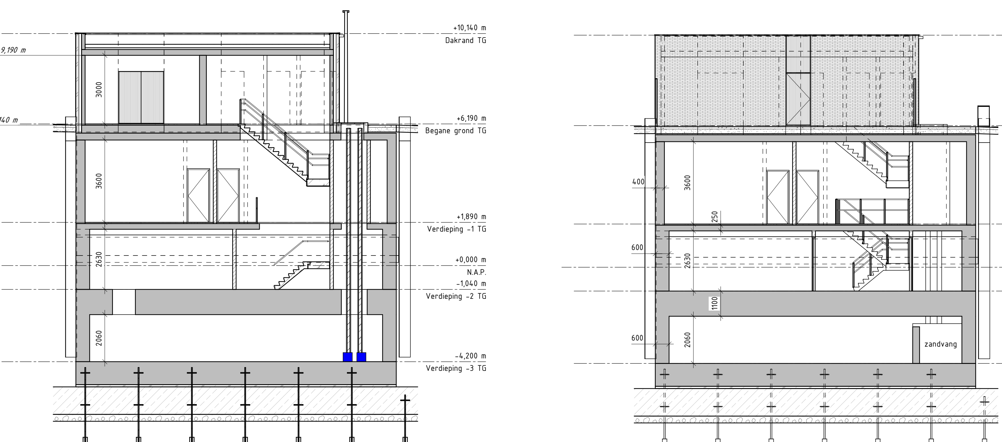
Doorsnede technische ruimte A-A V0 schaal: 1 : 100
