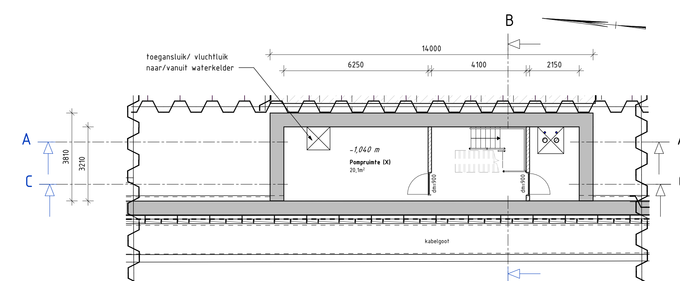
Verdieping -2 TG schaal: 1 : 100
