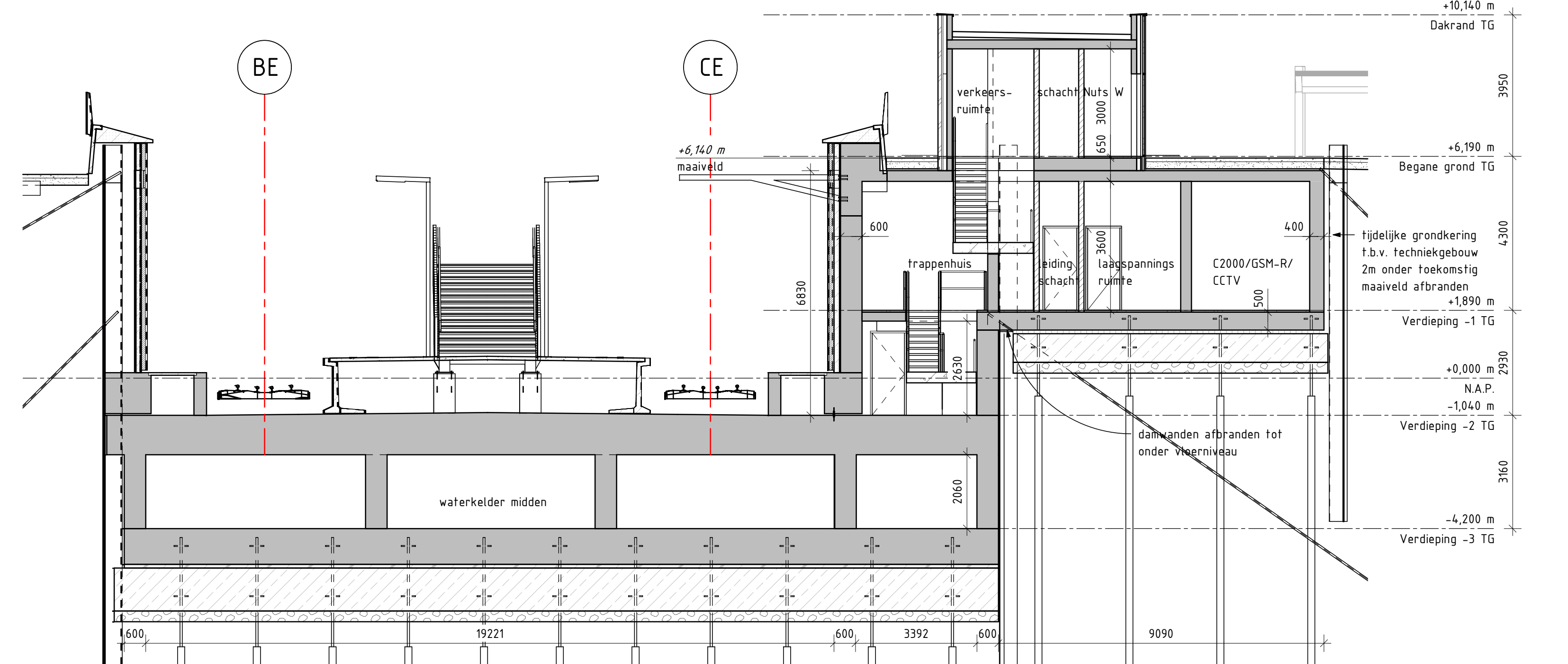
Doorsnede technische ruimte B-B V0 schaal: 1 : 100
