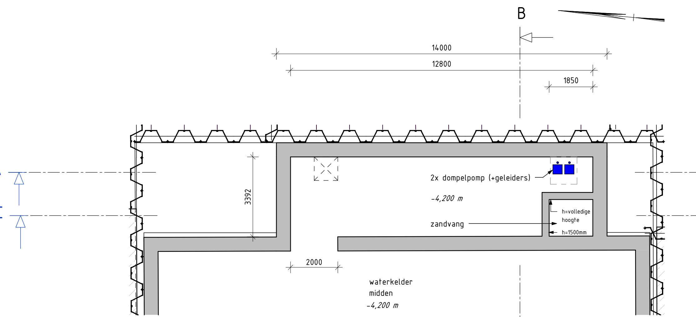
Verdieping -3 TG en waterkelder midden schaal: 1 : 100
