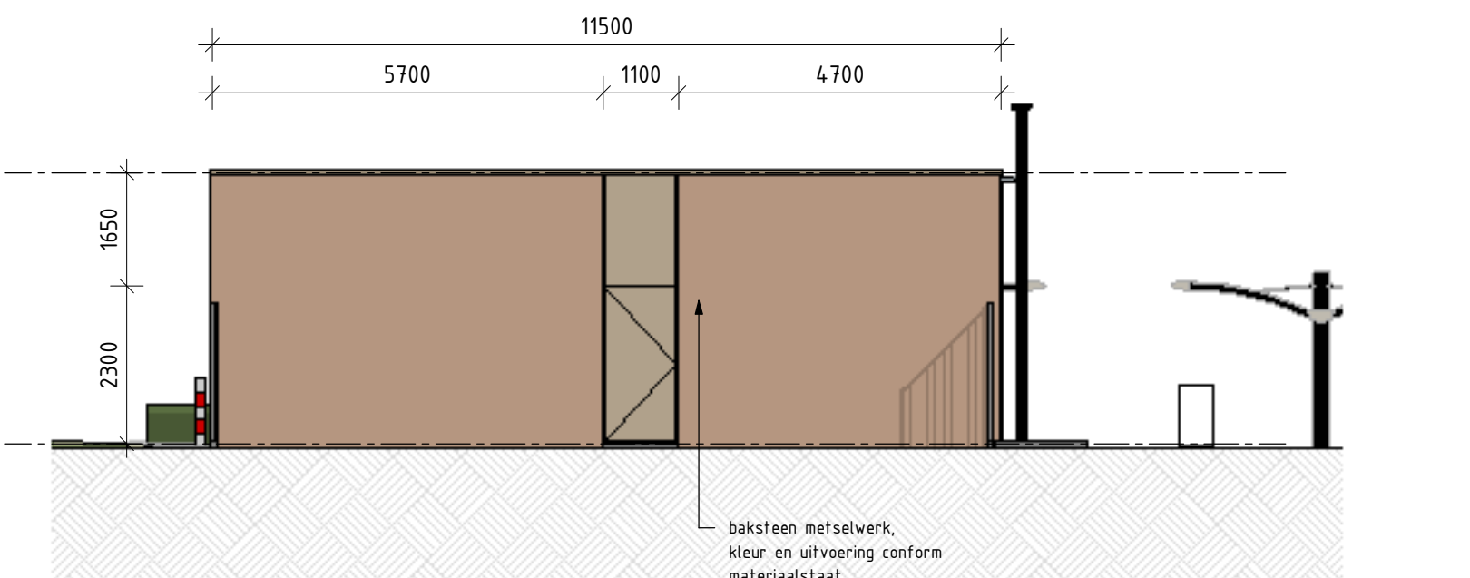
Techniekgebouw Westgevel schaal: 1 : 100
