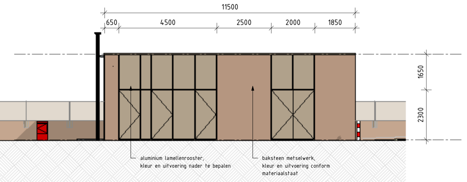
Techniekgebouw Oostgevel schaal: 1 : 100
