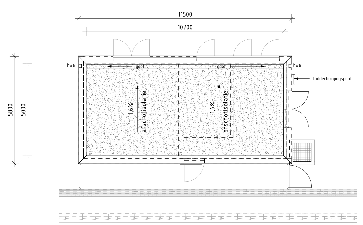
Dakrand TG schaal: 1 : 100
