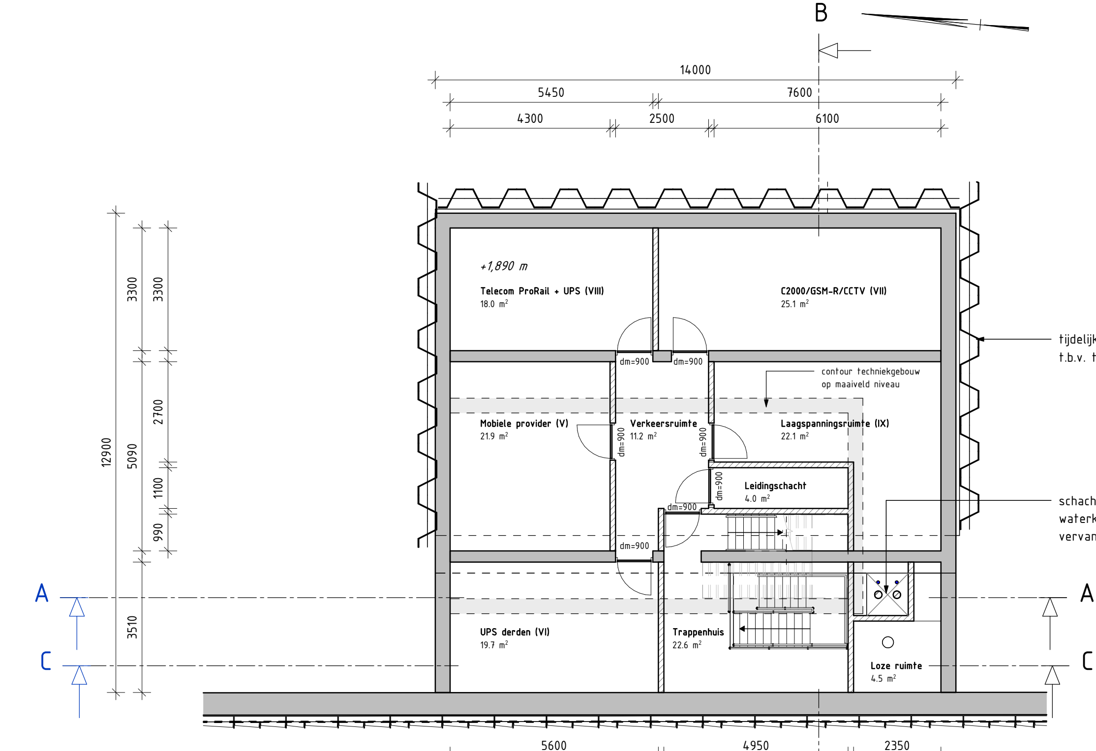
Verdieping -1 TG schaal: 1 : 100
