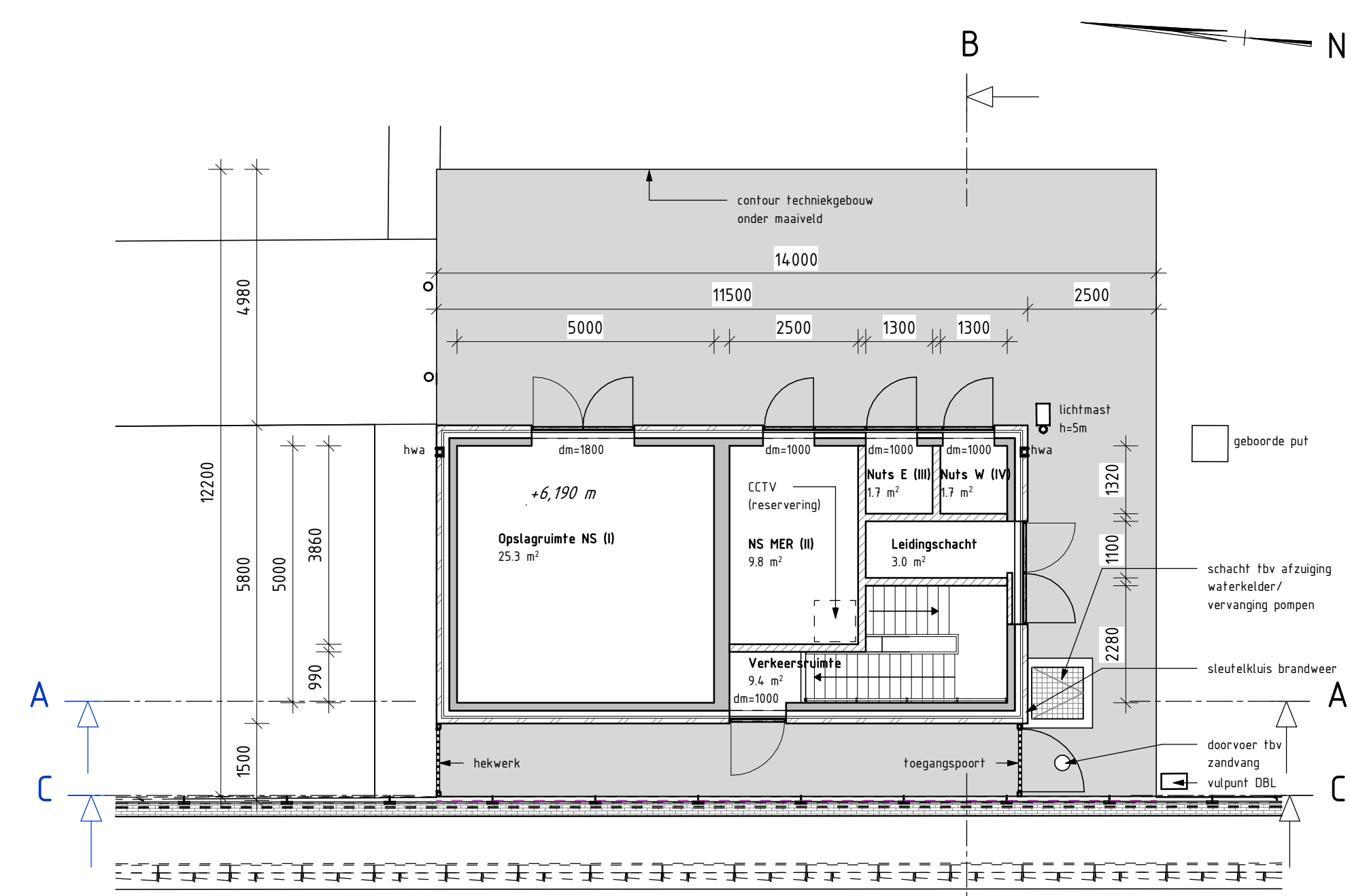
Begane grond TG schaal: 1 : 100
