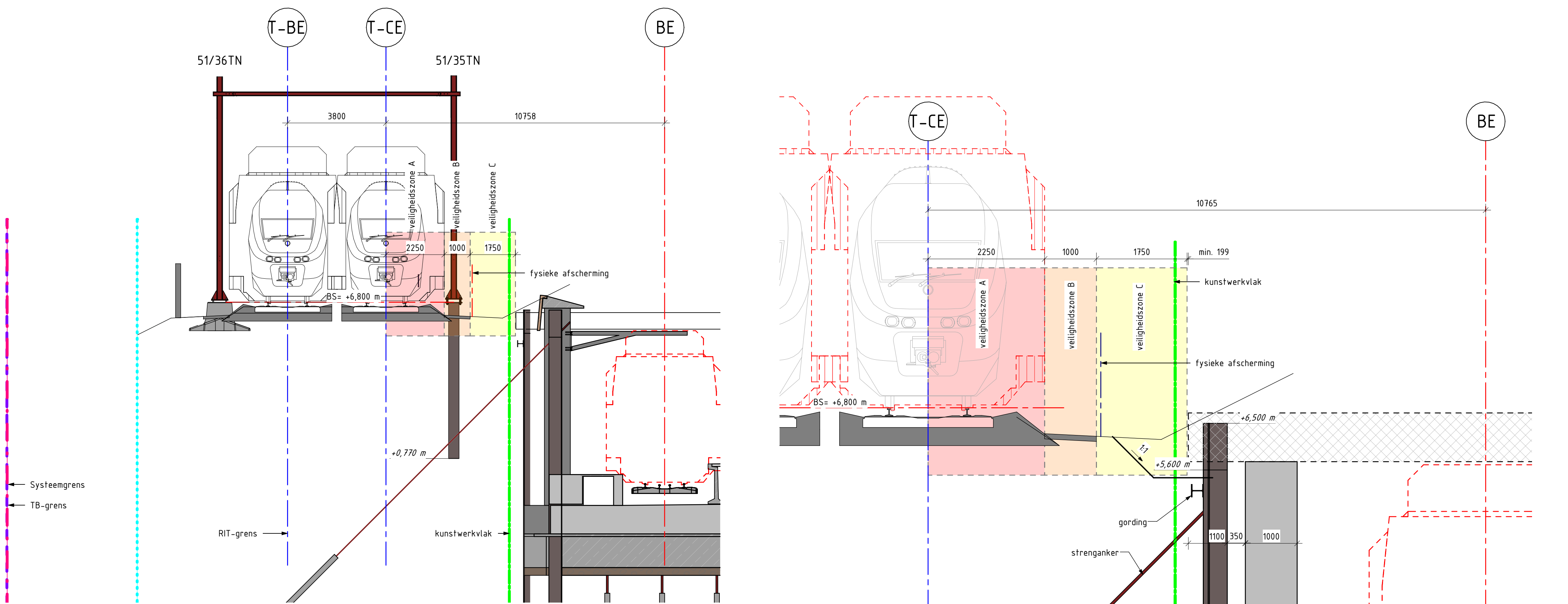
Doorsnede t.p.v. Bovenleidingsportaal C1
