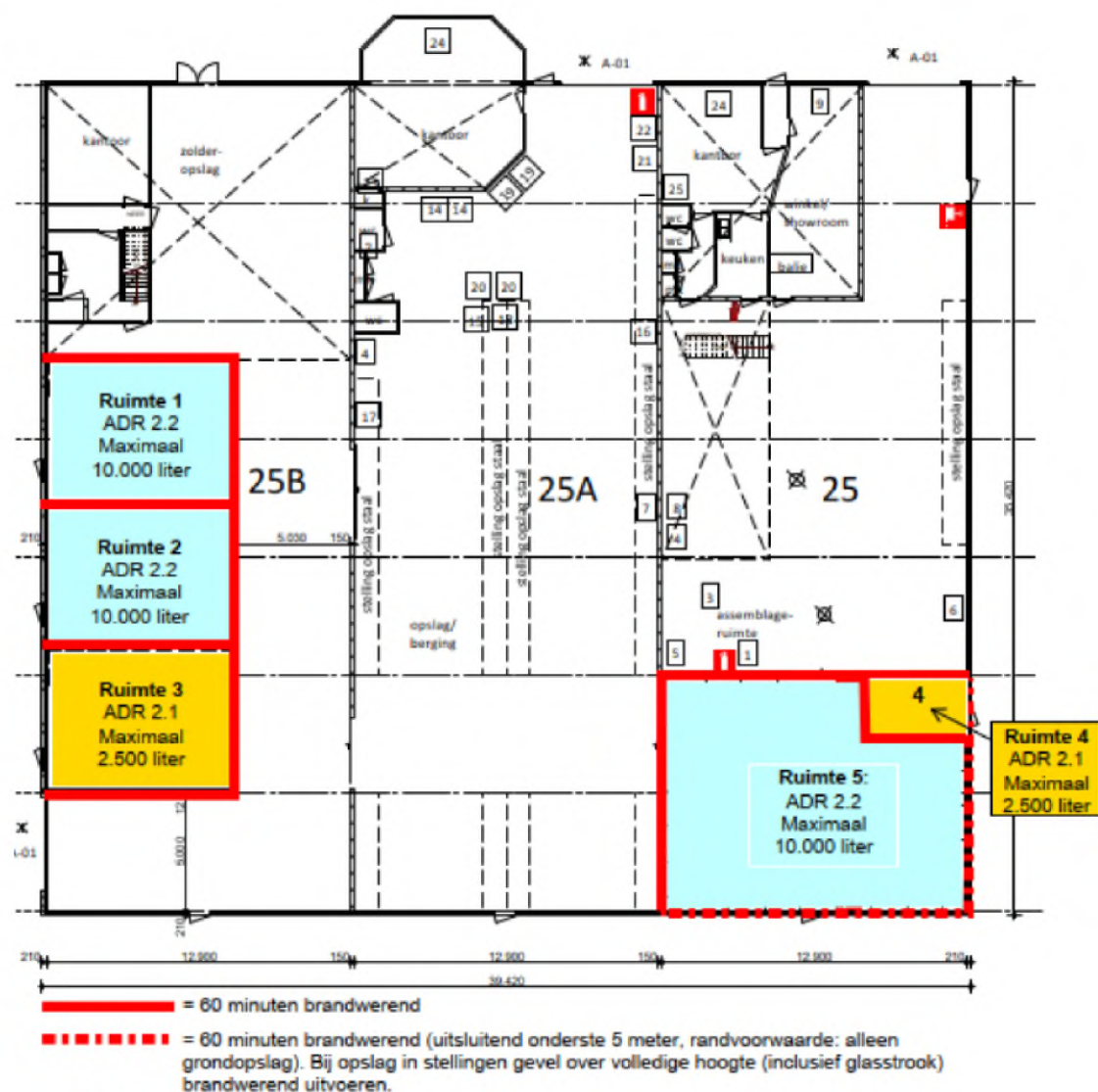
Figuur 1: indeling bedrijfshal
