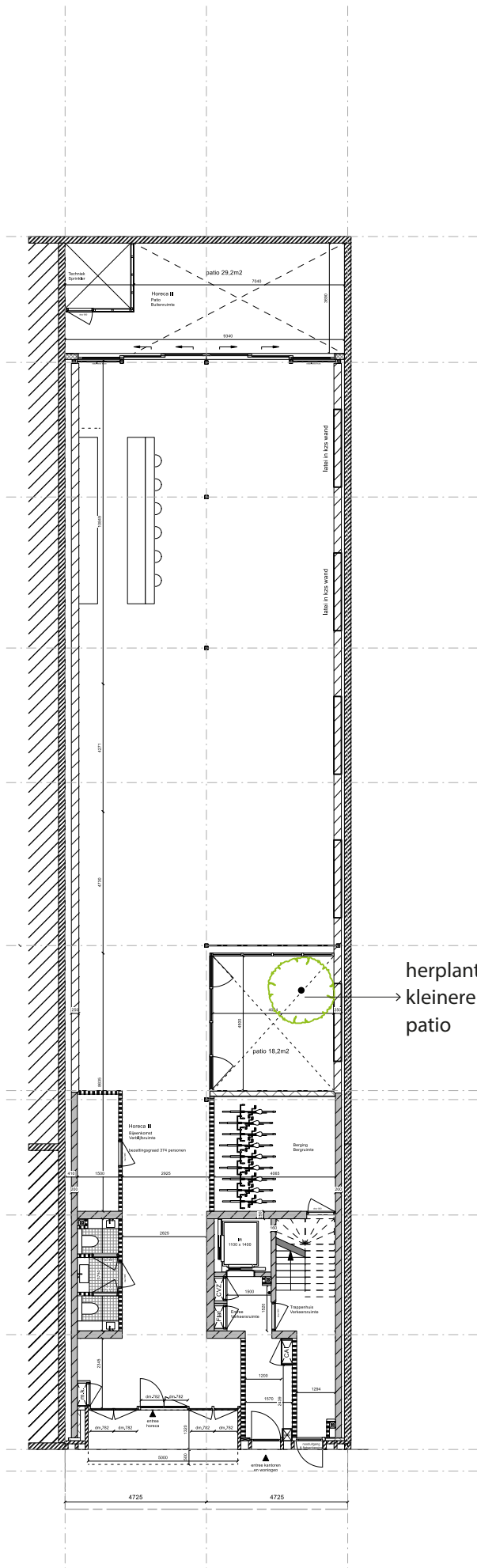
begane grond
