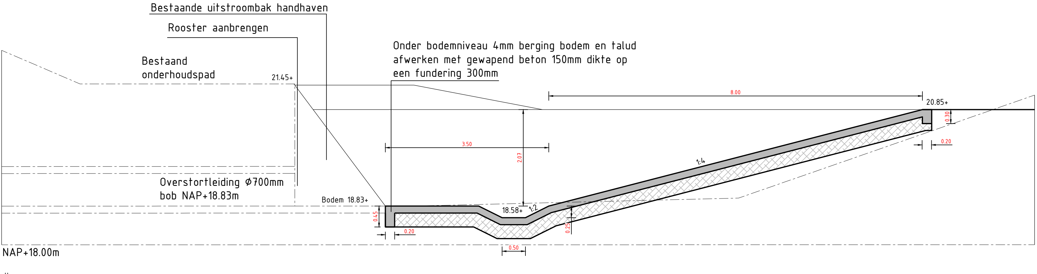
Detail uitstroombereiding overstort 2679: Dwarsdoorsnede Schaal 1:50
