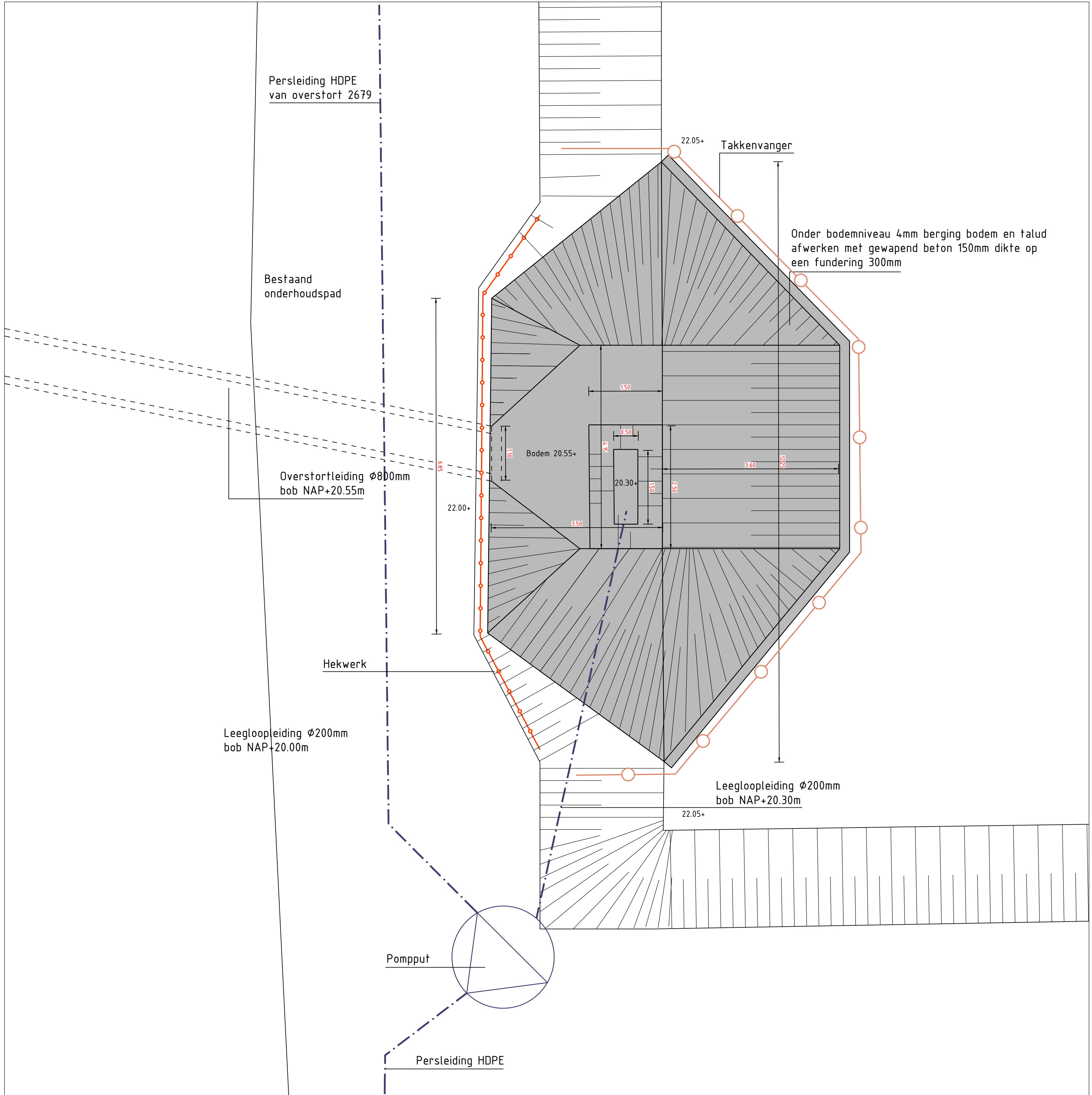
Detail uitstroombereiding overstort 2678: Situatie Schaal 1:50
