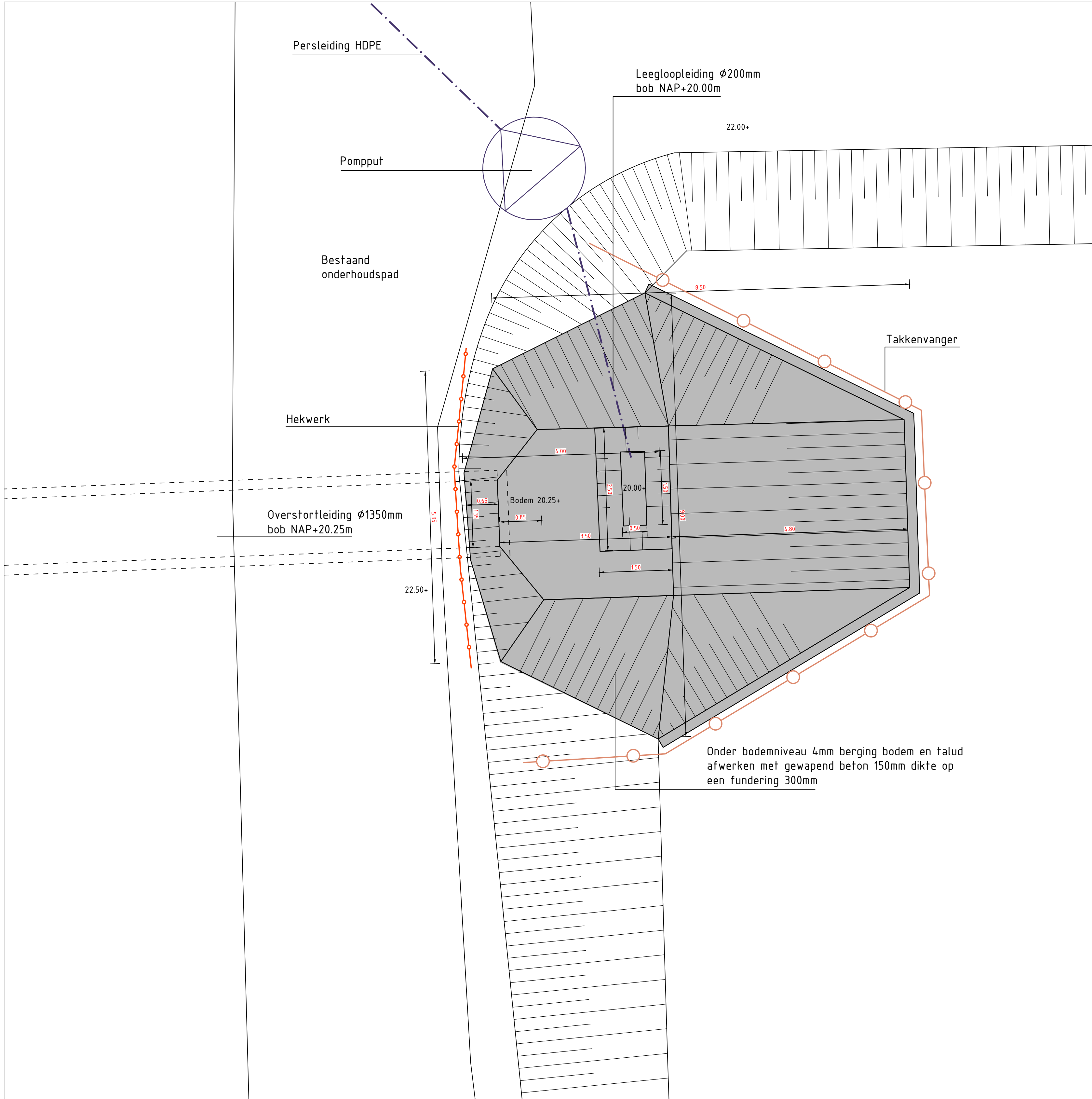
Detail uitstroombereiding overstort 3050: Situatie Schaal 1:50
