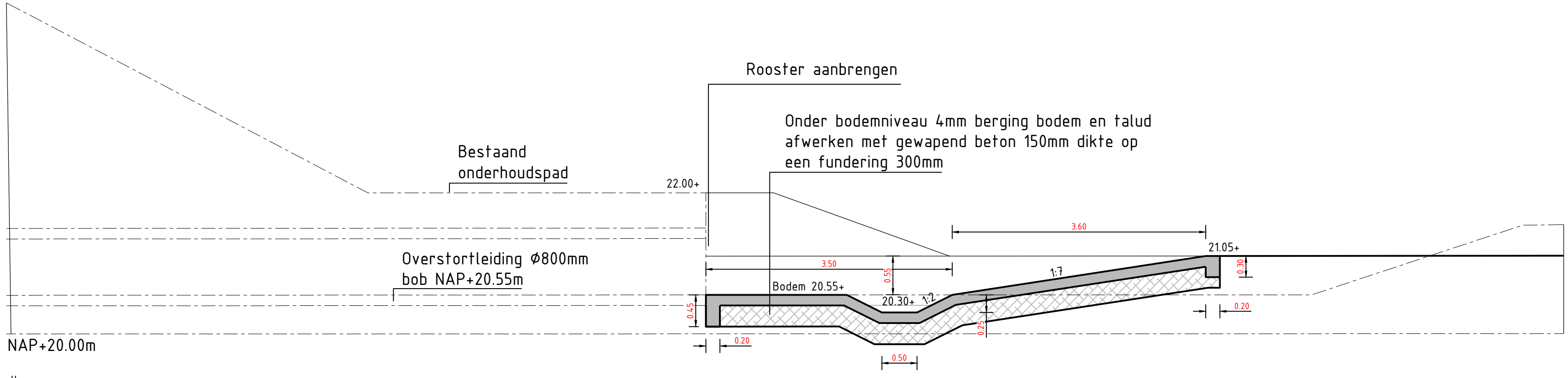
Detail uitstroombereiding overstort 2678: Dwarsdoorsnede Schaal 1:50
