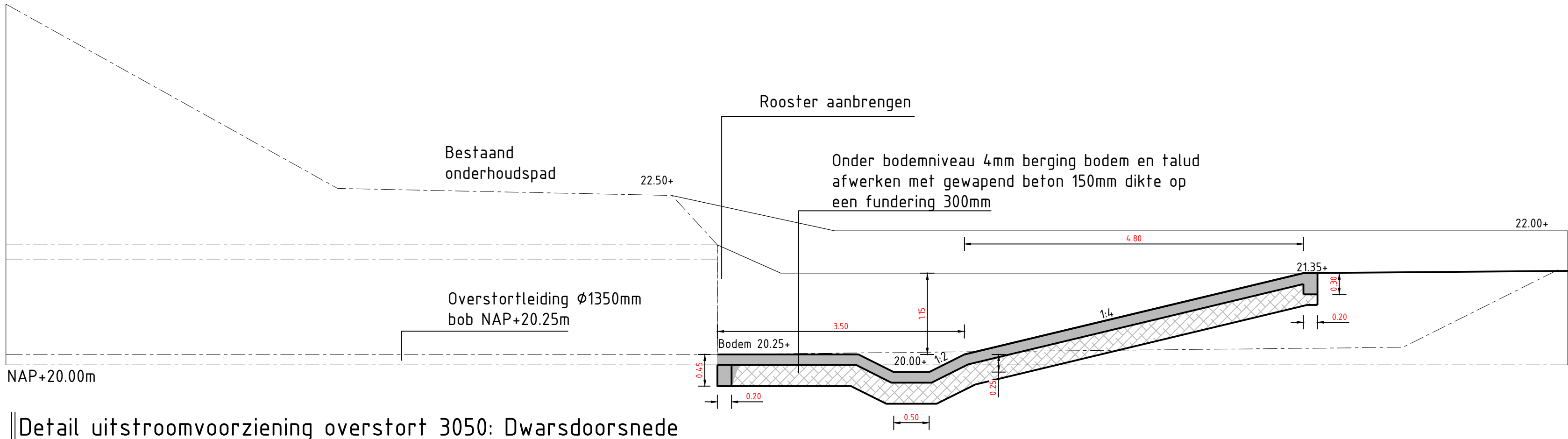
Detail uitstroombereiding overstort 3050: Dwarsdoorsnede Schaal 1:50
