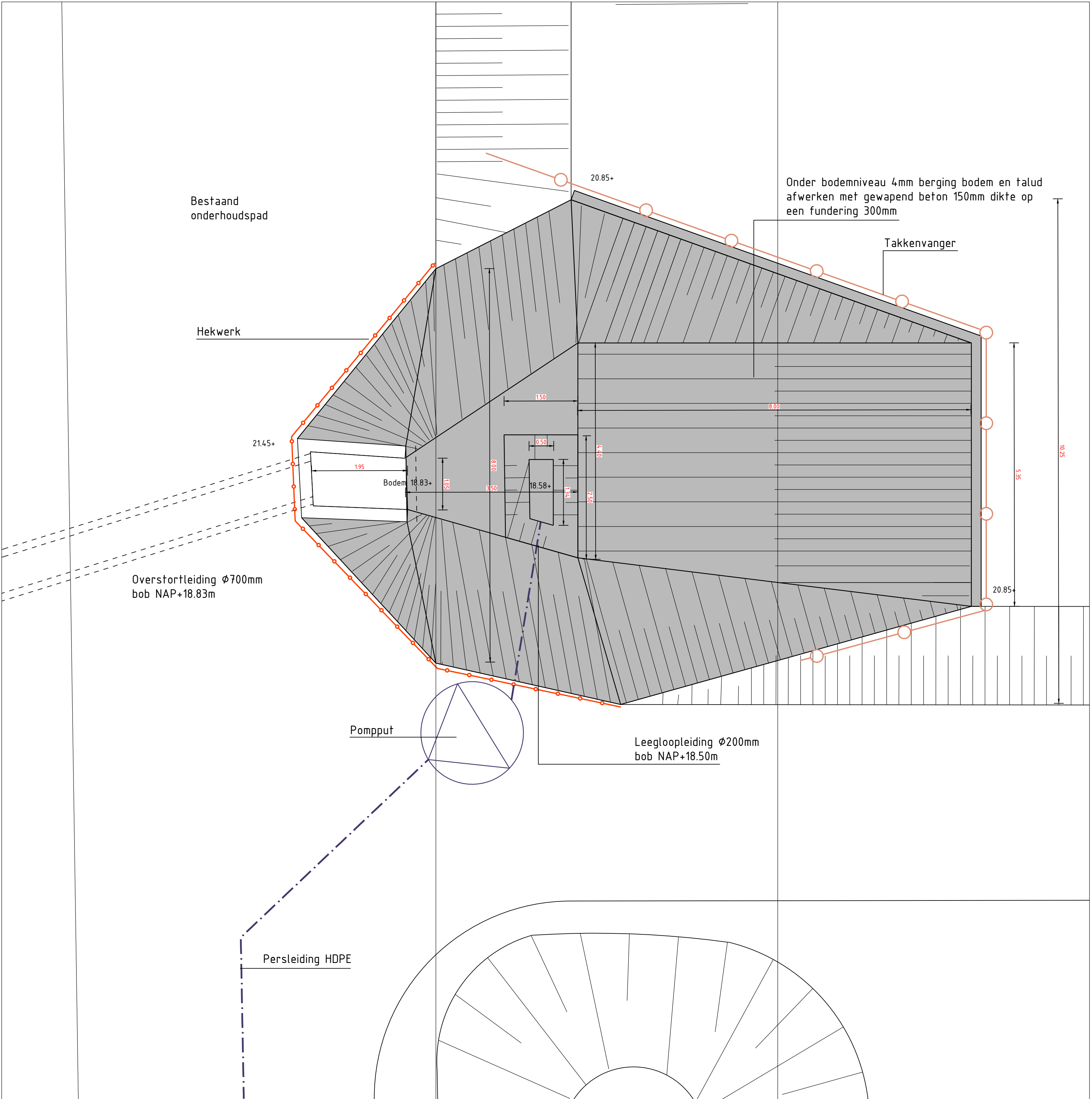
Detail uitstroombereiding overstort 2679: Situatie Schaal 1:50
