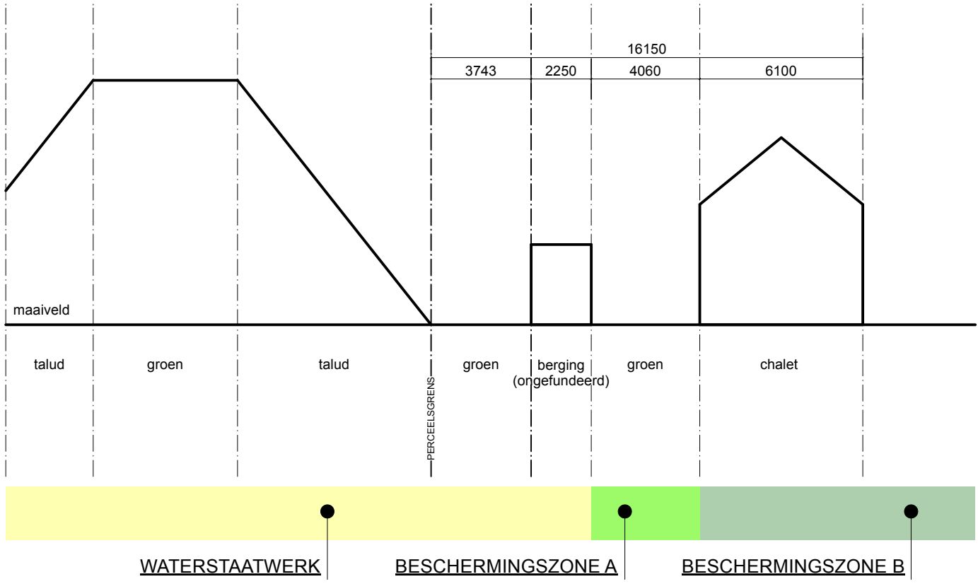
PROFIEL C* *maatvoering in millimeter
