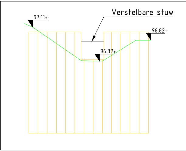
Profiel tpv stuw A-A' SCHAAL 1 : 50
