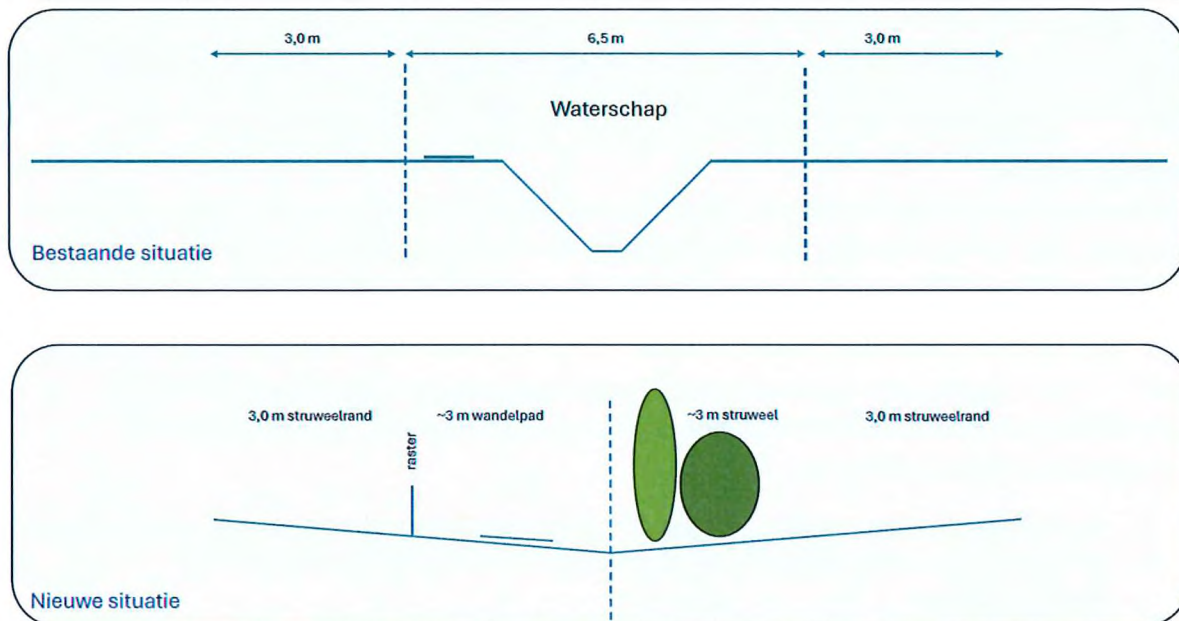
Fig 2: overzicht van bestaande en nieuwe situatie van de watergang GA78.
