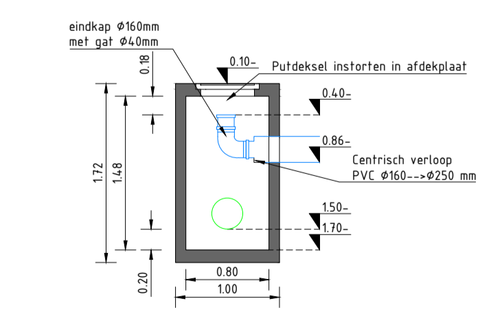
Detail 2 Knijpconstructie 1-1 SCHAAL 1 : 50
