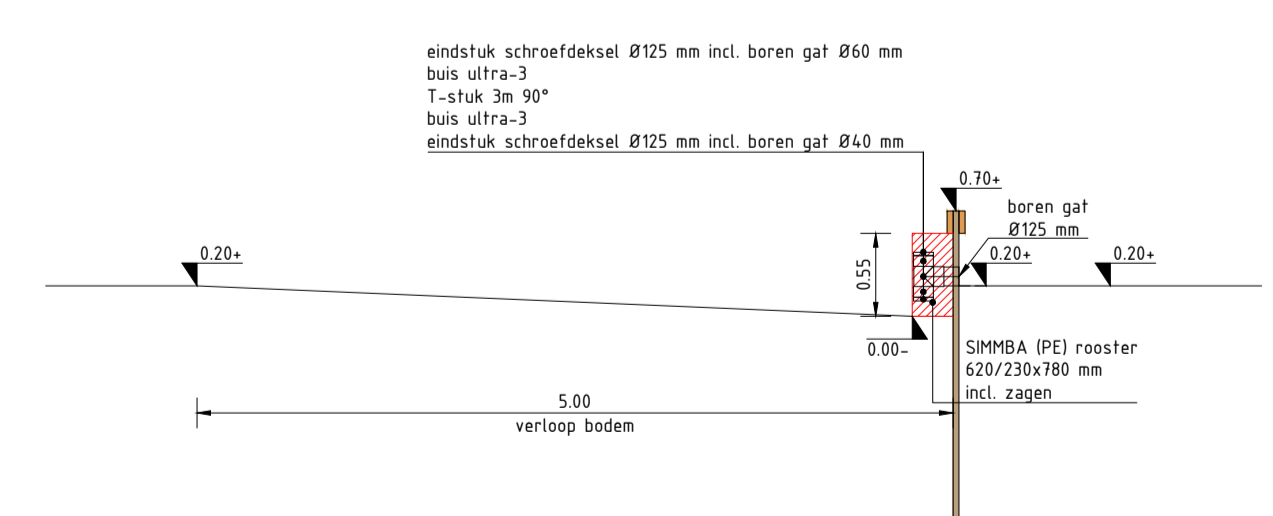
Detail 1 - Zijaanzicht Simmba stuw SCHAAL 1 : 50
