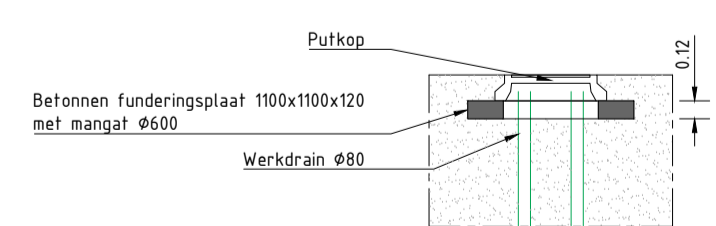
Detail 3 - Uittredepunt werkdrain SCHAAL 1 : 50
