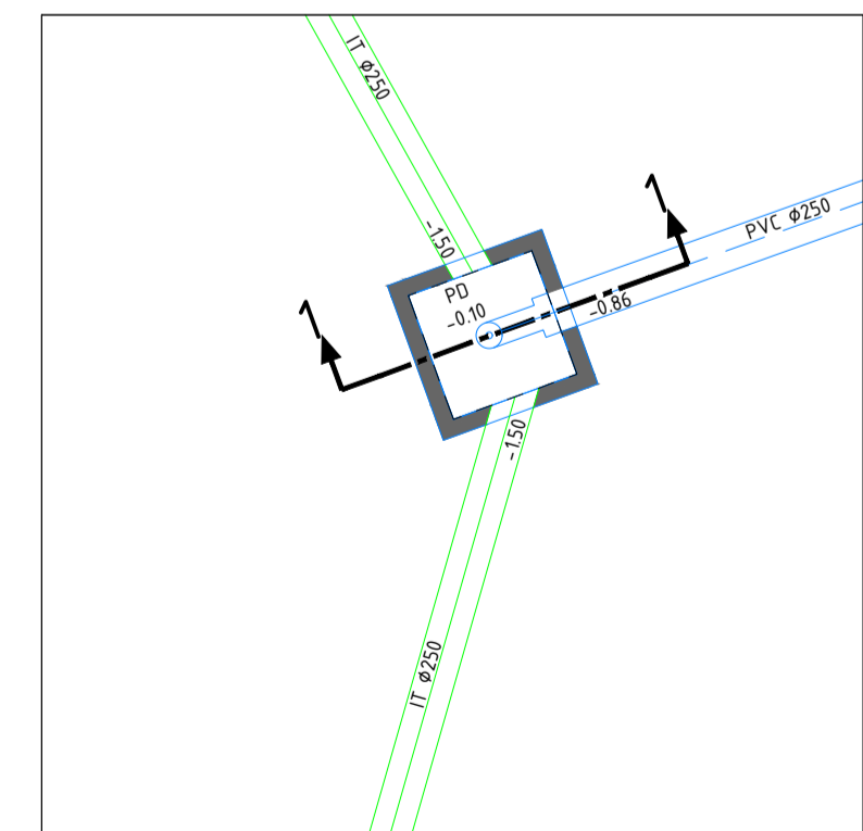
Detail 2 - Knijpconstructie SCHAAL 1 : 50
