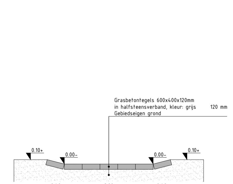
Doorsnede D-D SCHAAL 1 : 50
