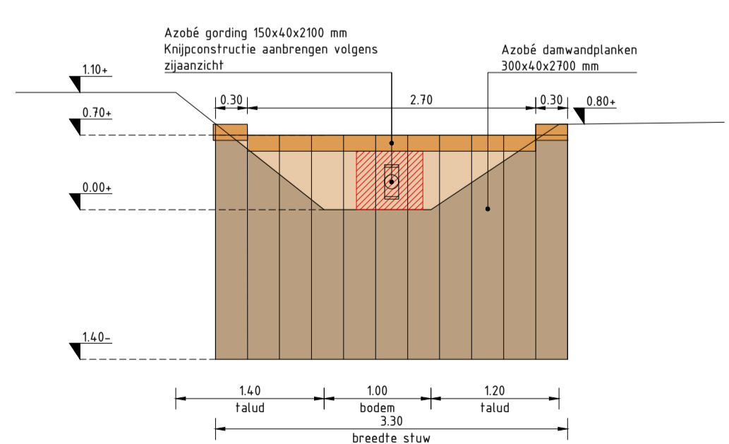
Detail 1 - Vooraanzicht Simmba stuw SCHAAL 1 : 50
