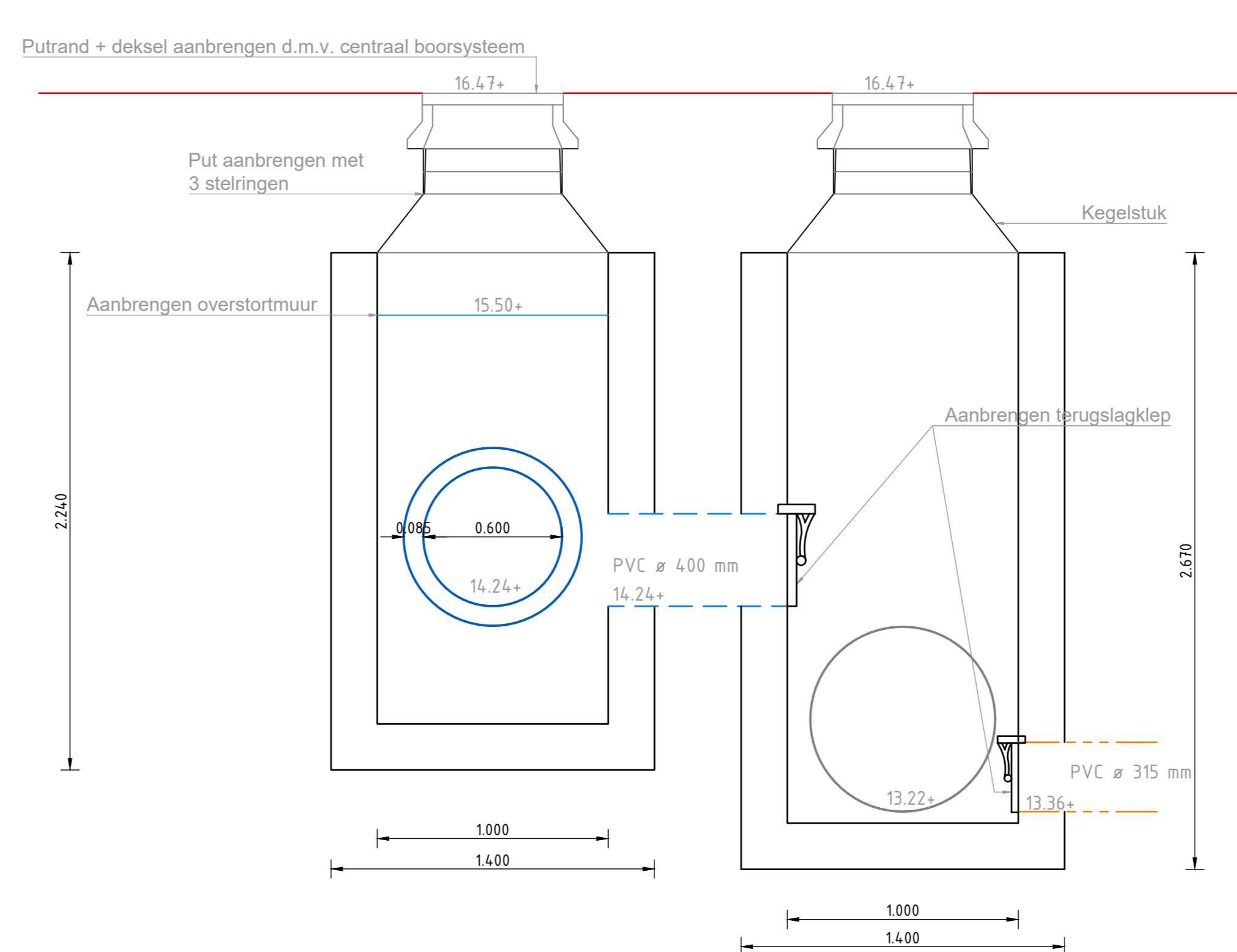
Detail 2 IT-overstortput R1 richting bestaand stelsel kruising Maasstraat-Derckxweg schaal 1:20
