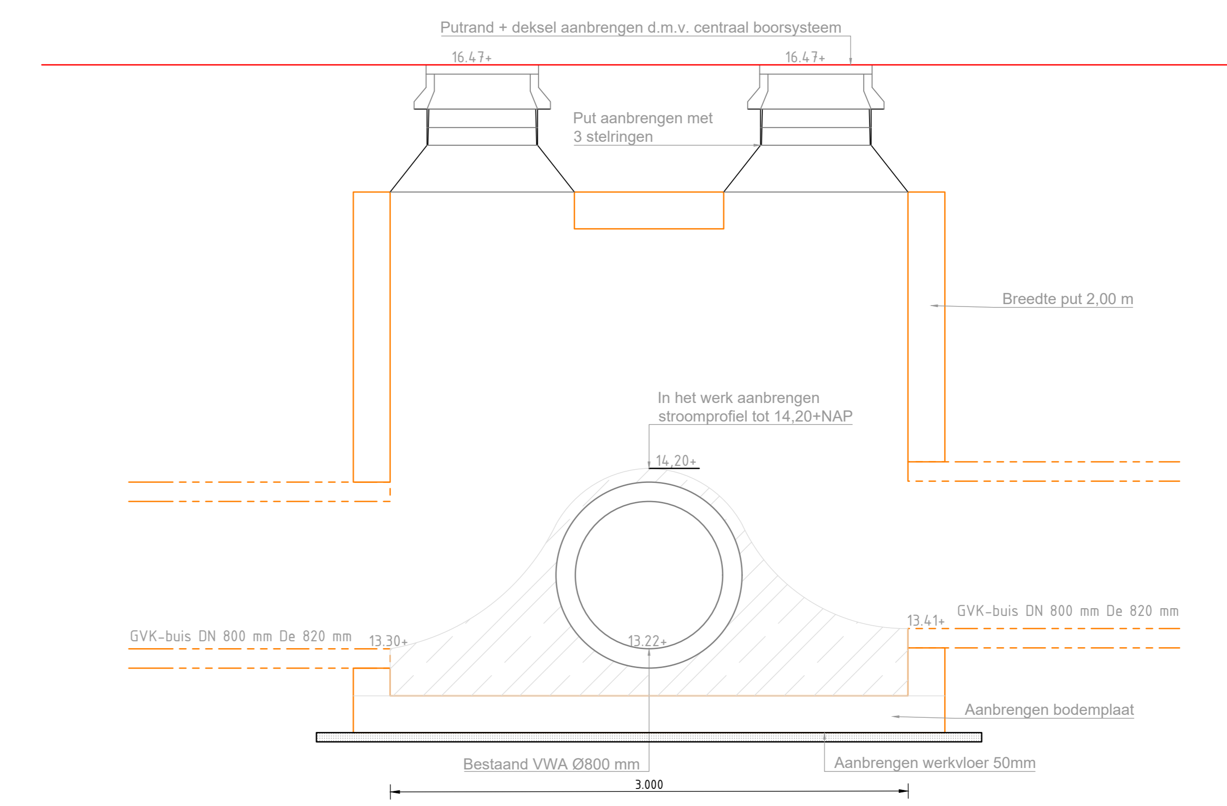
Detail 1 GWA-overstortput G3 richting BBB kruising Maasstraat-Derckxweg schaal 1:20
