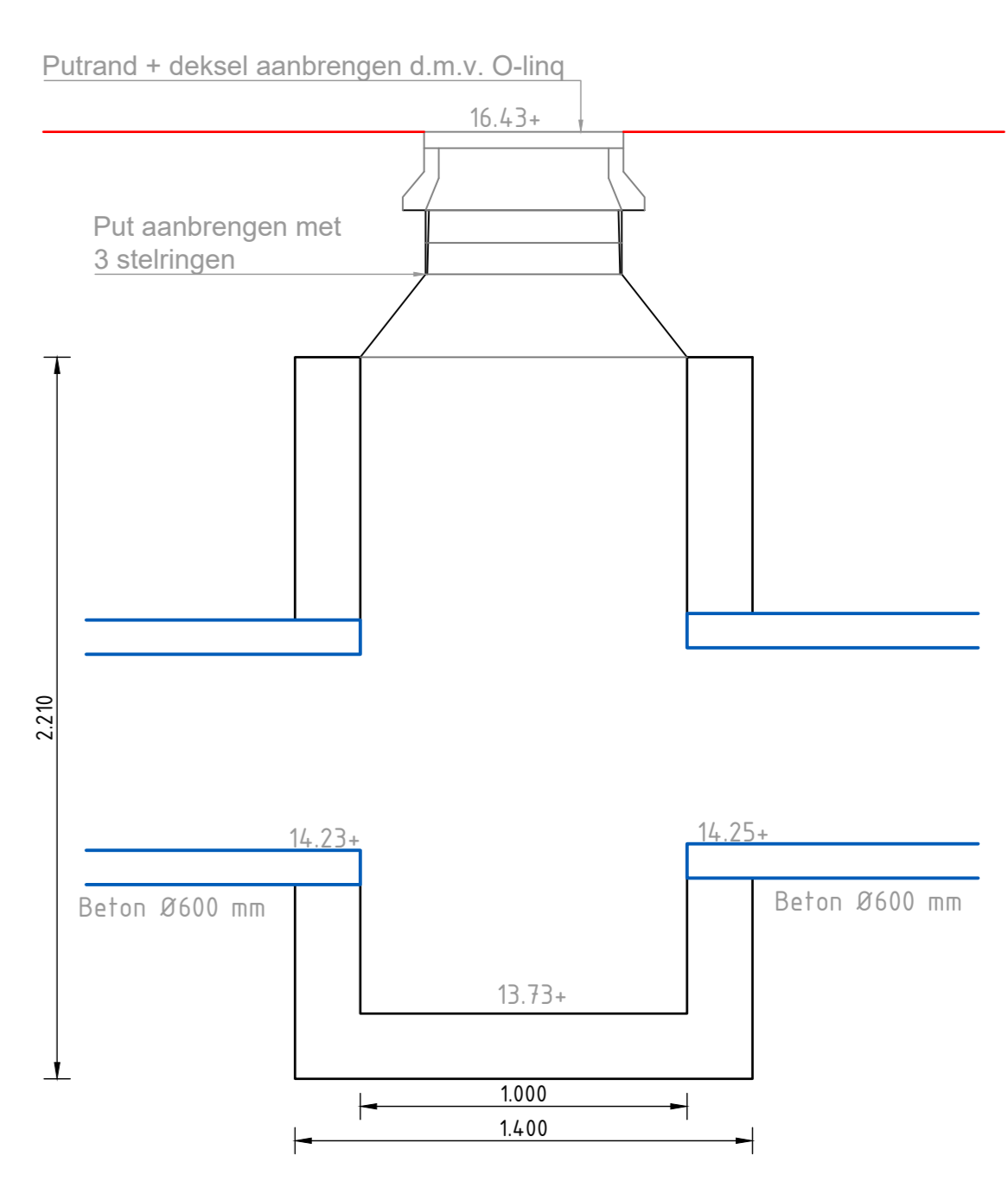
Detail 3 IT-inspectieput R2 algemeen detail schaal 1:20
