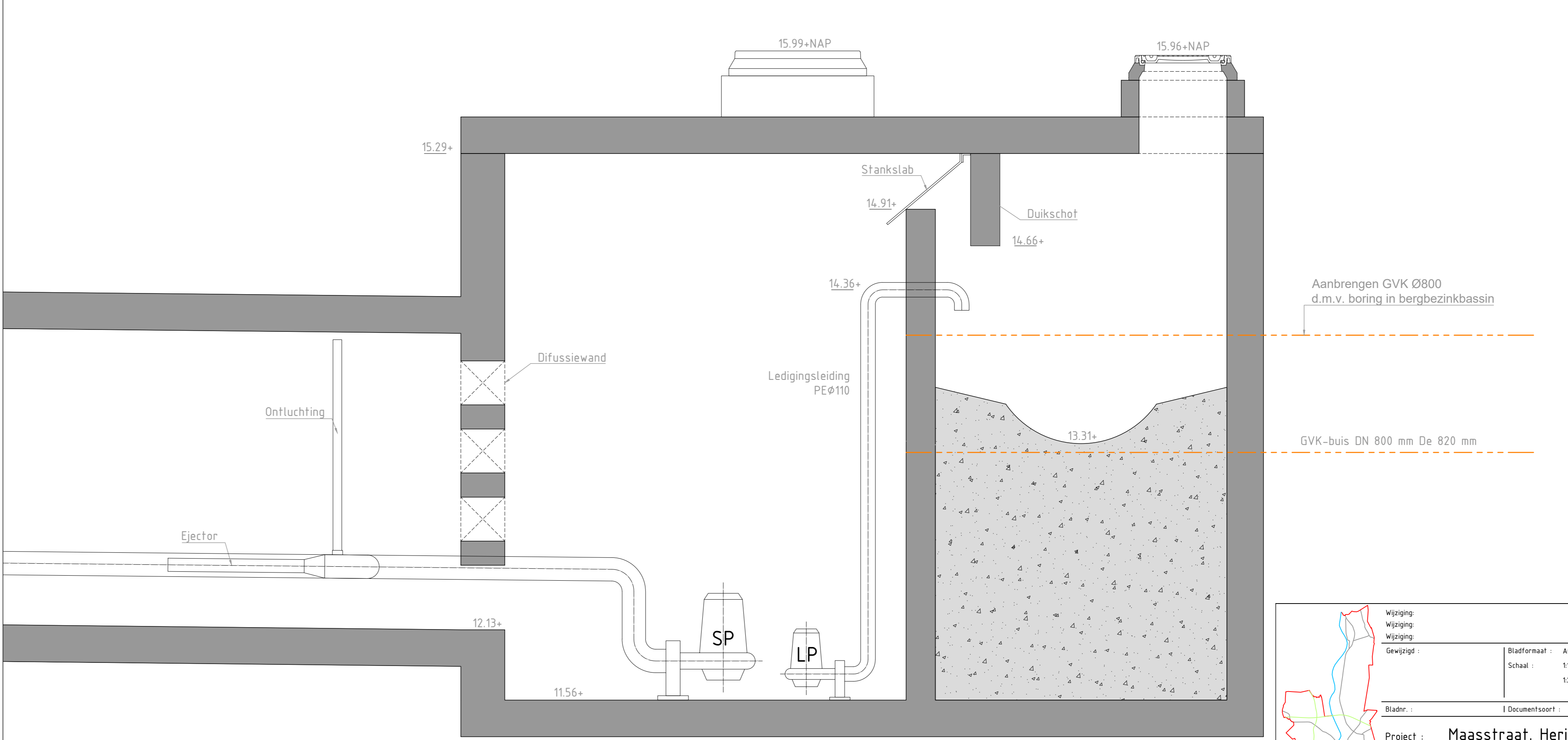
Detail 4 Aanbrengen GVK-buis DN800 De 820 mm in bestaande bergbezinkbassin d.m.v. boring schaal 1:20
