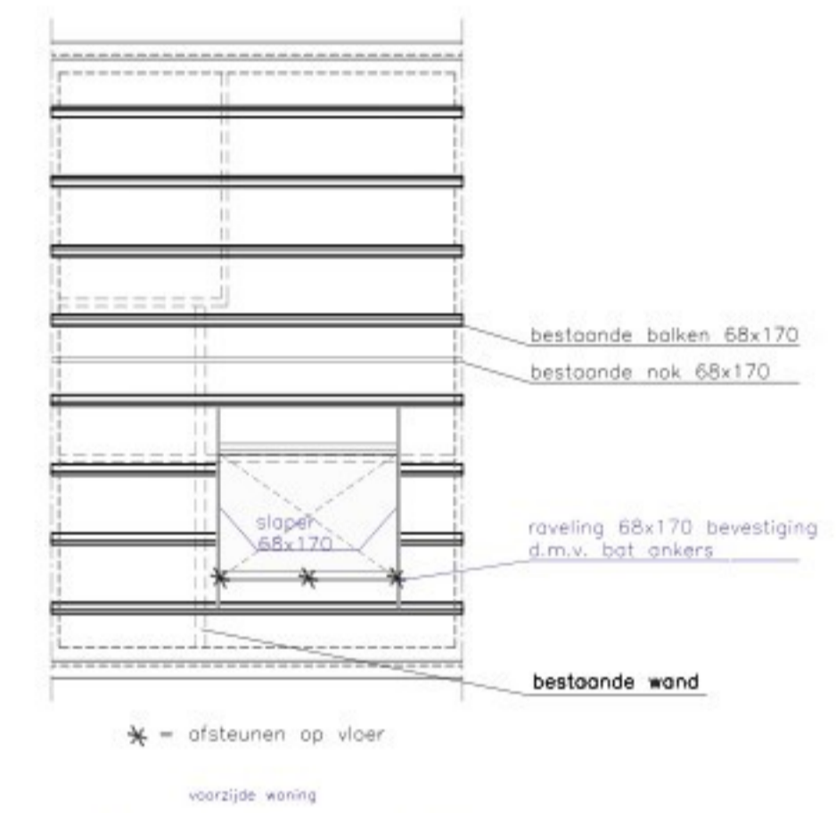
KAPPLAN NIEUW
