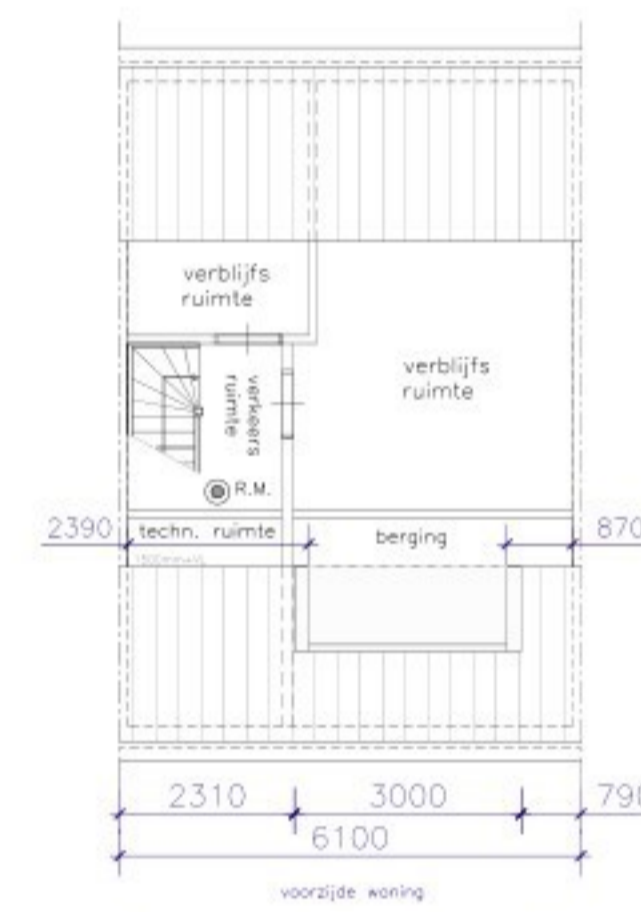
INDELING NIEUW
