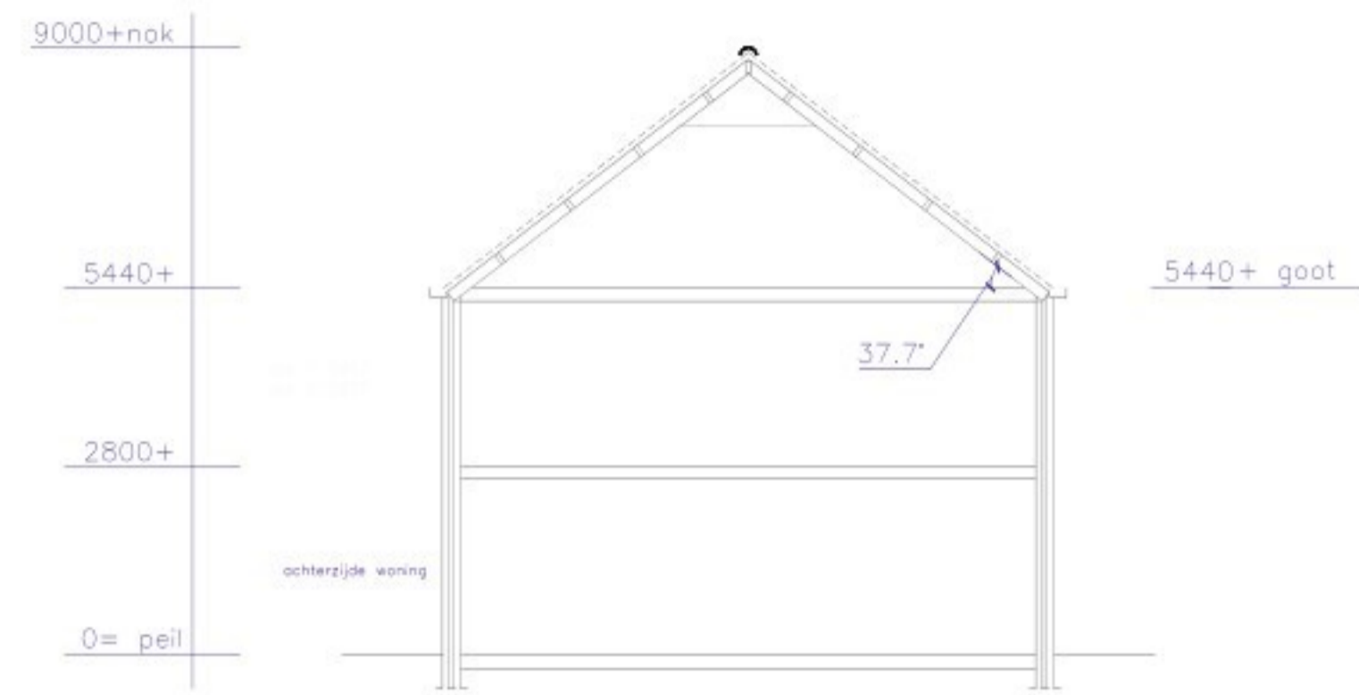
DOORSNEDE BESTAAND
