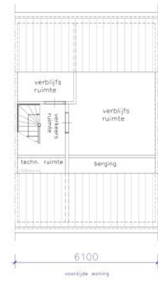
INDELING BESTAAND
