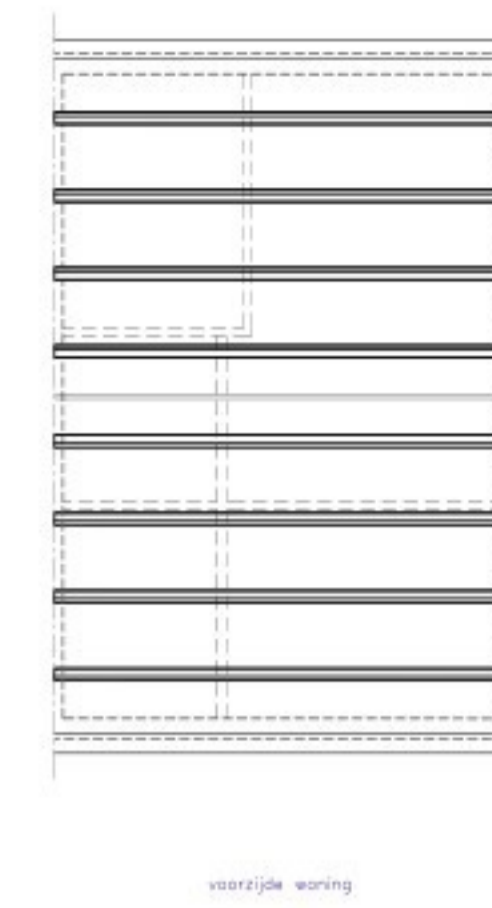
KAPPLAN BESTAAND
