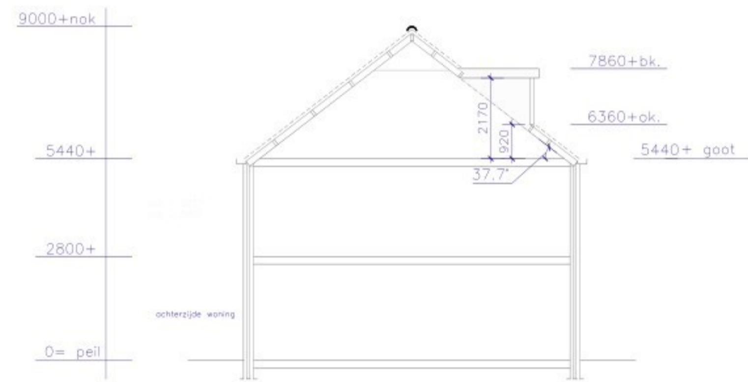
DOORSNEDE NIEUW
