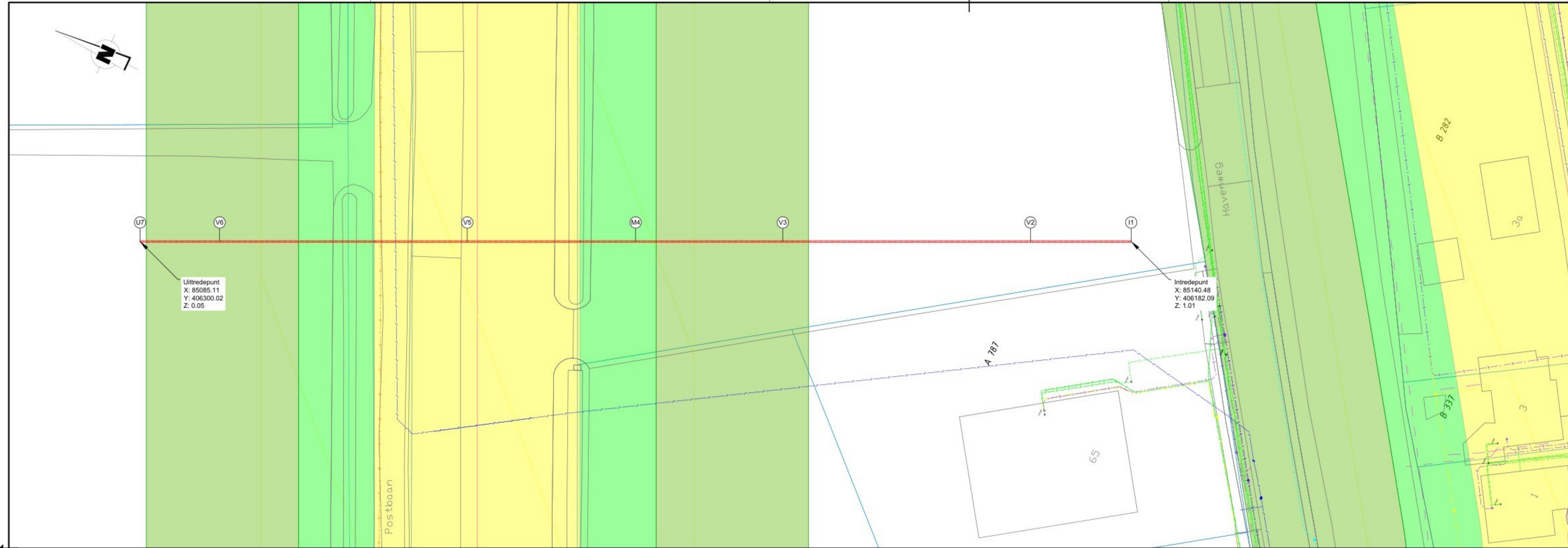
OVERZICHT SCHAAAL 1: 250
